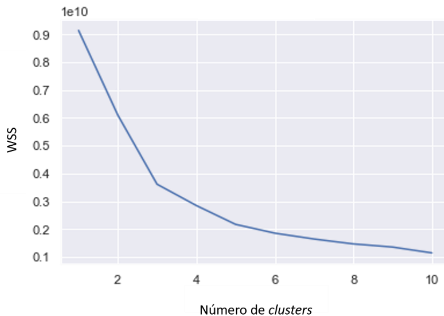
Figura 11 - Método do Cotovelo
