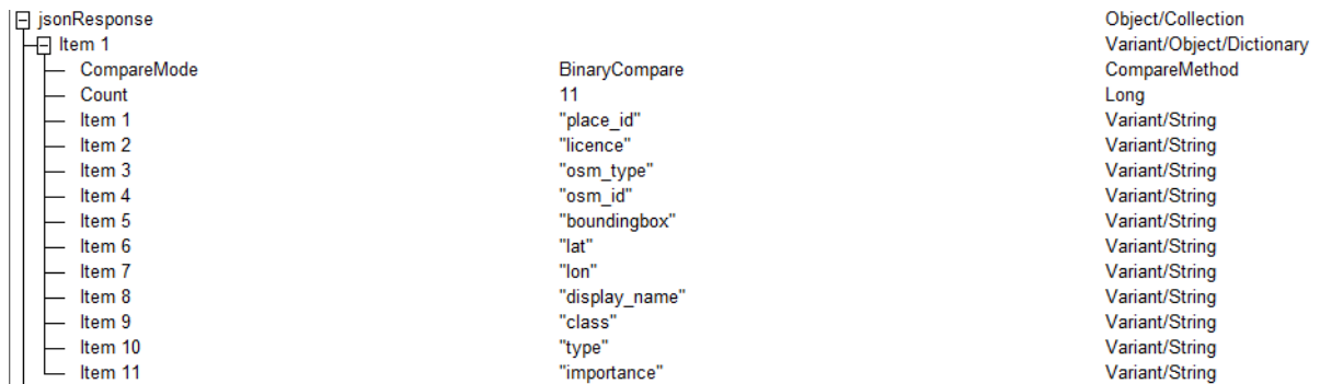
Figura 2: Exemplo de JSON convertido em dicionário - resposta Geocoding API
