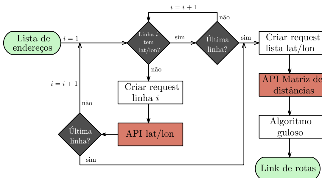
Figura 3: Funcionamento dos módulos
