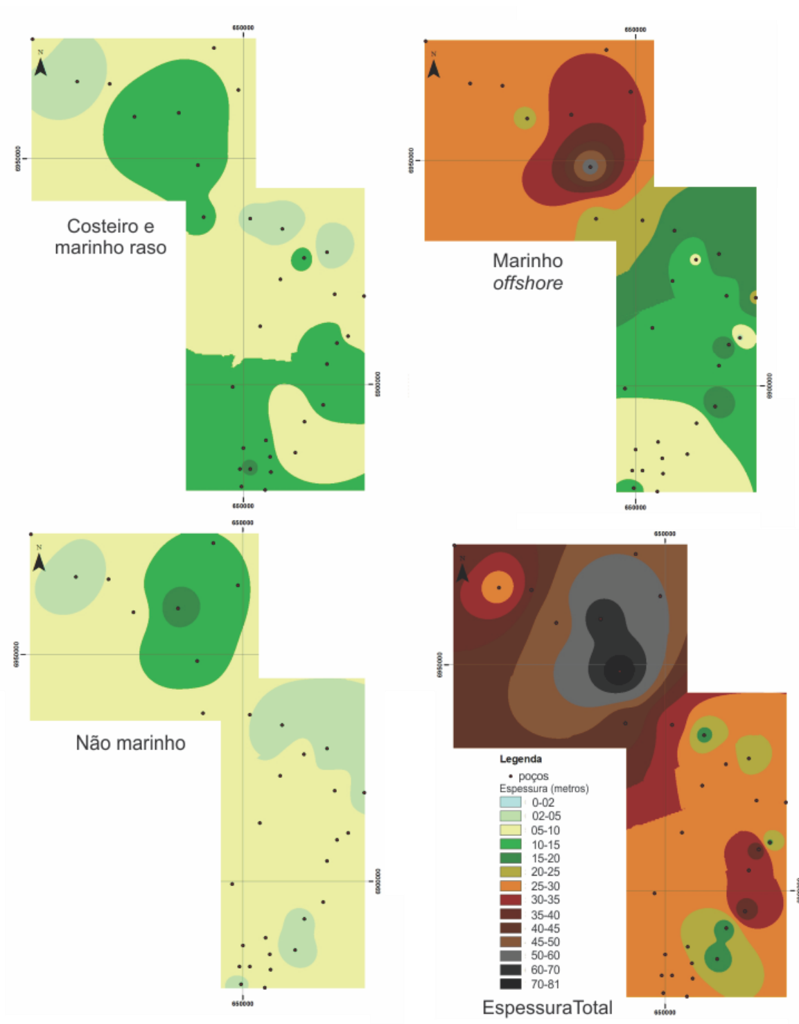
FIGURA 19: MAPA DE ISÓPACAS DA SEQUÊNCIA 2 INCLUINDO ESPESSURA TOTAL E ESPESSURA DAS ASSOCIAÇÕES A, B e C.
