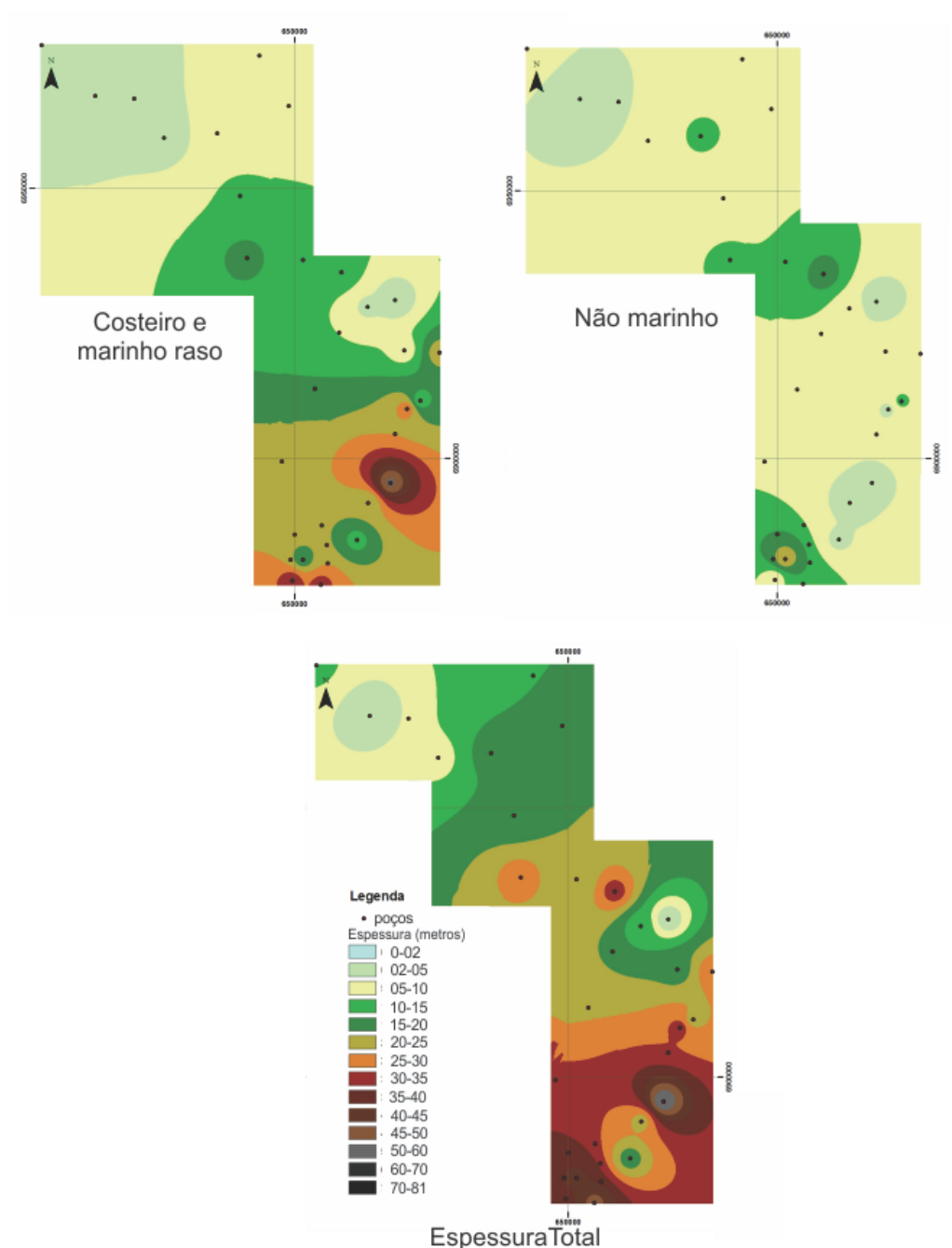
FIGURA 18: MAPA DE ISÓPACAS DA SEQUÊNCIA 1 INCLUINDO ESPESSURA TOTAL E ESPESSURA DAS ASSOCIAÇÕES A E B.
