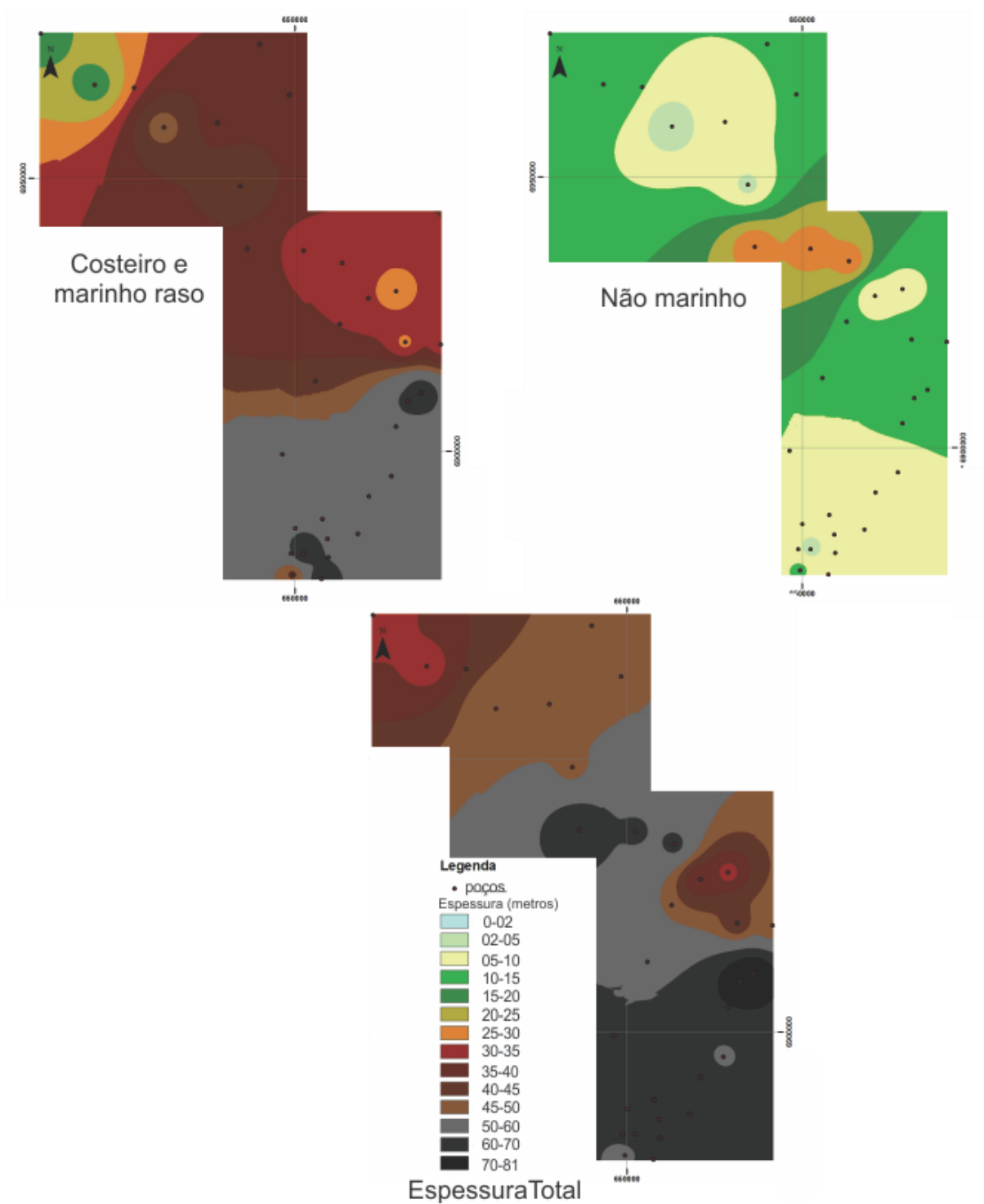
FIGURA 20: MAPA DE ISÓPACAS DA SEQUÊNCIA 3 INCLUINDO ESPESSURA TOTAL E ESPESSURA DAS ASSOCIAÇÕES A E B.
