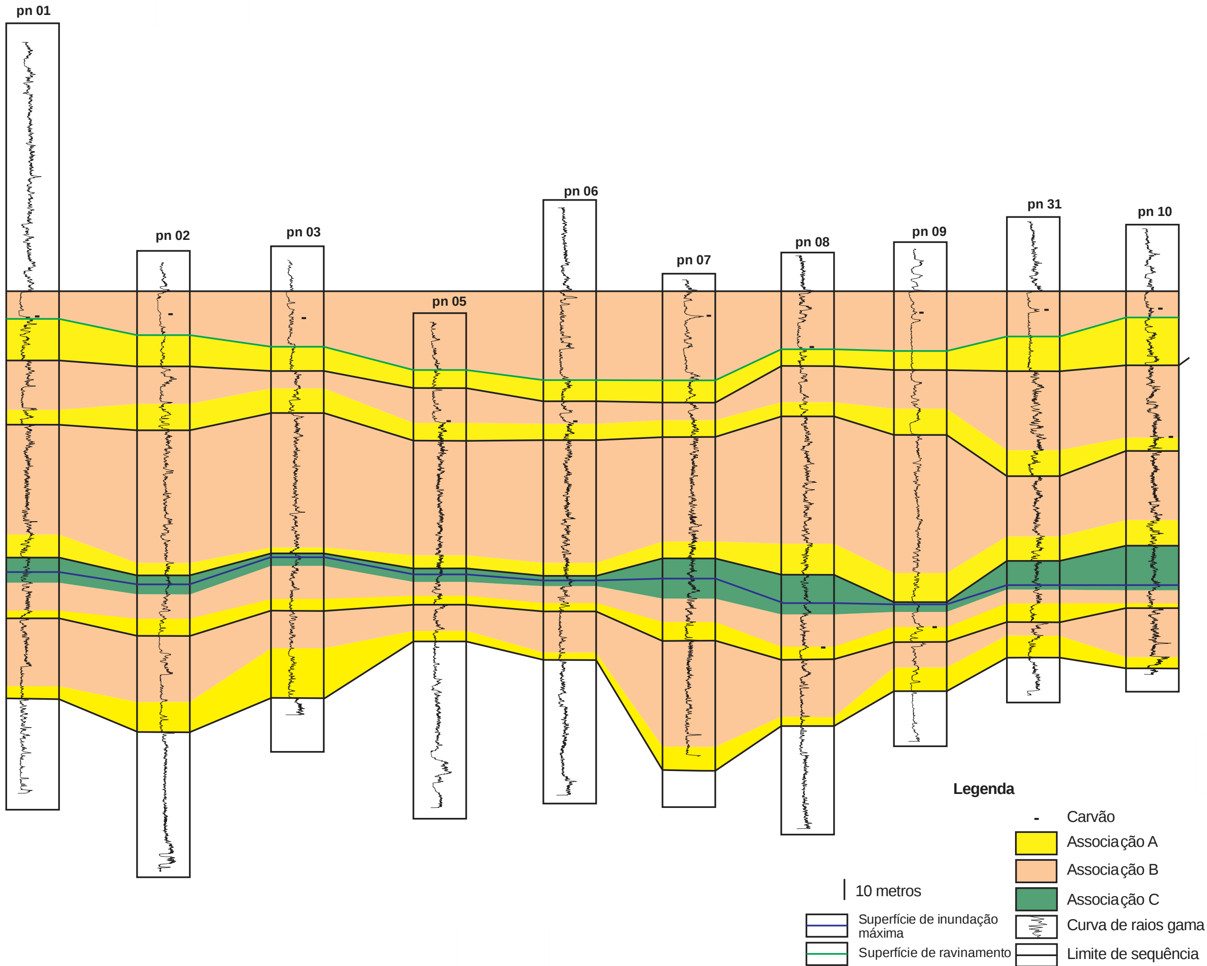
FIGURA 16: SEÇÃO B COM ASSOCIAÇÕES E SEQUÊNCIAS INTERPRETADAS. DIREÇÃO PARALELA A PALEOLINHA DE COSTA (MEDEIROS E THOMAZ FILHO, 1973).
