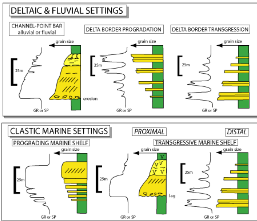
FIGURA1: MODELO DE INTERPRETAÇÃO DOS POSSÍVEIS AMBIENTES SEDIMENTARES ATRAVÉS DA COLUMA LITOLÓGICA E PERFÍL DE RAIOS GAMA.
