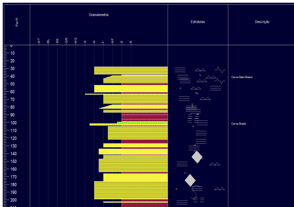
FIGURA 5: PERFIL PN 10 DIGITALIZADO COM O SOFTWARE ANASETE (PETROBRAS) CONTENDO PROFUNDIDADE DO POÇO, GRANULOMETRIA, ESTRUTURAS E LOCAIS ONDE FORAM IDENTIFICADOS DEPÓSITOS DE CARVÃO.
