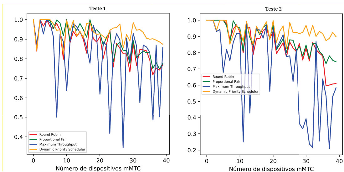
Figura 5.6: Índice de Jain calculado para os testes 1 e 2 respectivamente.
