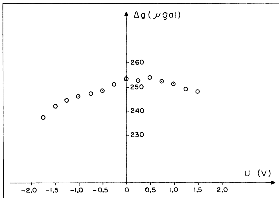
FIGURA 73 - GRAVÍMETRO III, \Delta g = f(U)
