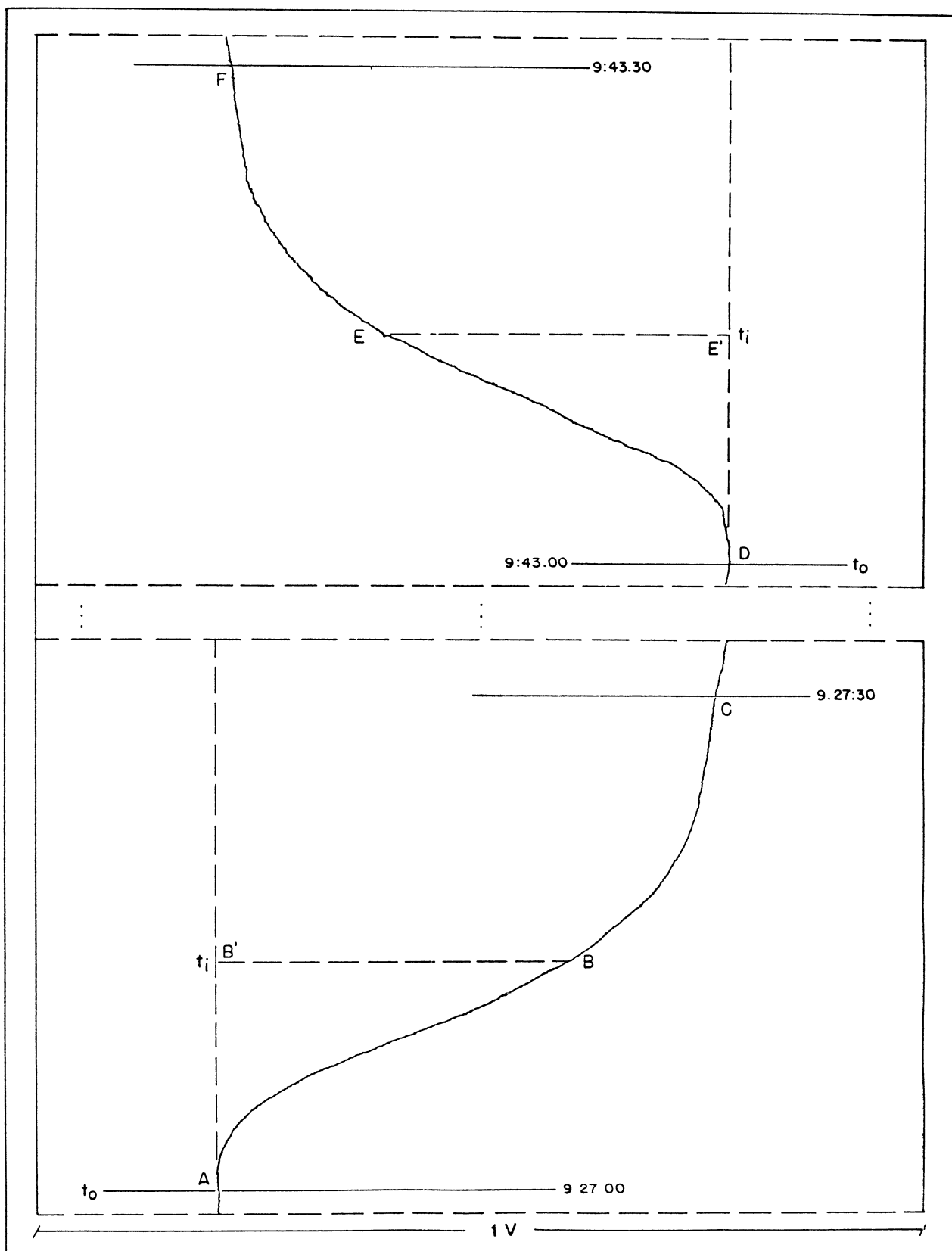
FIGURA 76 - APLICAÇÃO E REMOÇÃO DO IMPULSO INSTANTÂNEO (TENSÃO DE 17,50V APLICADA AO DISPOSITIVO ELETROSTÁTICO).
