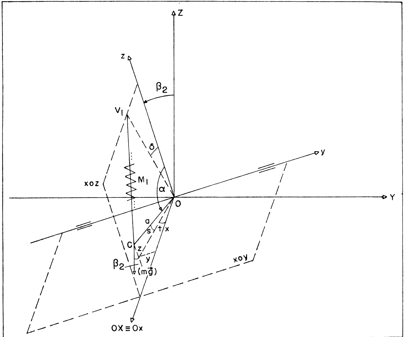
FIGURA 11 - GRAVÍMETRO INCLINADO SEGUNDO O NÍVEL II. O CENTRO DE MASSA C TEM COORDENADAS (x, y, z) NO SISTEMA INSTRUMENTAL. SUPÕE-SE NO ESQUEMA QUE A ALAVANCA DE SUSTENTAÇÃO DA MOLLA PRINCIPAL ESTEJA PARALELA A Ox \equiv OX .
