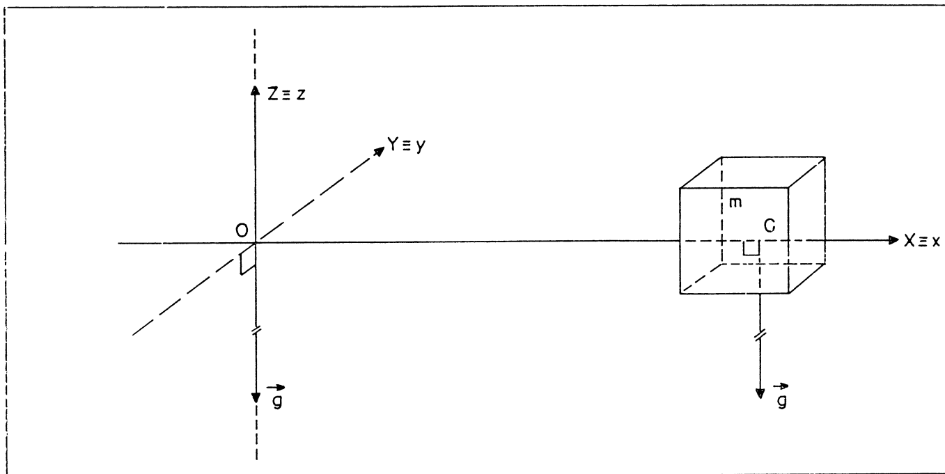
FIGURA 35 - GRAVÍMETRO NIVELADO. O VETOR g É NORMAL À VIGUETA E AO EIXO DE ROTAÇÃO. A LINHA INTERROMPIDA REPRESENTANDO O EIXO INDICA QUE A SUA REALIZAÇÃO NO GRAVÍMETRO ASKANIA É VIRTUAL.
