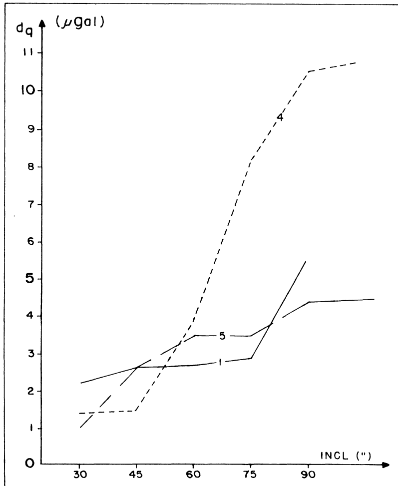
FIGURA 62 - EXPERIMENTOS IIA (INCLINA- ÇÃO SECUNDÁ- RIA)
