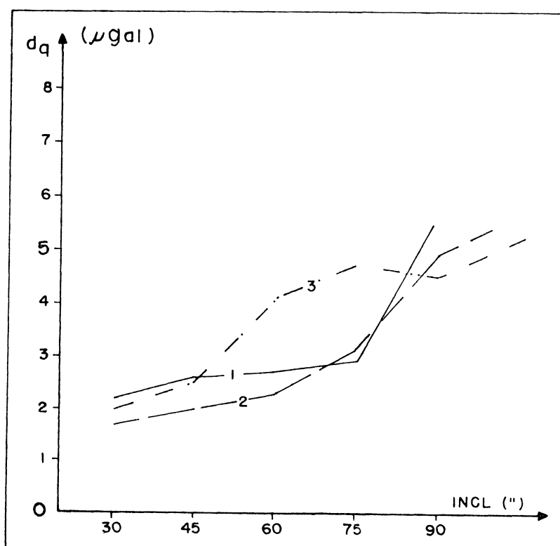
FIGURA 57 - EXPERIMENTOS IIA (VARIAÇÃO NO NÍVEL DE SAÍDA)
