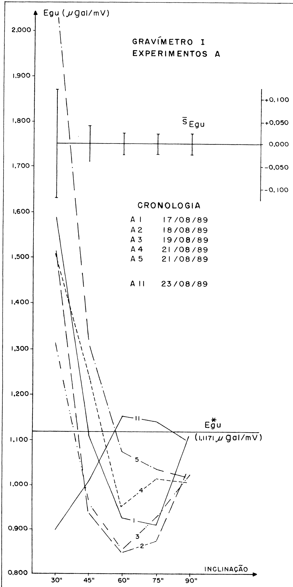
FIGURA 40 - GRAVÍMETRO I, EXPERI- MENTOS A
