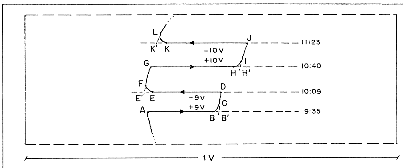
FIGURA 77 - TRECHO DO REGISTRO ANALÓGICO CORRESPONDENTE AO EXPERIMENTO COM A VARIAÇÃO DA TENSÃO DA FONTE DO DISPOSITIVO ELETROSTÁTICO DE CONTROLE DA POSIÇÃO DA VIGUETA.
