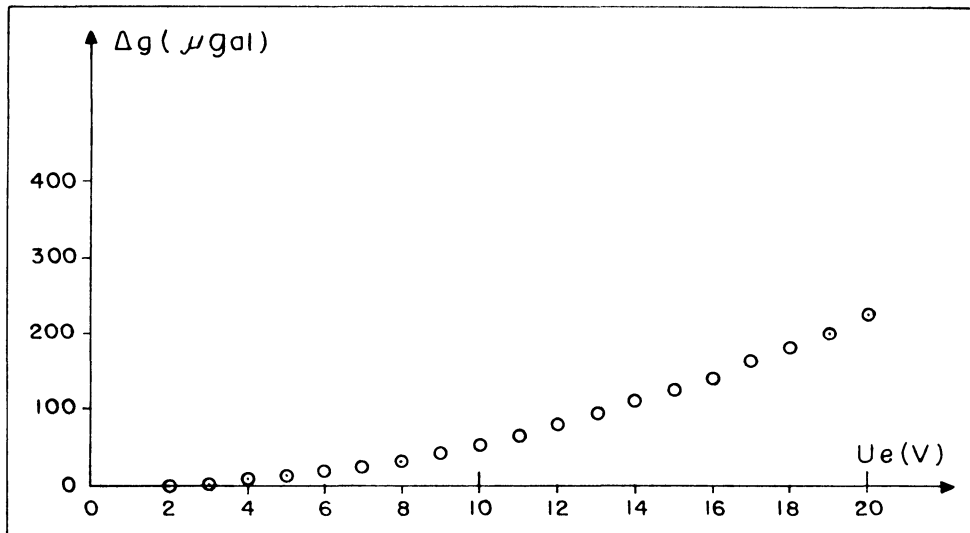
FIGURA 80 - GRAVÍMETRO V: \Delta g = f(U_e)
