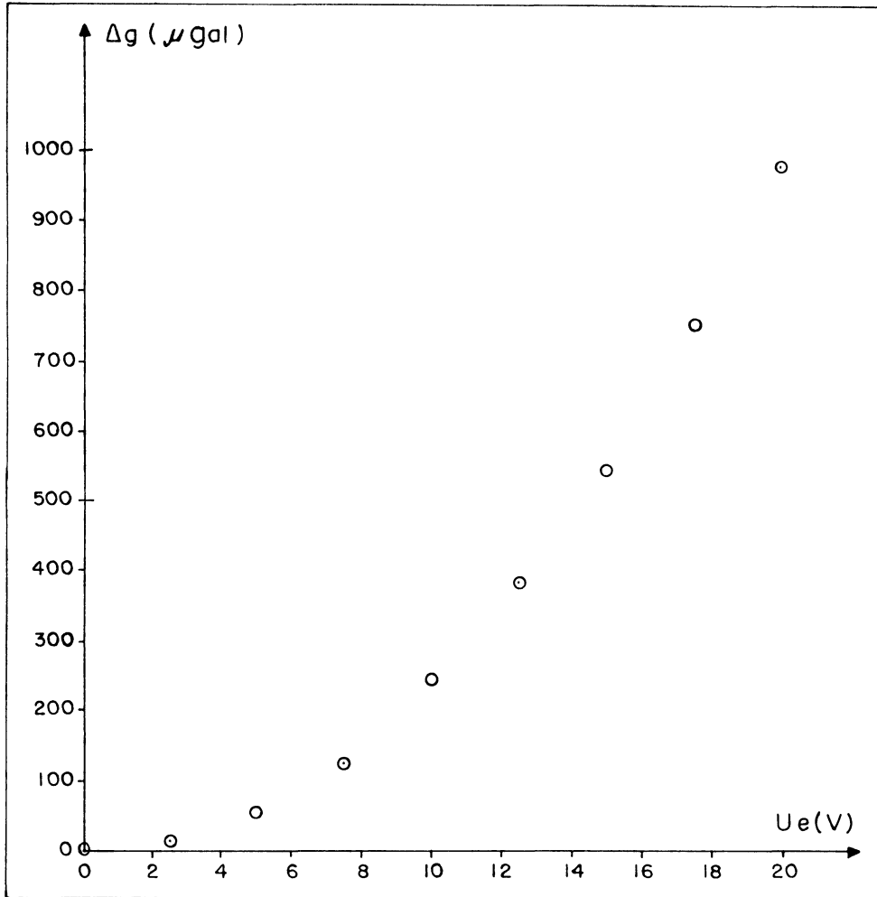
FIGURA 79 - GRAVÍMETRO IV: \Delta g = f(U_e)
