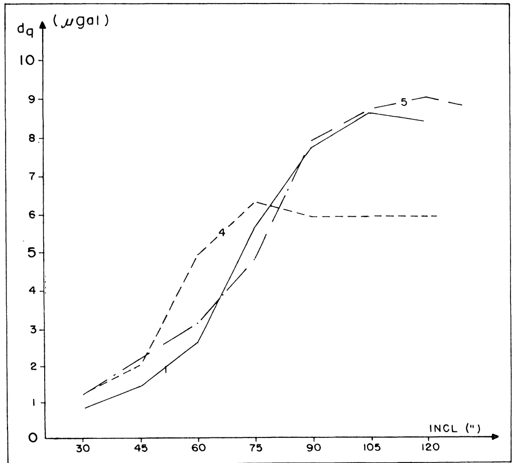
FIGURA 65 - EXPERIMENTOS VA (INCLINAÇÃO SECUNDÁRIA)
