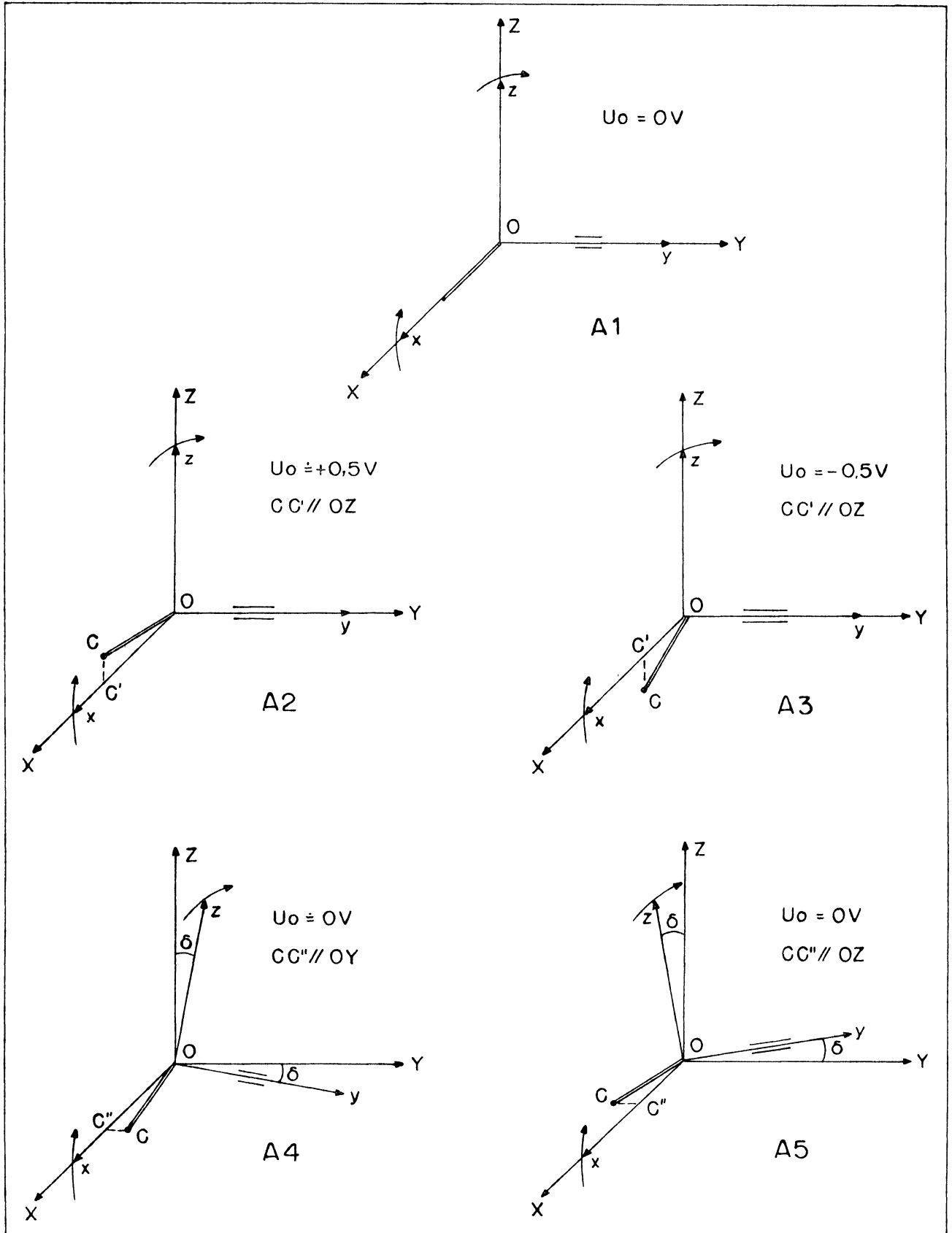
FIGURA 32 - EXPERIMENTOS EM POSIÇÃO A: CONDIÇÕES INICIAIS
