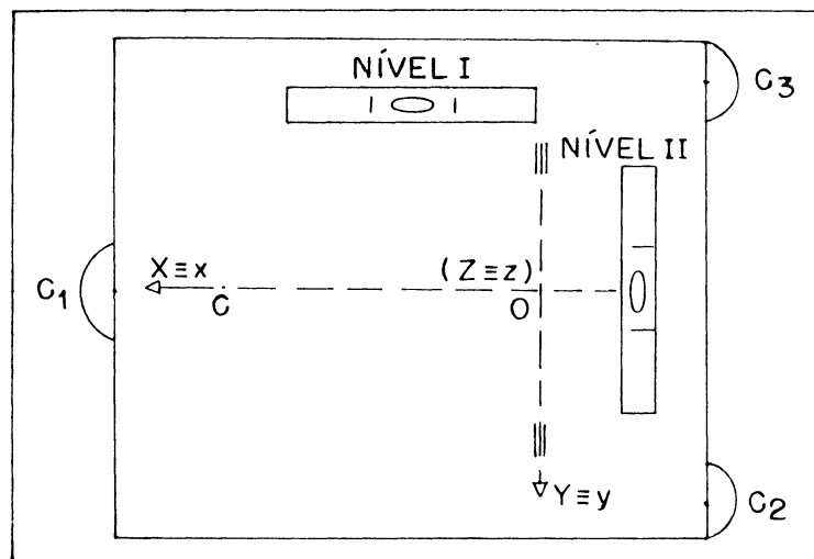
FIGURA 03 - PAINEL SUPERIOR DO GRAVÍMETRO. O NÍVEL I É SITUADO PARALELAMENTE AOS EIXOS OX \equiv O_x (NÍVEL LONGITUDINAL); O NÍVEL II É PARALELO A OY \equiv O_y (NÍVEL TRANSVERSAL) E TAMBÉM AO EIXO DE ROTAÇÃO DA VIGUETA. NA BASE DO INSTRUMENTO, OS PARAFUSOS CALANTES C_1 , C_2 E C_3 .
