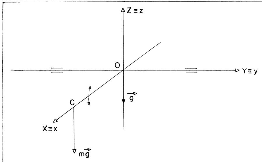
FIGURA 05 - O GRAVÍMETRO NIVELADO E A VIGUETA NA POSIÇÃO HORIZONTAL, SEU EIXO DE ROTAÇÃO COINCIDINDO COM OY \equiv Oy
