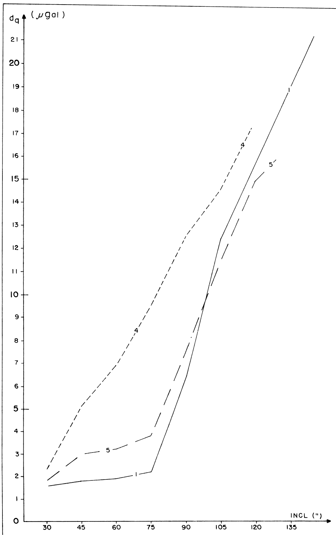
FIGURA 64 - EXPERIMENTOS IVA (INCLINAÇÃO SECUNDÁRIA)
