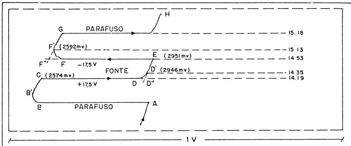
FIGURA 72 - TRECHO DO REGISTRO ANALÓGICO, MOSTRANDO UM EXEMPLO DAS OPERAÇÕES PARA O EXAME DA LINEARIDADE DA FUNÇÃO \Delta y = f(U) . O ALCANCE DE MEDIDA NO REGISTRO É DE 1V.
