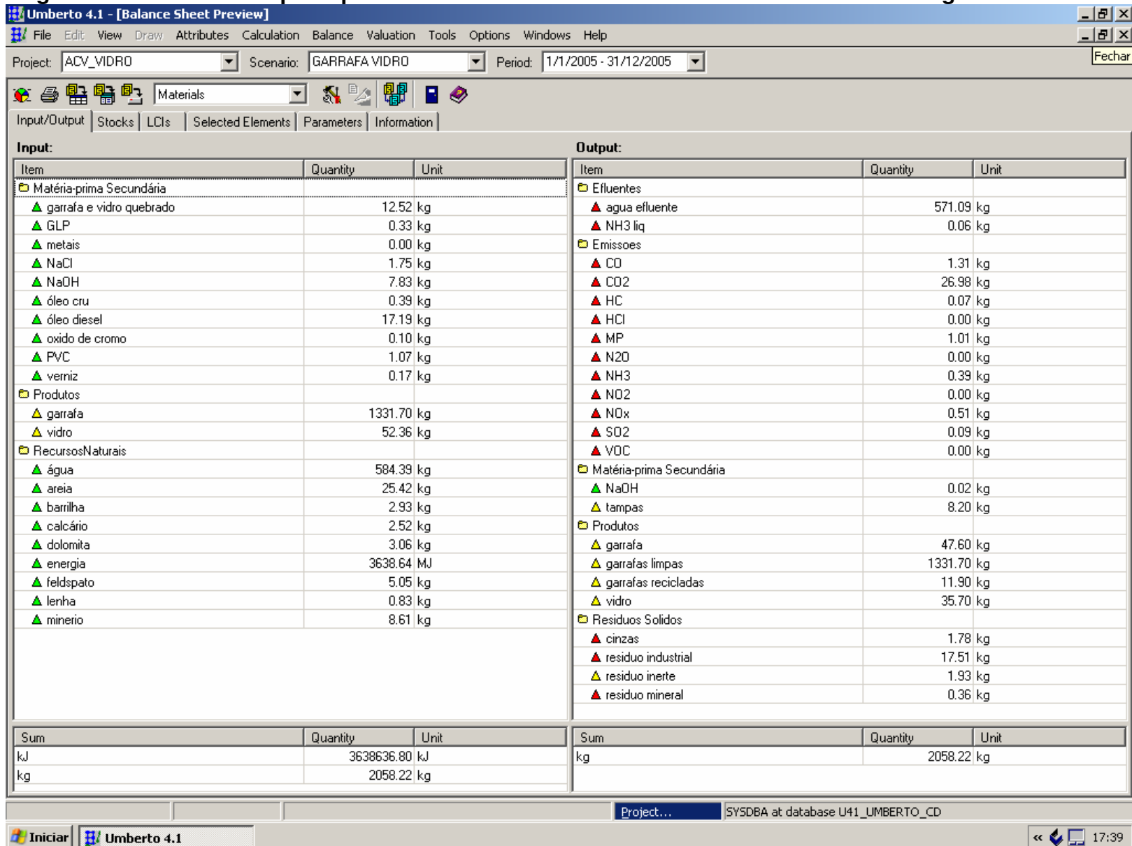
Figura 35 – Resumo das principais entradas e saídas de materiais do ciclo de vida das garrafas de vidro
