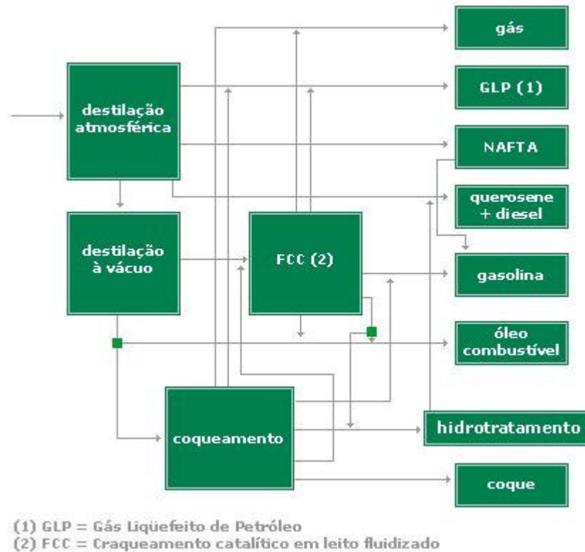
Figura 9 – Refino do Petróleo
