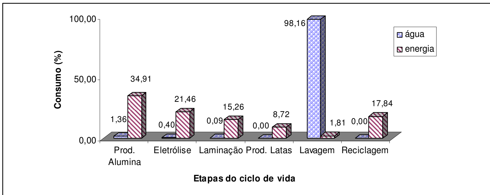
Figura 23 – Consumo de água e energia no ciclo de vida das latas de ALUMÍNIO
