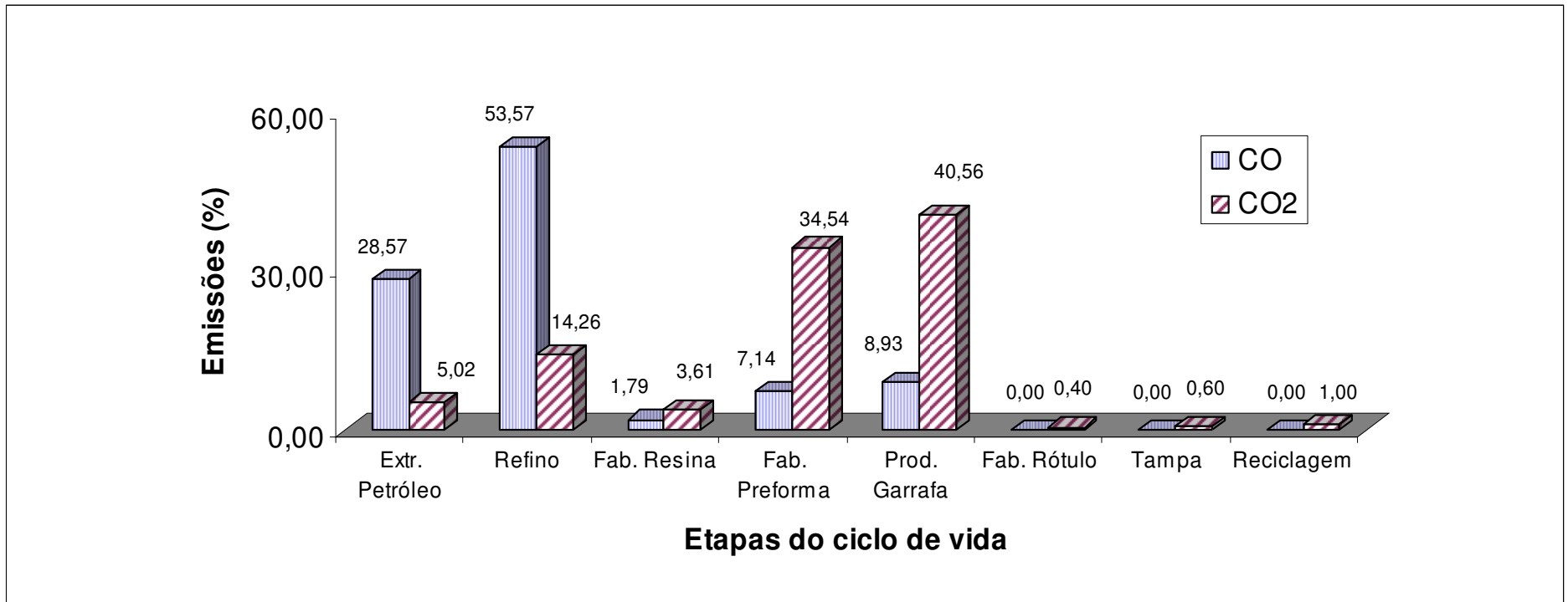
Figura 29 – Emissão de CO e CO 2 no ciclo de vida das garrafas de PET
