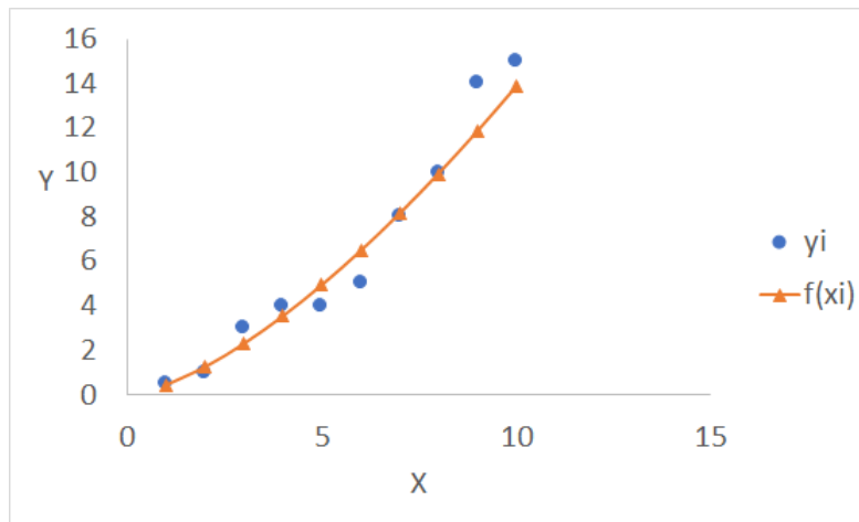
Figura 3 – Modelo geométrico para os dados da Tabela 3.
