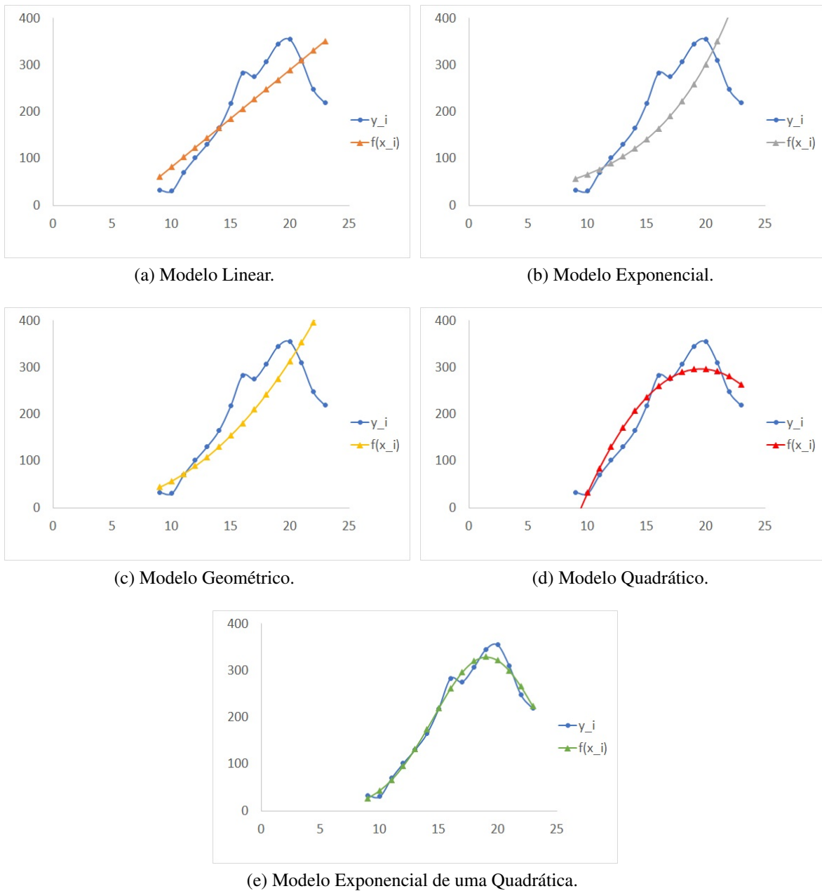
Figura 18 – Ajuste de curvas aos óbitos por COVID-19 das 15 últimas semanas no Paraná.
