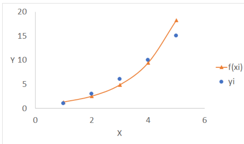
Figura 2 – Modelo exponencial para os dados da Tabela 2.
