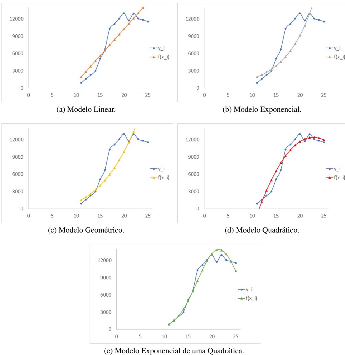
Figura 15 – Ajuste de curvas de casos de COVID-19 das 15 últimas semanas no Paraná.
