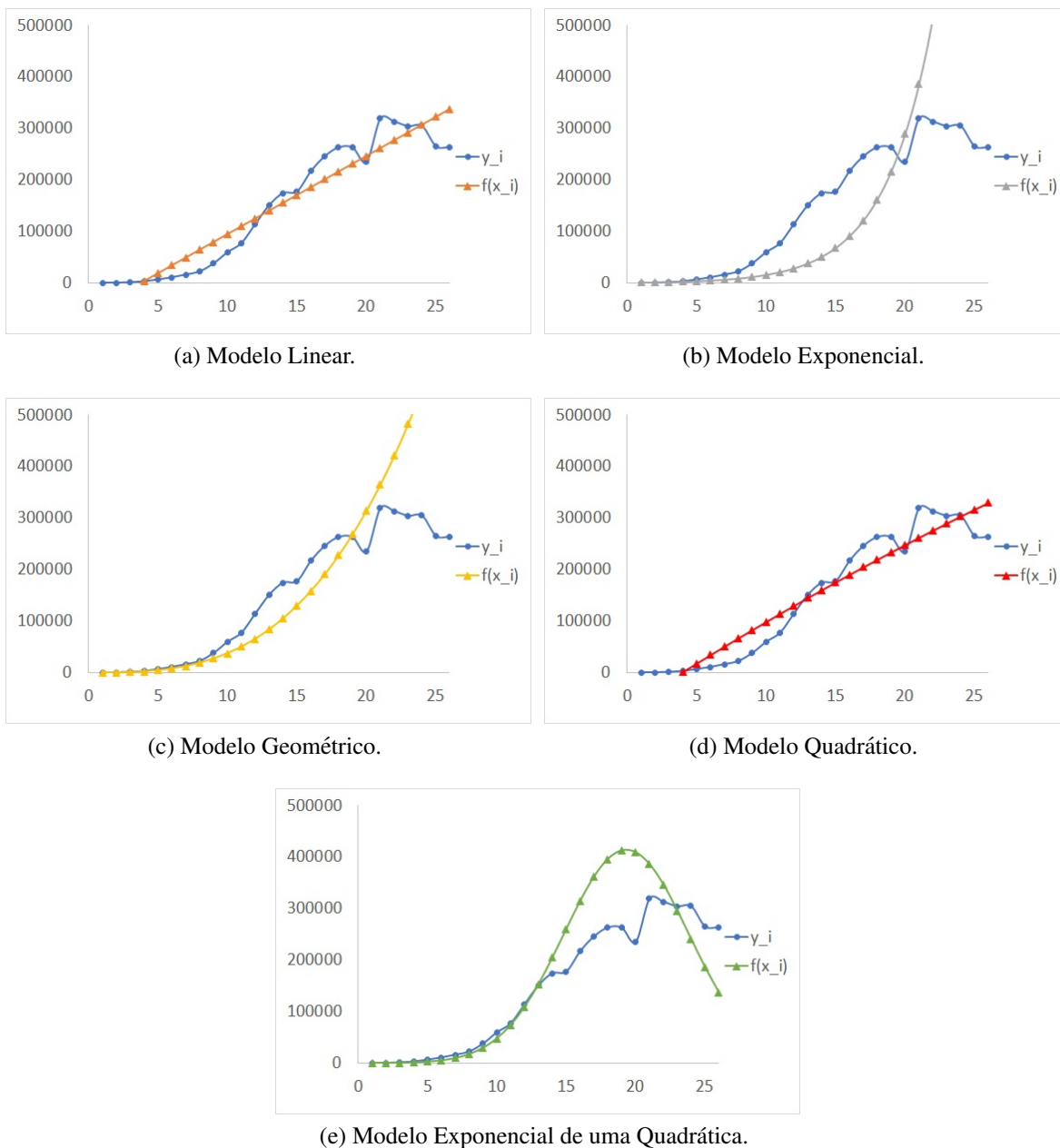
Figura 20 – Ajuste de curvas aos dados semanais de casos confirmados de COVID-19 no Brasil.
