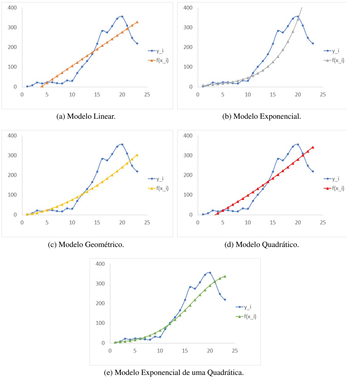
Figura 17 – Ajuste de curvas aos dados semanais de óbitos por COVID-19 no Paraná.
