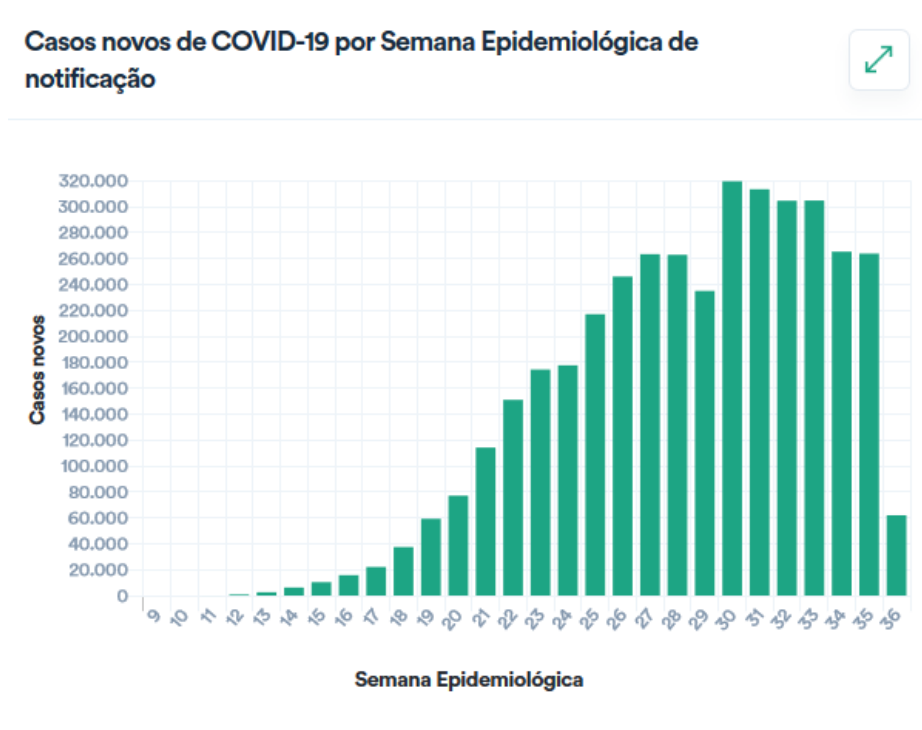
Figura 19 – Número de casos confirmados de COVID-19 no Brasil de 23/02 a 31/08/2020 [7].
