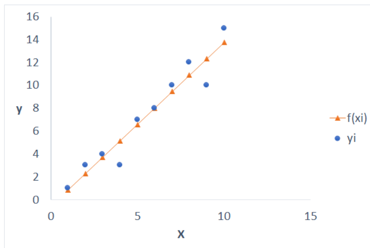
Figura 1 – Modelo linear para os dados da Tabela 1.
