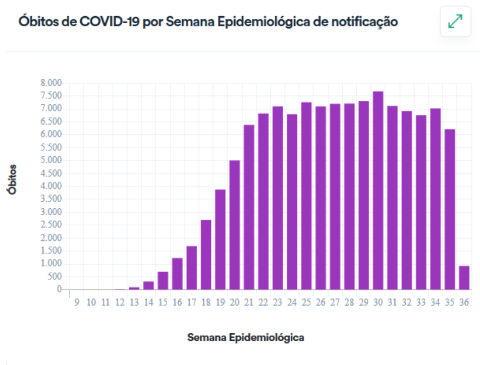
Figura 22 – Óbitos semanais de COVID-19 no Brasil 23/02 a 31/08/2020 [7].
