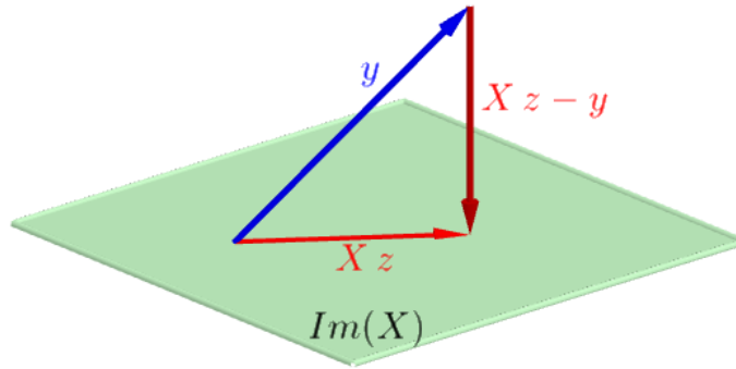
Figura 5 – Projeção do vetor y \in \mathbb{R}^3 na imagem de X \in \mathbb{R}^{3 \times 2} , com z \in \mathbb{R}^2 .
