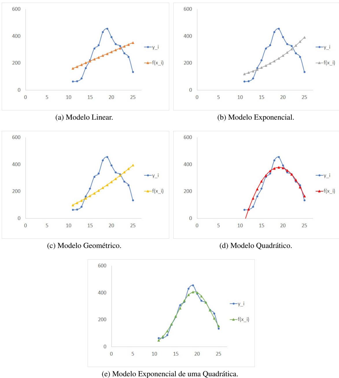
Figura 9 – Ajuste de curvas de casos de COVID-19 das 15 últimas semanas em Curitiba.
