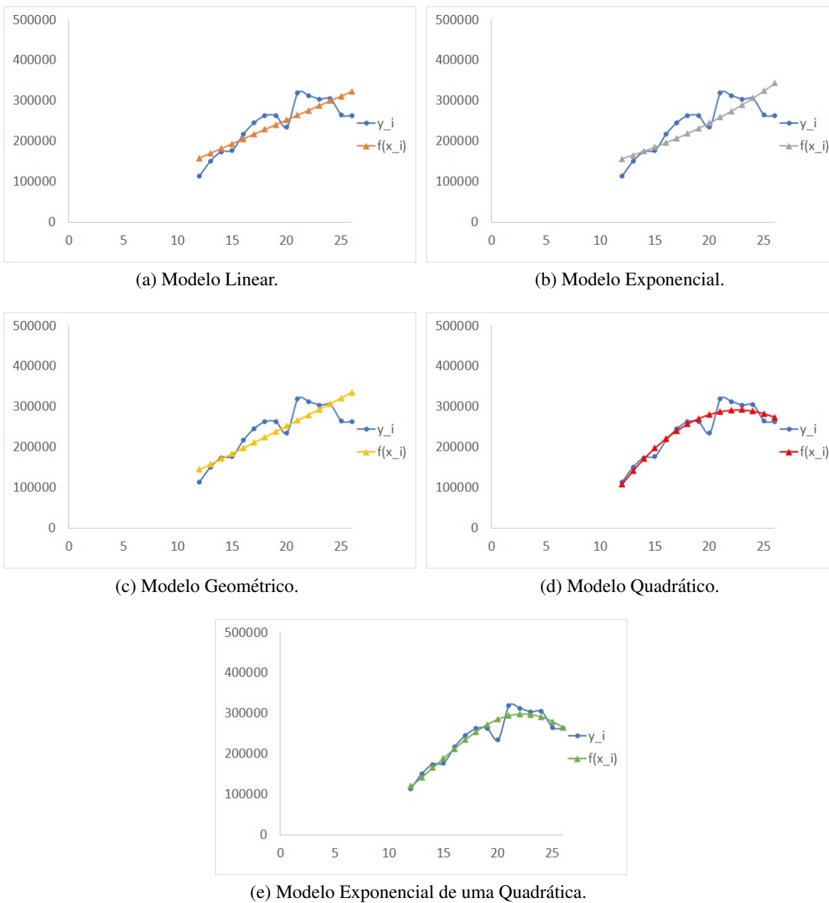
Figura 21 – Ajuste de curvas de casos de COVID-19 das 15 últimas semanas no Brasil.
