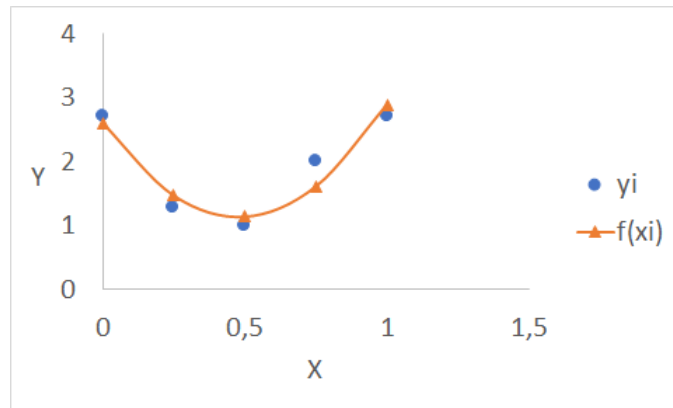
Figura 4 – Modelo quadrático para os dados da Tabela 4.
