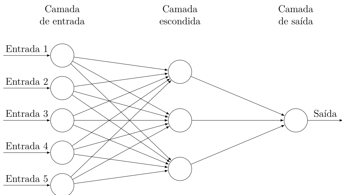
Figura 7: Esquema de uma rede neural artificial.
