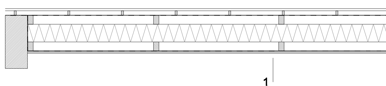
PLANTA ESTRUTURA ENTRE PÓRTICOS ESCALA 1:25
