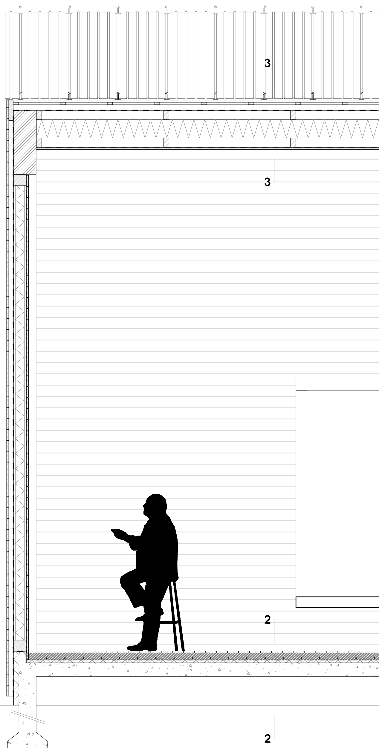
CORTE LONGITUDINAL ESCALA 1:25
