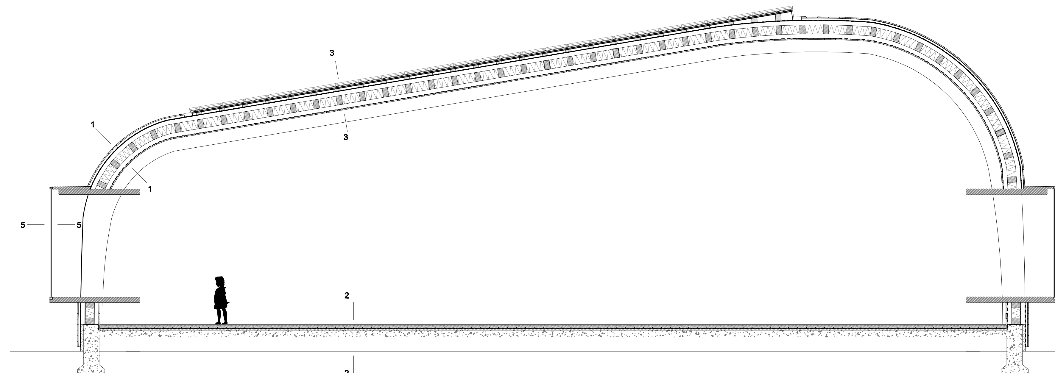
CORTE TRANSVERSAL ESCALA 1:50
