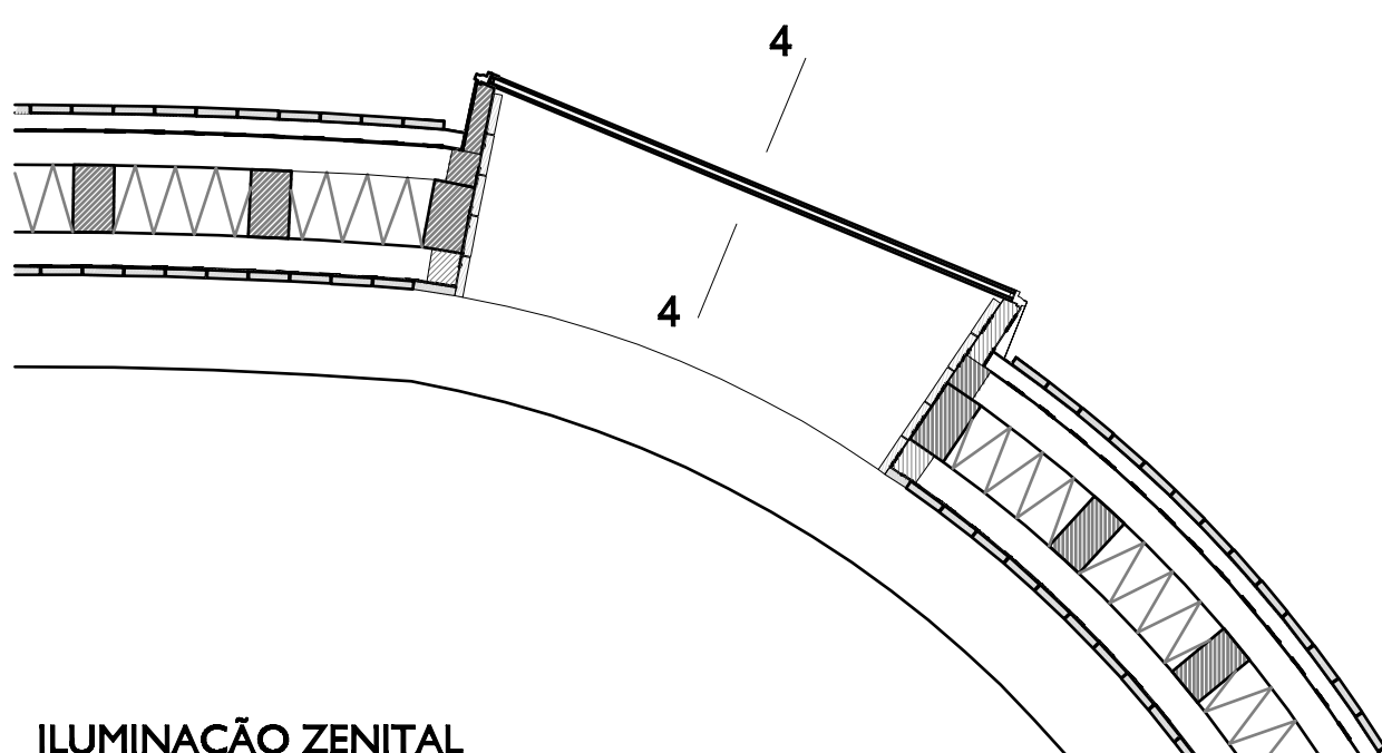
ILUMINAÇÃO ZENITAL ESCALA 1:25
