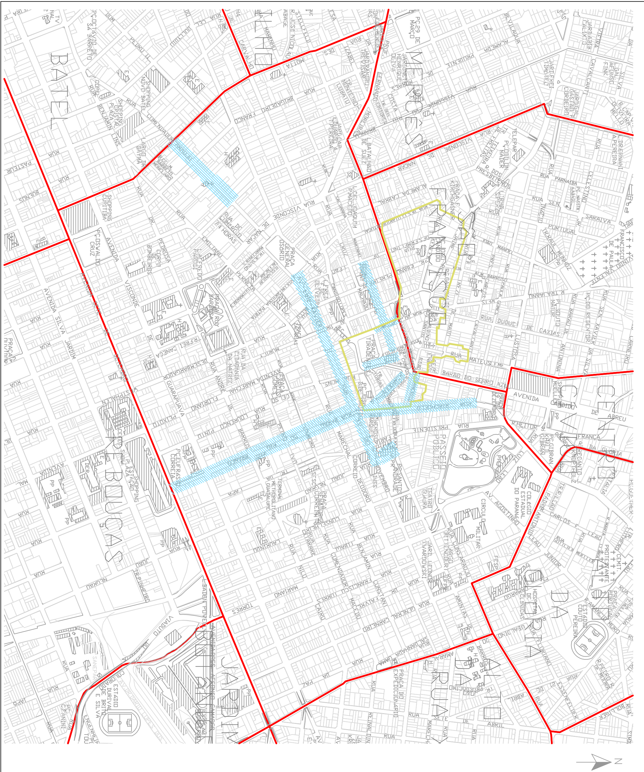
ÁREAS DE INTERESSE DE PATRIMÔNIO HISTÓRICO - Figura 70 Bairro Centro de Curitiba - ESCALA: 1/10000
