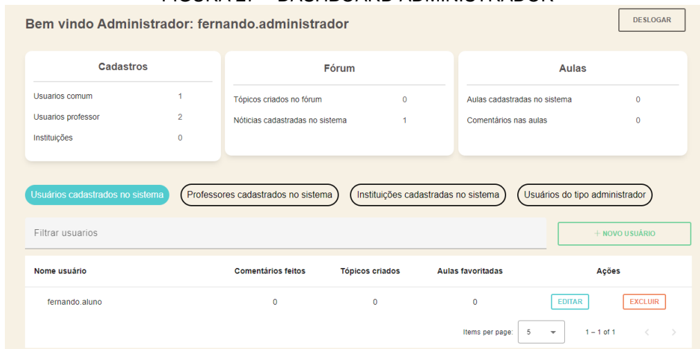
FIGURA 27 – DASHBOARD ADMINISTRADOR
