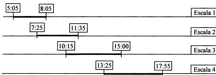
FIGURA 4.3 – EXEMPLO DE COMBINAÇÕES DE ESCALAS.
