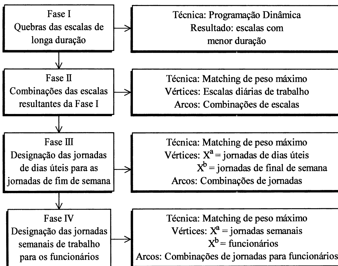
FLUXOGRAMA 4.1 – AS ETAPAS DA RESOLUÇÃO DO PROBLEMA.
