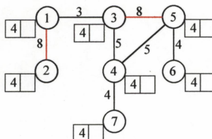
FIGURA A1.2 – GRAFO G NO PASSO INICIAL.
