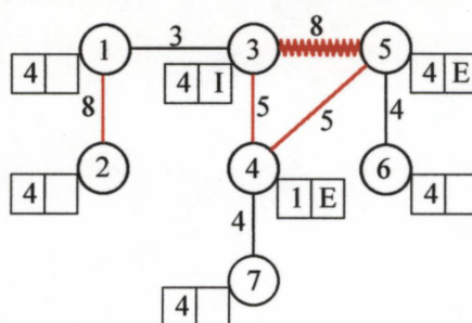
FIGURA A1.4 – GRAFO G NA SEGUNDA ATUALIZAÇÃO.
