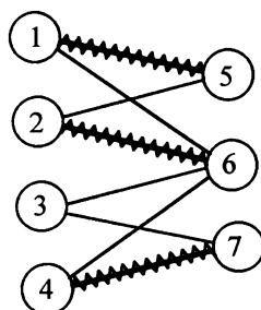
FIGURA 3.12 - EXEMPLO DE UM PROBLEMA DE DESIGNAÇÃO.
