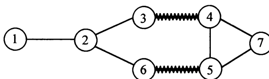
FIGURA 3.14 – EXEMPLO DE FORMAÇÃO DE UM CICLO ÍMPAR.
