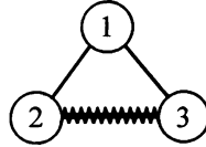
FIGURA 3.11 – EXEMPLO DE UM CONJUNTO COM CARDINALIDADE ÍMPAR.
