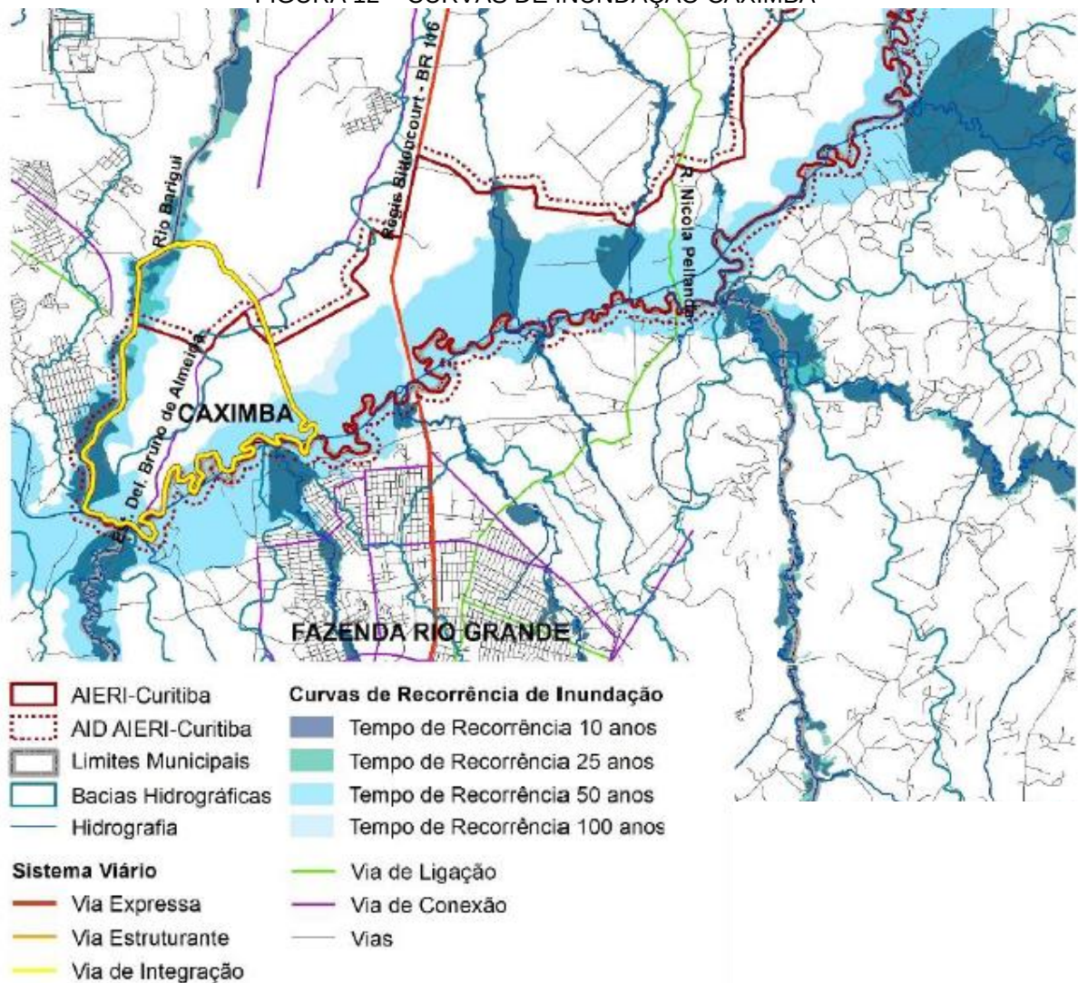
FIGURA 12 – CURVAS DE INUNDAÇÃO CAXIMBA
