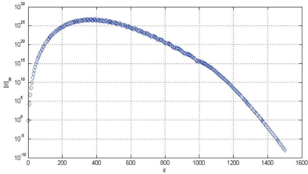
FIGURA 60 – RESÍDUO VERSUS ITERAÇÕES PARA O SINGLEGRID COM WAVEFORM RELAXATION PADRÃO - 2D.
