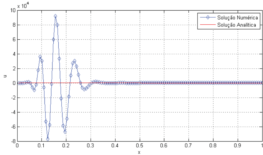
FIGURA 40 – SOLUÇÃO APROXIMADA COM 2 ITERAÇÕES DO SINGLEGRID COM WAVEFORM RELAXATION PADRÃO - 1D.
