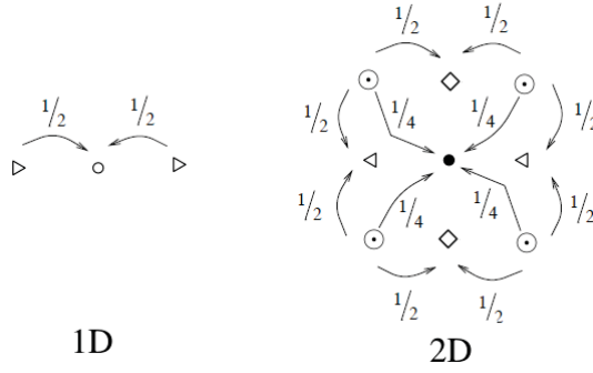
FIGURA 12 – INTERPOLAÇÃO LINEAR E BILINEAR.
