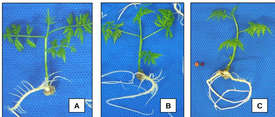
FIGURA 23 – Microestacas de Melia azedarach L. enraizadas em meio (A) MS/2+2,46 \mu M de AIB (incremento na altura do caule); (B) MS/2+4,92 \mu M de AIB (número de raízes e porcentagem de enraizamento); (C) MS+9,84 \mu M de AIB (número de raízes).
