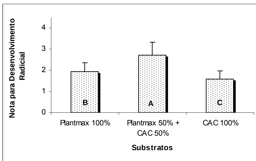
FIGURA 12 – Comparação das médias dos tratamentos na segunda fase de aclimatização de microestacas de Melia azedarach , L. enraizadas in vitro , para a variável nota para desenvolvimento radicial.
