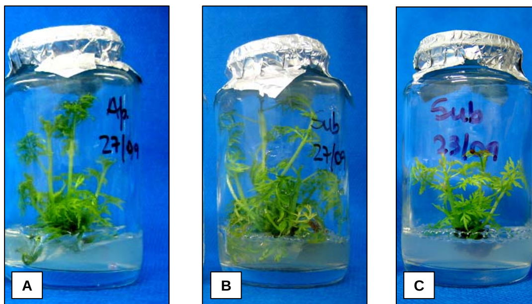
FIGURA 24 – Microestacas de Melia azedarach L. multiplicadas em meio (A) MS+1,66 de BAP (apical); (B) MS+1,66 \mu M de BAP (subapical) – número de brotos e de gemas por explante; (C) MS+3,33 \mu M de BAP (subapical) – número de brotos e formação de calo na base da brotação.
