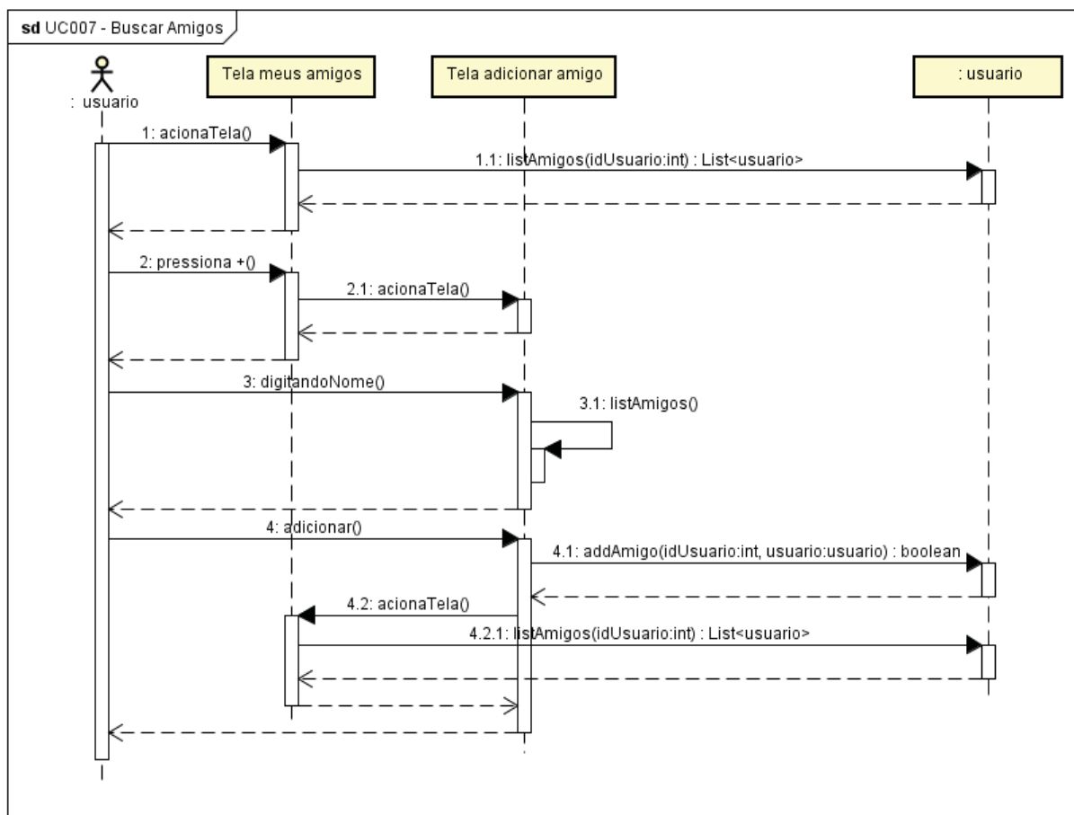
FIGURA 37 - SEQUENCIA BUSCA DE AMIGOS
