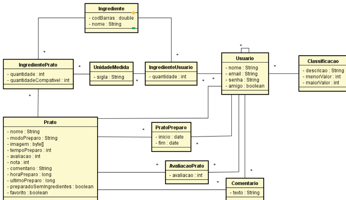
FIGURA 30 - DIAGRAMA DE CLASSE COM ATRIBUTOS
