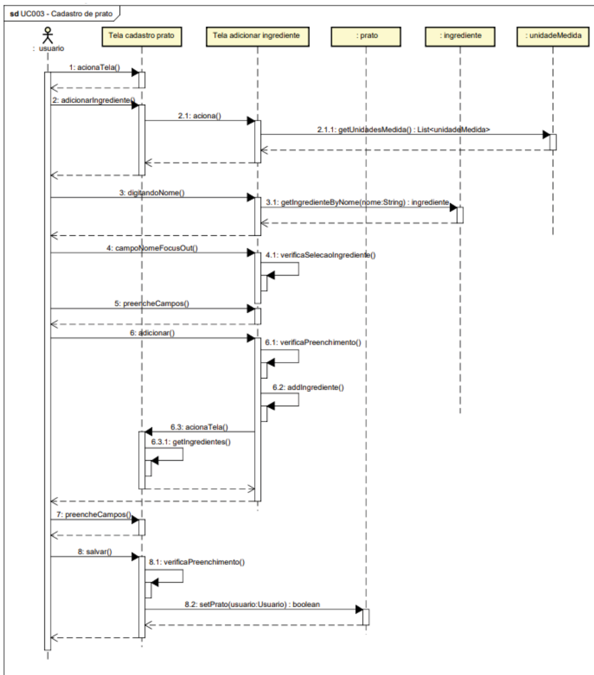
FIGURA 33 – SEQUENCIA CADASTRO DE PRATO
