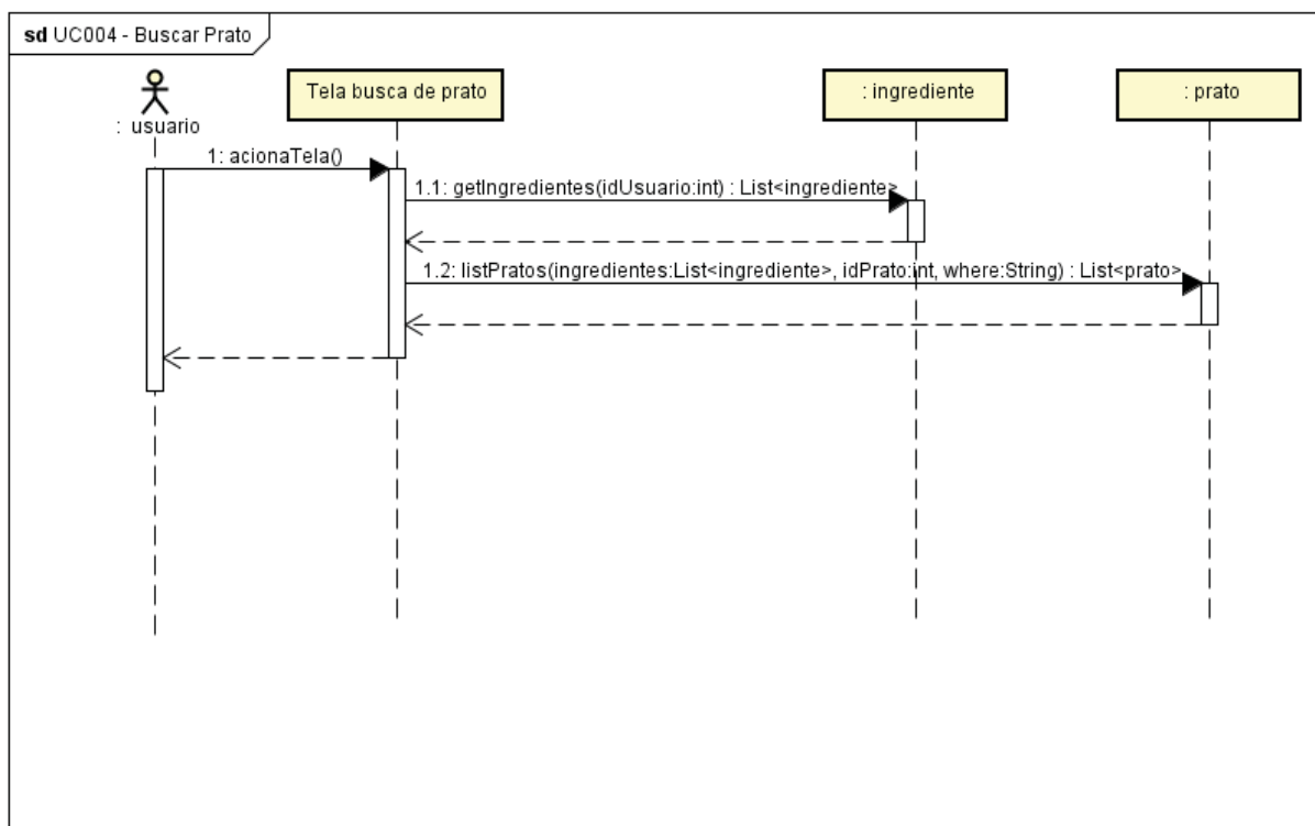
FIGURA 34 - SEQUENCIA BUSCA DE PRATO
