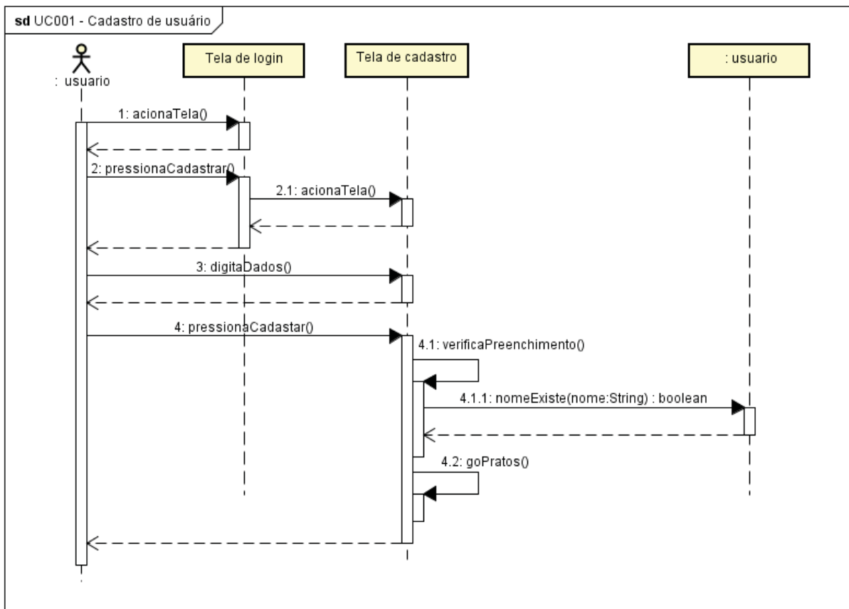
FIGURA 31 - SEQUENCIA CADASTRO DE USUÁRIO
