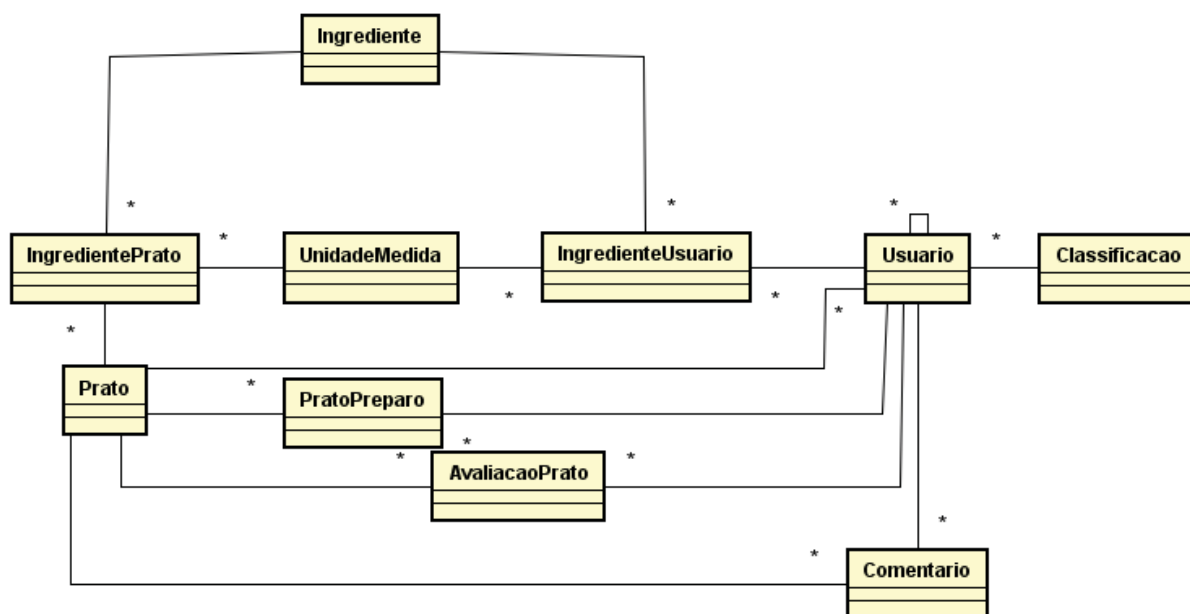
FIGURA 28 - DIAGRAMA DE CASSES NEGOCIAL
