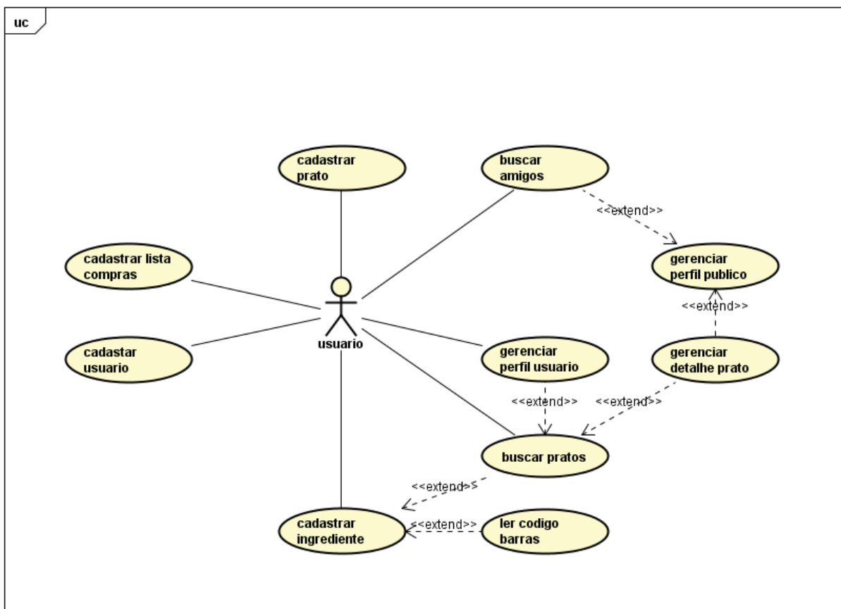
FIGURA 29 - DIAGRAMA DE CASO DE USO COMPLETO
