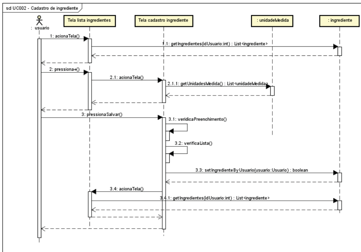
FIGURA 32 - SEQUENCIA CADASTRO DE INGREDIENTES
