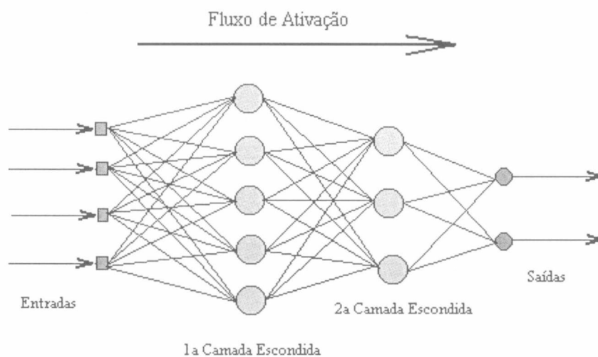
FIGURA 4 - EXEMPLO DE REDE NEURAL MULTI-CAMADAS FEEDFORWARD , TOTALMENTE CONECTADA FONTE: (DYMINSKI, 2000)
