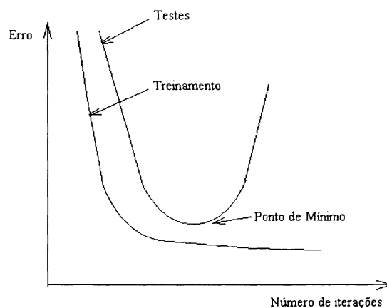
FIGURA 5 - TREINAMENTO VERSUS CAPACIDADE DE GENERALIZAÇÃO DA RN FONTE: (DYMINSKI, 2000)
