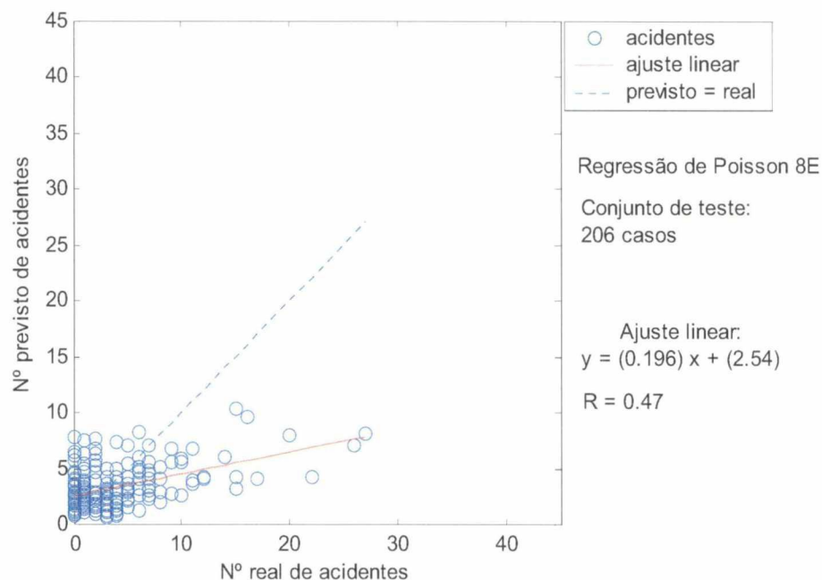
FIGURA 17 - GRÁFICO DE ACIDENTES (REAL X PREVISTO) DO MODELO P8E - CONJUNTO DE TESTE
