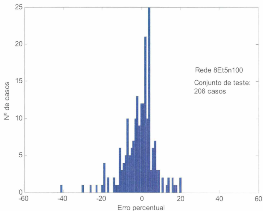
FIGURA 7 - HISTOGRAMA DA REDE 8Et5n100 - CONJUNTO DE TESTE
