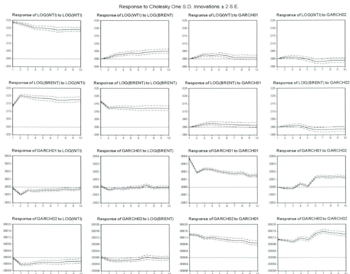
FIGURA 4 - FUNÇÕES DE IMPULSO-RESPOSTA
