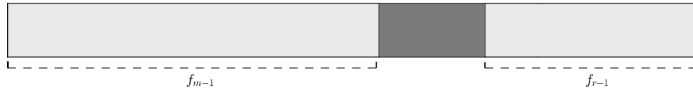
FIGURA 12 – REPRESENTAÇÃO DA DISTRIBUIÇÃO DE PEÇAS EM UM CANTEIRO DE LARGURA m + r ONDE NÃO SEJA VIÁVEL SEPARAR NA LARGURA m
