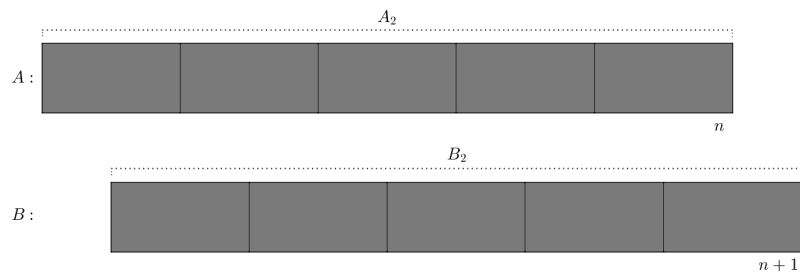
FIGURA 32 – REPRESENTAÇÃO DE CANTEIROS, DE MESMO TAMANHO, COMPOSTOS POR APENAS BLOCOS RETANGULARES
