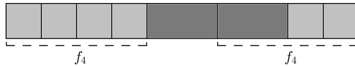
FIGURA 8 – ILUSTRAÇÃO DE UM CASO PARTICULAR DA IDENTIDADE 3.1, NO CASO n = 5 , ONDE A PEÇA CENTRAL DO CANTEIRO É UM RETÂNGULO
