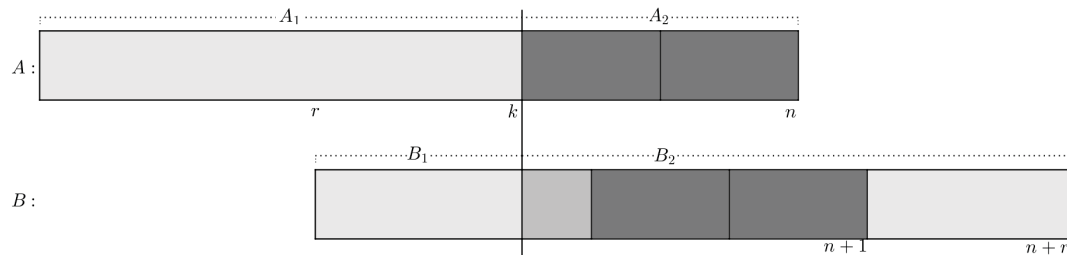
FIGURA 34 – IMAGEM QUE REPRESENTA DOIS CANTEIROS DE LARGURA n , COM B DESLOCADO EM r UNIDADES DE A , ONDE k É A ÚLTIMA CÉLULA SEPARÁVEL DE A E B . NOMEOU-SE AS PARTES OBTIDAS DESTA SEPARAÇÃO
