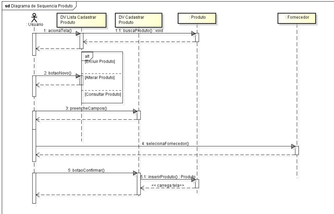
Cadastrar Produto, fonte: o autor (2014)
