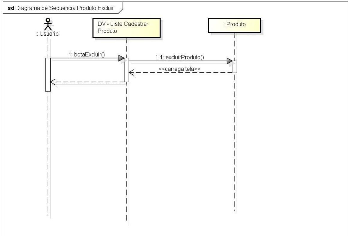
Cadastrar Produto - Excluir, fonte: o autor (2014)
