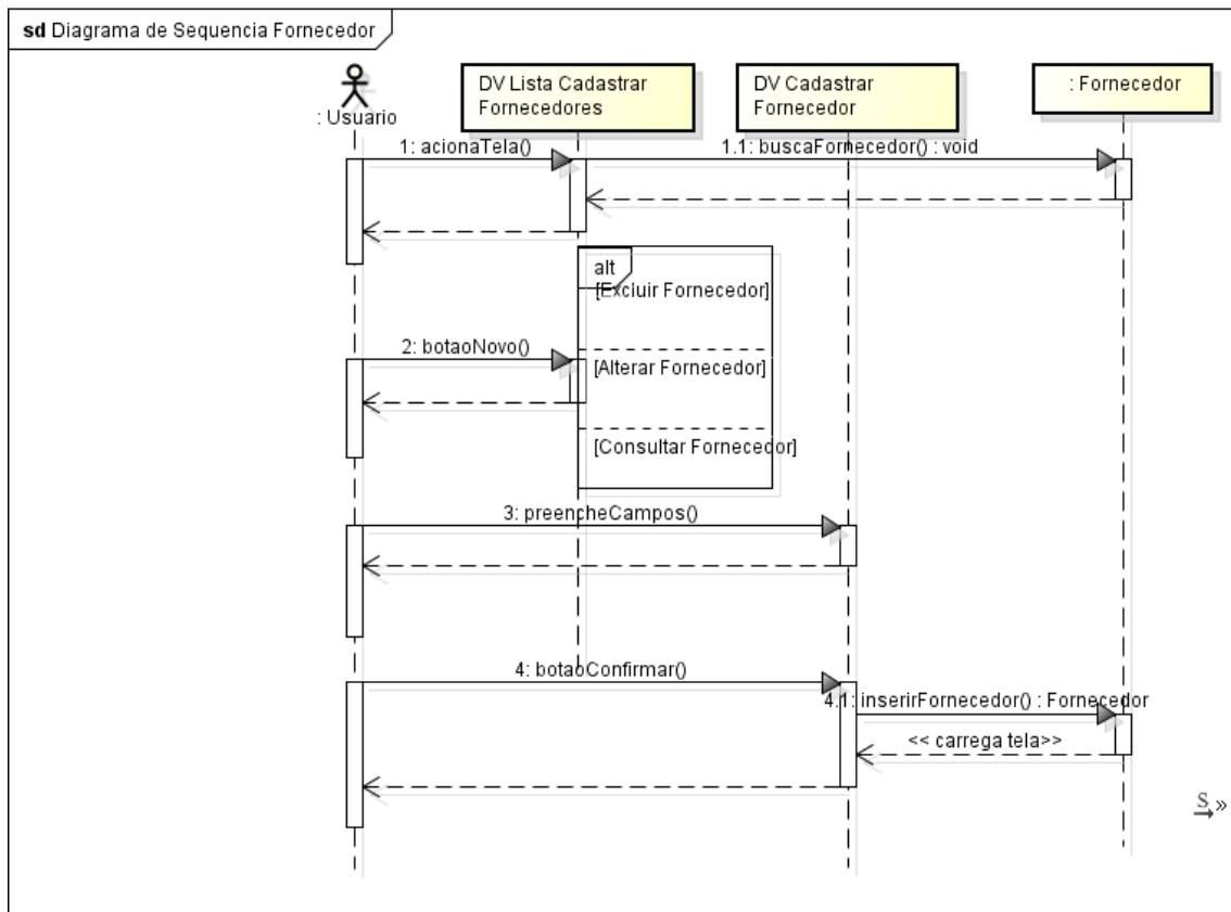
Cadastrar Fornecedor, fonte: o autor (2014)
