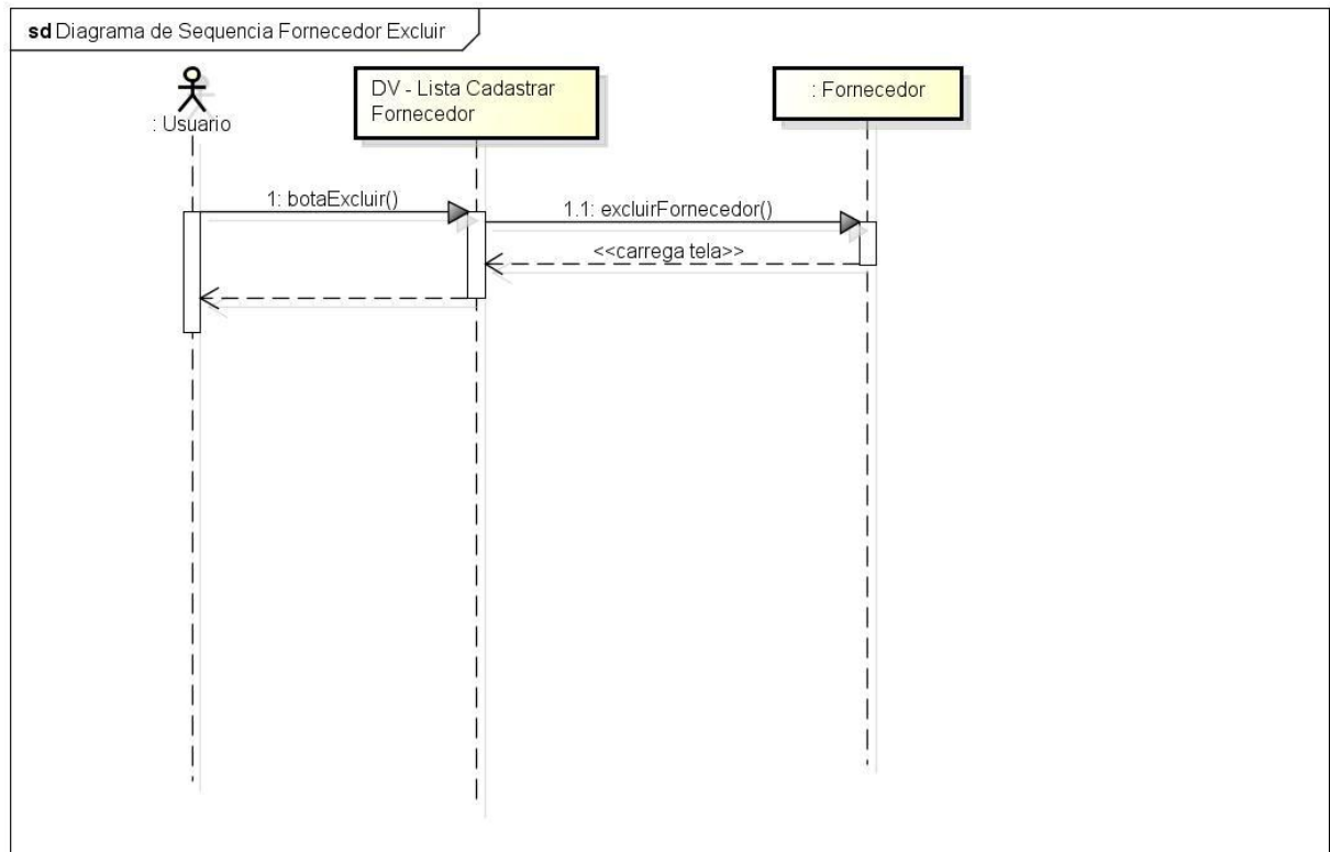
Cadastrar Fornecedor - Excluir, fonte: o autor (2014)
