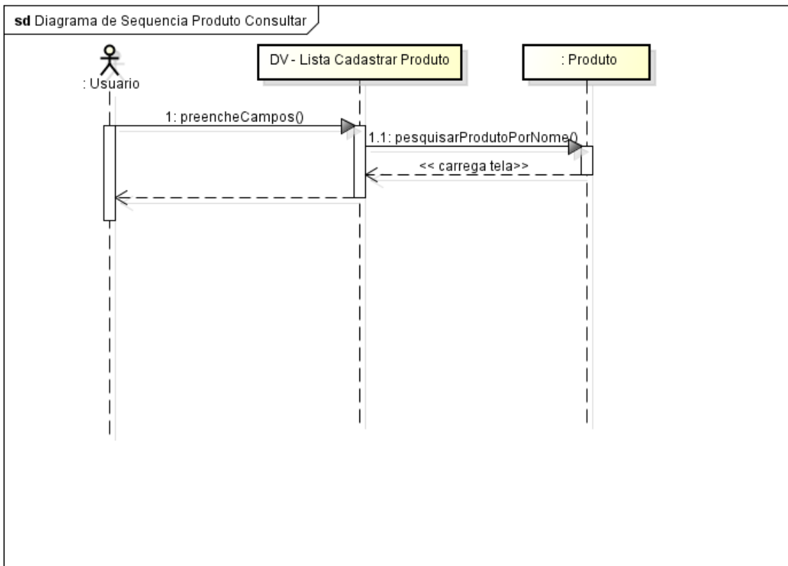
Cadastrar Produto - Consultar, fonte: o autor (2014)
