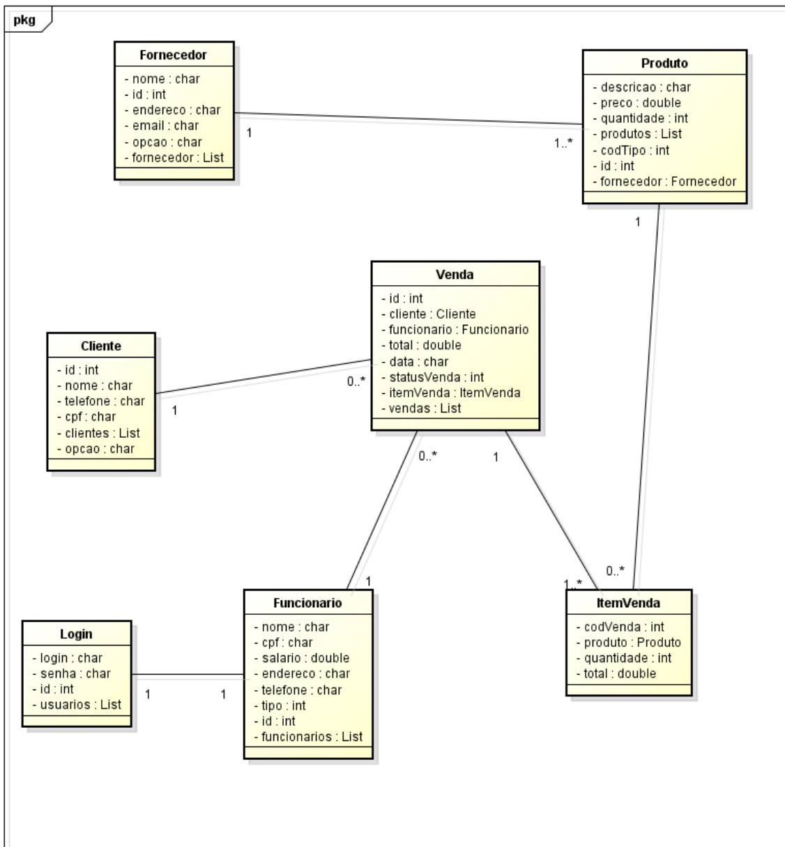
Modelo de objetos, fonte: o autor (2014)
