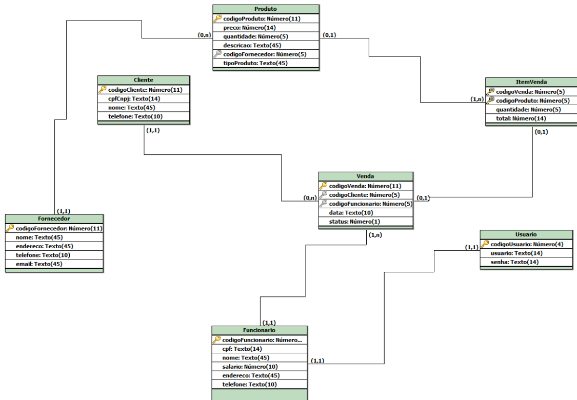
Modelo Banco de Dados, fonte: o autor (2014)
