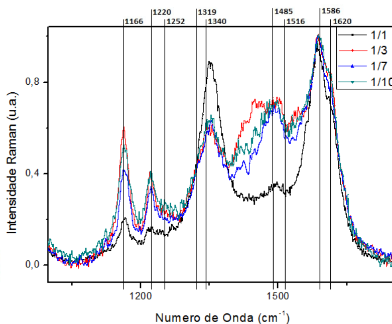
Figura 25 – Diagrama por espectroscopia Raman para os filmes de NTC/PANI base esmeraldina (concentrações 1/1, 1/3, 1/7 e 1/10) depositados sobre substrato de silício, na região entre 1000\text{ cm}^{-1} e 1700\text{ cm}^{-1} .
