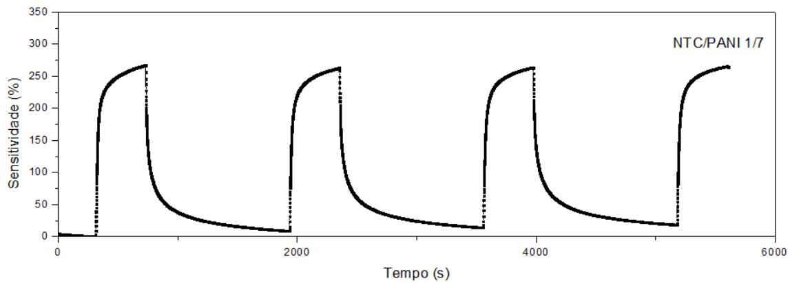
Figura 39 – Curva de sensibilidade para dispositivos baseados em filmes de NTC/PANI dopada com H_2SO_4 (proporção 1/7).
