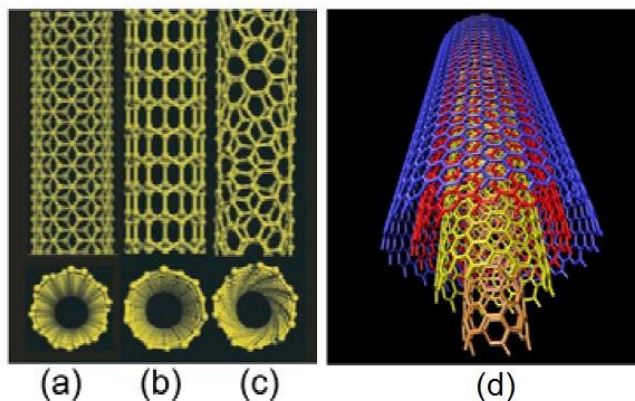
Figura 7 – (a) SWCNT Armchair. (b) SWCNT Zigzag. (c) SWCNT Chiral e (d) MWCNT. Adaptada de [39].
