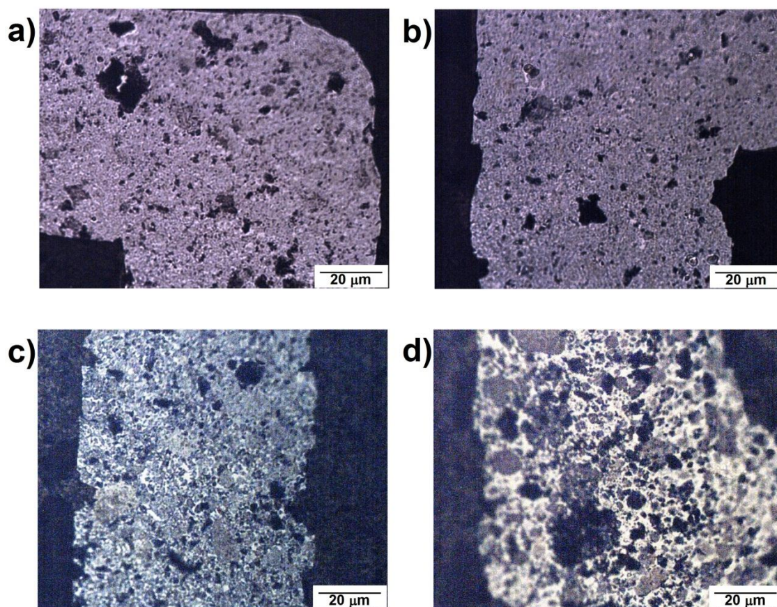
Figura 42- Imagens a partir de microscopia ótica de filmes de NTC/PANI sobre eletrodos de Cr/Au, com magnificação de 1000 vezes. Proporções 1/1 (a), 1/3 (b), 1/7 (c) e 1/10 (d).
