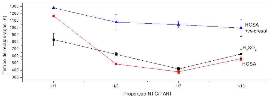
Figura 46 – Representação gráfica para tempos de recuperação para sensibilidade a 1000 PPM de amônia (NH 3 ) em ar para filmes de NTC/PANI com dopagem primária de H 2 SO 4 , dopagem primária de HCSA e dopagem secundária de HCSA mais m-cresol.
