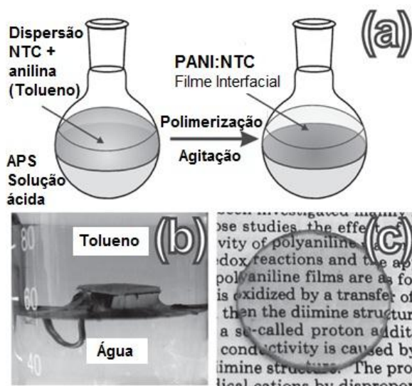
Figura 16 – Esquema para obtenção de filmes de PANI e NTC/PANI, através do método automontado. a) Dispersão de NTC e anilina em meio aquoso, agitação de 24h e formação do filme na interface dos líquidos. b) “Pesca” do filme sobre o substrato. c) Filme de Polianilina mais NTC. Adaptado de [67]
