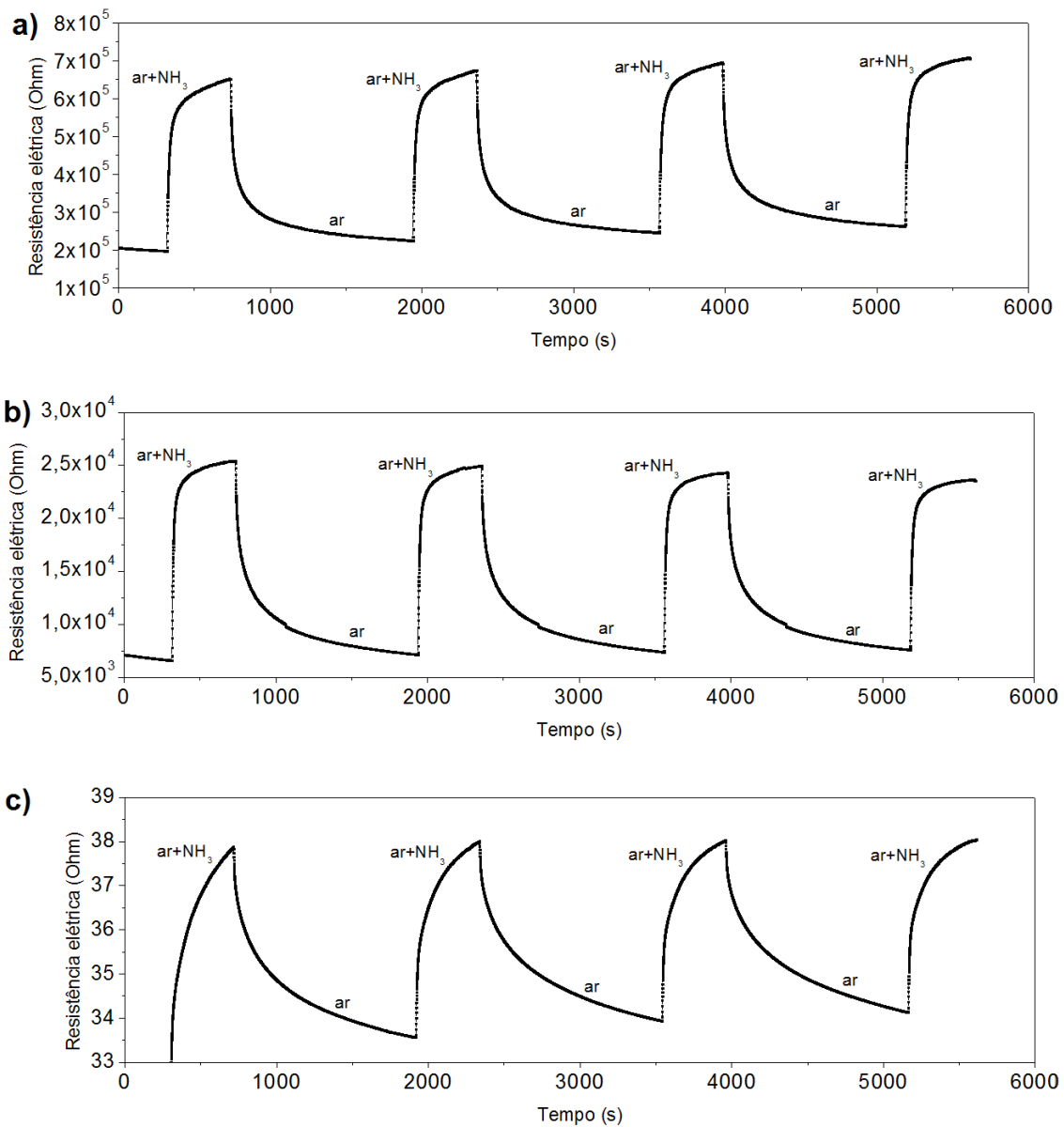
Figura 37 – Curvas de sensibilidade a 1000 PPM de NH 3 em ar para sensor com filme de camada ativa NTC/PANI, proporção 1/10, com dopagem primária de H 2 SO 4 em (a), dopagem primária de HCSA em (b) e dopagem secundária de HCSA mais m-cresol em (c).
