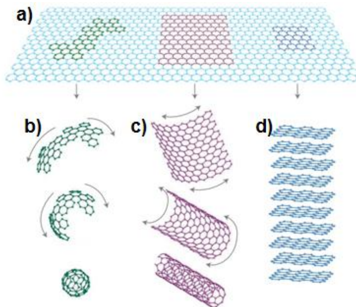
Figura 1 – Grafeno é uma estrutura 2D (a), base para outras formas de grafite. Estruturas 0D são fulerenos (buckyballs) (b), 1D são Nanotubos de Carbono (c) e 3D são grafites (d) e diamantes [10].
