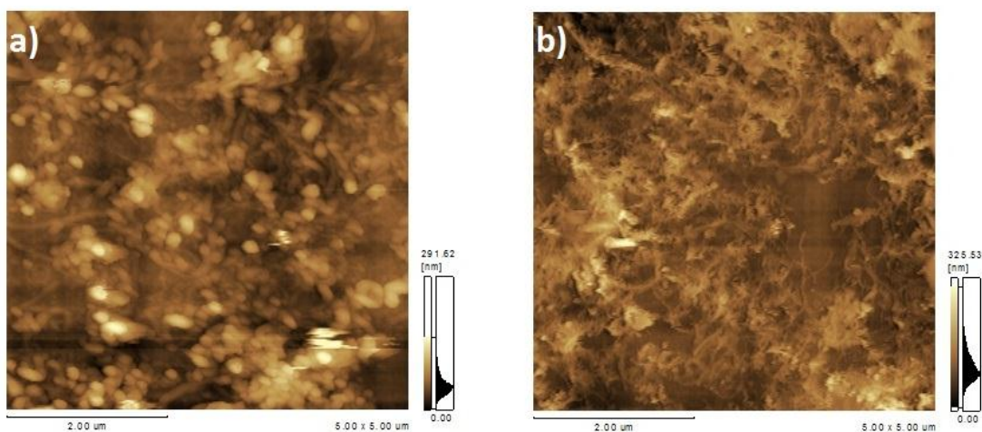
Figura 27 – Imagens a partir da técnica de microscopia de força atômica de filmes do compósito NTC/PANI. a) Filme com dopagem primária de H 2 SO 4 . b) Filme com dopagem secundária de HCSA e m-cresol.
