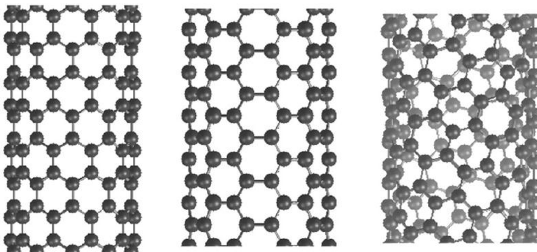
Figura 6 – Nanotubos de carbono de parede única, com diferentes quiralidades: zigzag (a esquerda), armchair (no centro) e chiral (a direita) [40].
