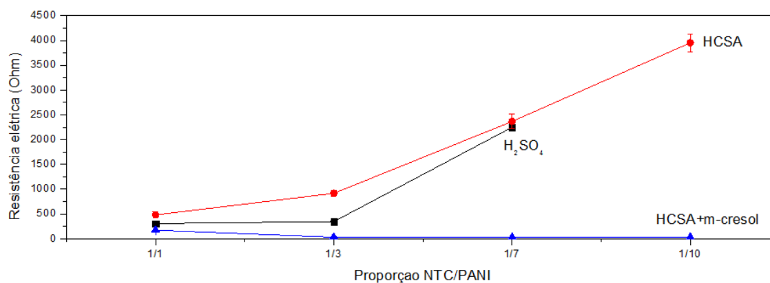
Figura 44 – Representação gráfica para valores de medida padrão de resistência elétrica entre dois contatos para filmes de NTC/PANI com dopagem primária de H_2SO_4 , dopagem primária de HCSA e dopagem secundária de HCSA mais m -cresol, medidos em fluxo de ar (5L/min) durante 1200 segundos (20 minutos).
