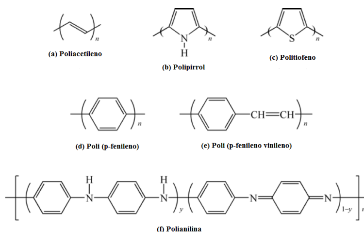
Figura 11 – Estrutura molecular de alguns polímeros condutores. (a) Poliacetileno. (b) Polipirrol. (c) Politiofeno. (d) Poli (p-fenileno). (e) Poli (p-fenileno vinileno). (f) Polianilina. Adaptado de [47].
