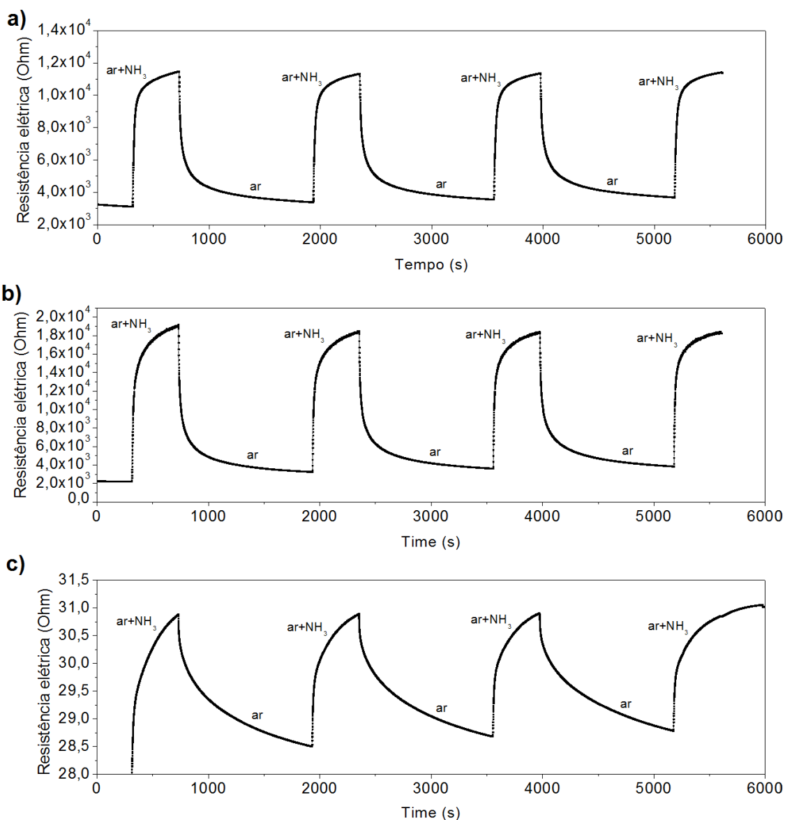
Figura 36– Curvas de sensibilidade a 1000 PPM de NH 3 em ar para sensor com filme de camada ativa NTC/PANI, proporção 1/7, com dopagem primária de H 2 SO 4 em (a), dopagem primária de HCSA em (b) e dopagem secundária de HCSA mais m -cresol em (c).
