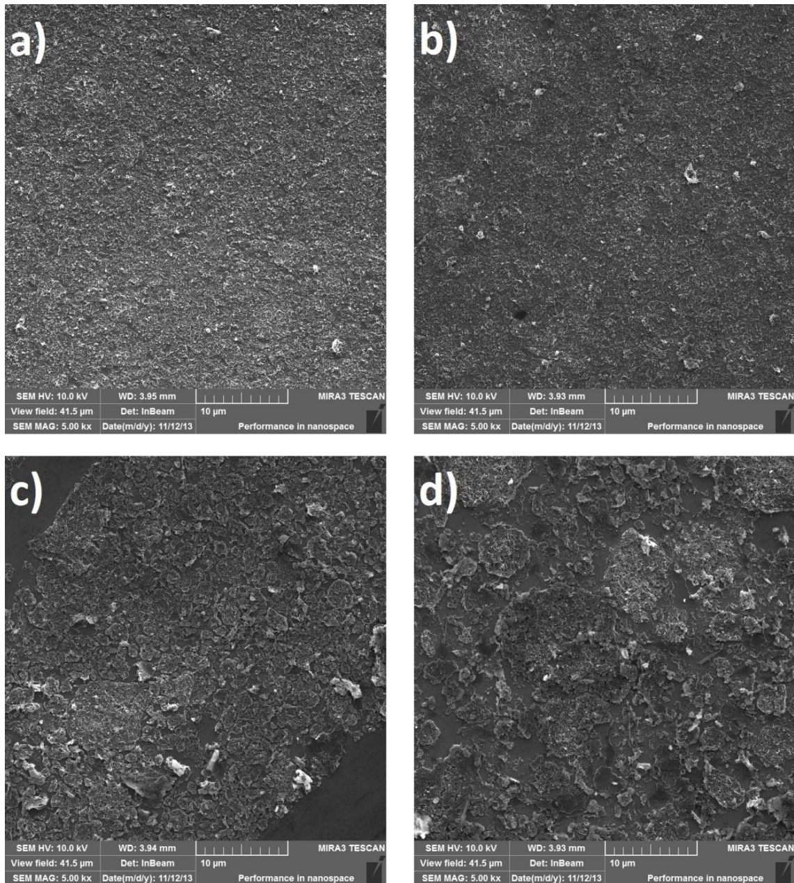
Figura 22 – Imagens dos filmes compostos de NTC/PANI (PANI sobre a forma base esmeraldina) a partir da técnica de microscopia eletrônica de varredura, com magnificação de 5000 vezes. a) Compósito 1/1. b) Compósito 1/3. c) Compósito 1/7. d) Compósito 1/10.
