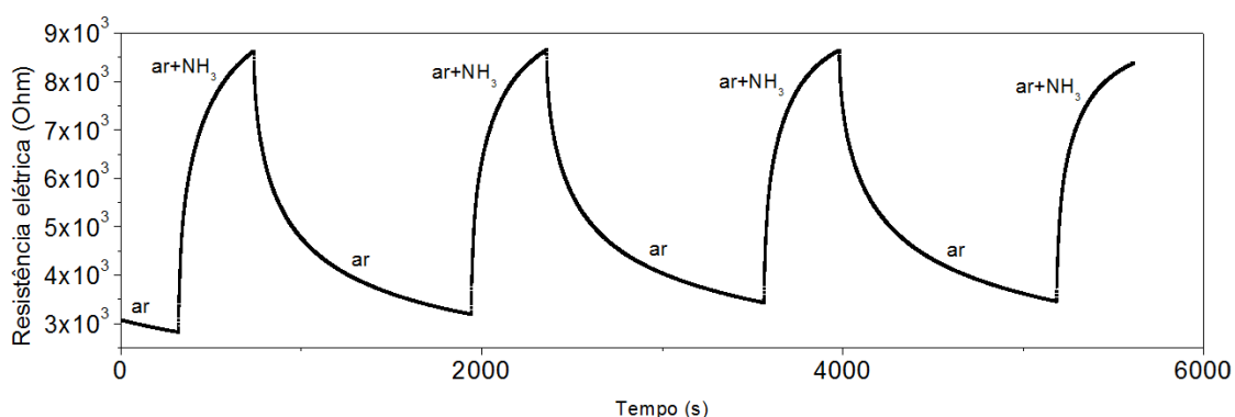
Figura 31 – Curvas de sensibilidade a 1000 PPM de \text{NH}_3 em ar para sensor com filme de camada ativa PANI, proporção 0/7 com dopagem primária de HCSA.
