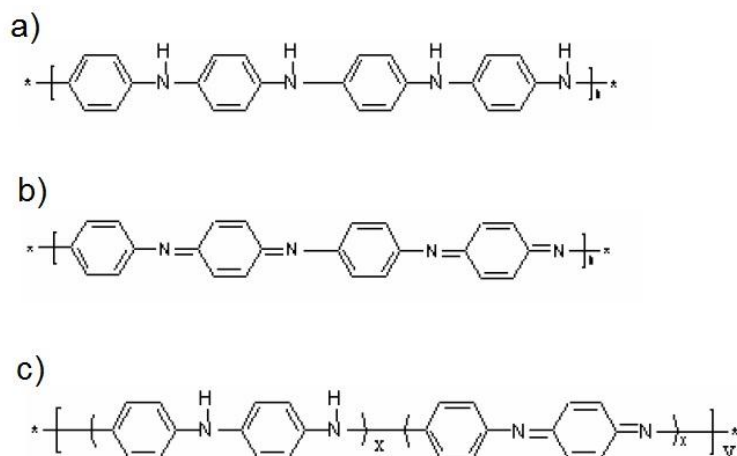
Figura 12 – a) Base Leucoesmeraldina. b) Base Pernigranilina. c) Base Esmeraldina. Adaptado de [54].
