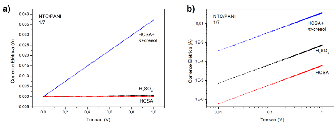
Figura 33 - (a) Comparativo IxV de dispositivos sensores com proporção NTC/PANI 1/7 e dopagem primária de H 2 SO 4 . (b) Comparativo log-log IxV para os mesmos dispositivos
