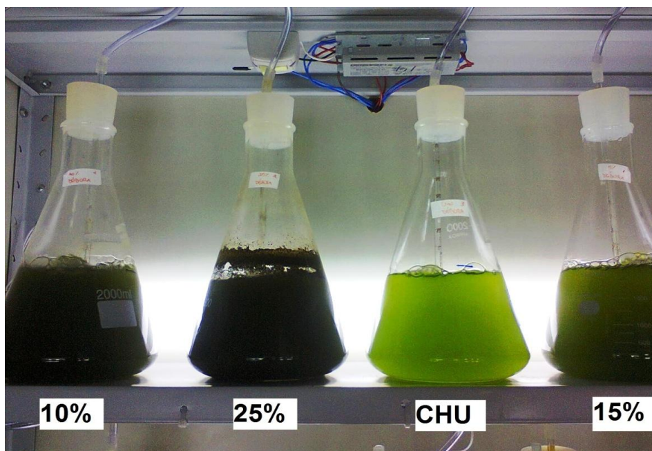
FIGURA 13 – DISPOSIÇÃO DOS FRASCOS PARA O EXPERIMENTO EM ESCALA LABORATORIAL
