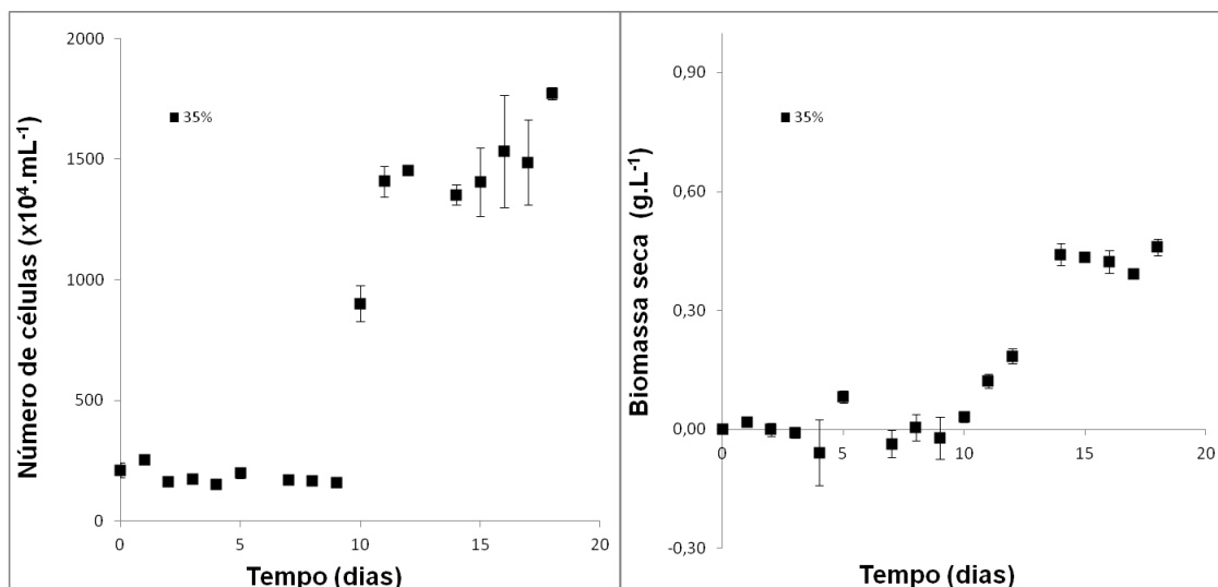
FIGURA 38 – ANÁLISES DE BIOMASSA SECA E NÚMERO DE CÉLULAS DA REPETIÇÃO DO CULTIVO COM 35% DE ESGOTO EM REATOR AIRLIFT
