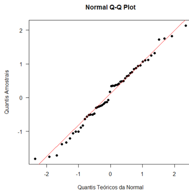
FIGURA 25 – GRÁFICO QUANTIL-QUANTIL PARA CRESCIMENTO CELULAR EM ESCALA LABORATORIAL
