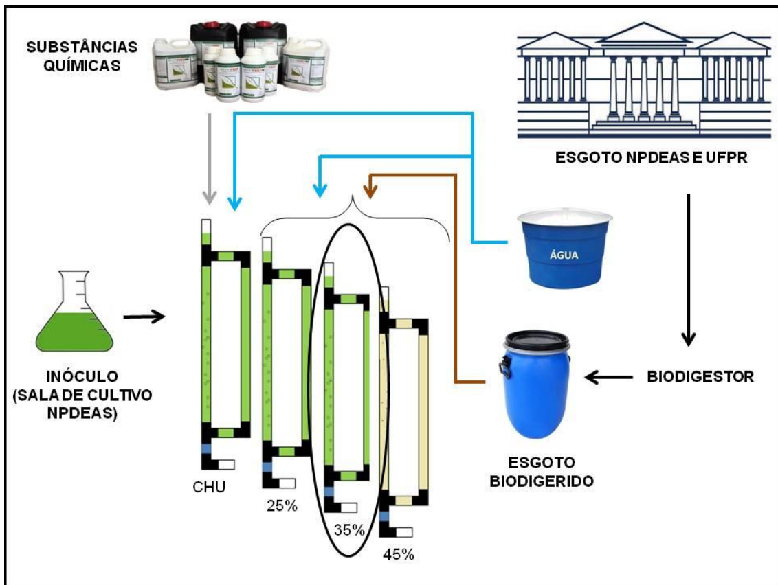
FIGURA 37 – FLUXOGRAMA DAS ATIVIDADES REALIZADAS EM REATOR AIRLIFT PARA DETERMINAÇÃO DA MELHOR CONDIÇÃO
