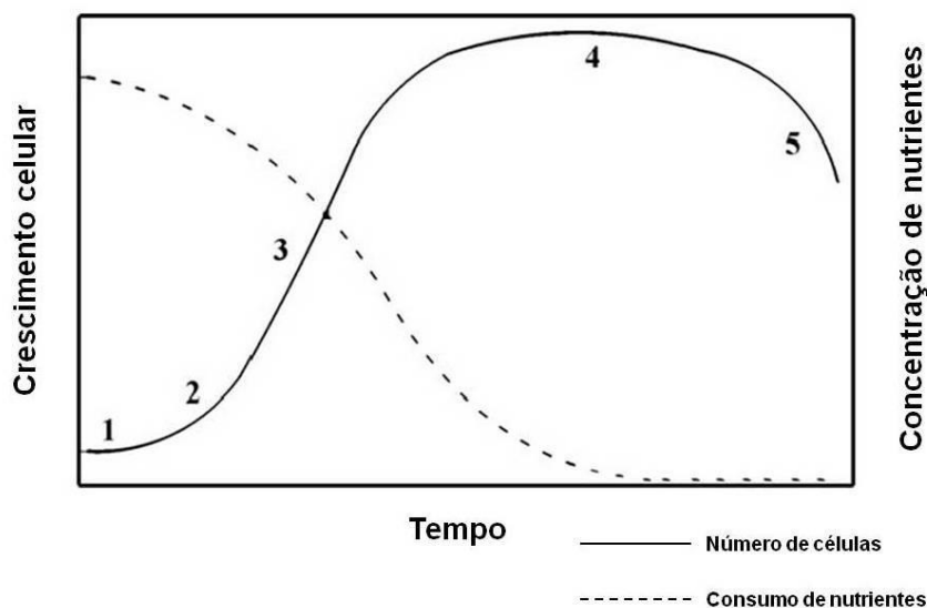
FIGURA 32 – CURVA TÍPICA DE CRESCIMENTO CELULAR. (1) FASE LAG, (2) FASE DE CRESCIMENTO EXPONENCIAL, (3) FASE DE CRESCIMENTO LINEAR, (4) FASE ESTACIONÁRIA, (5) FASE DE DECLÍNIO
