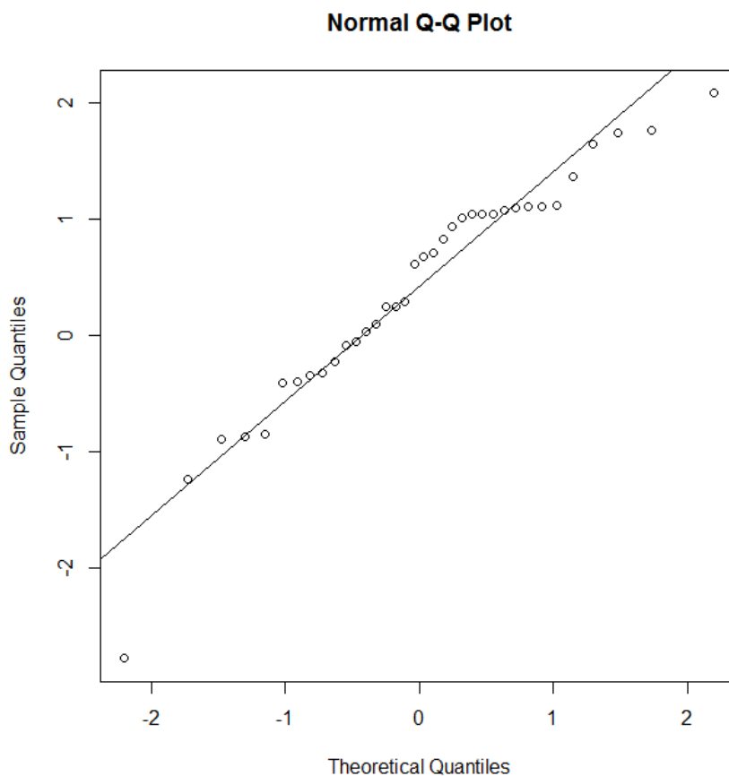
FIGURA 34 – GRÁFICO QUANTIL-QUANTIL PARA VARIÁVEL NÚMERO DE CÉLULAS EM REATOR AIRLIFT
