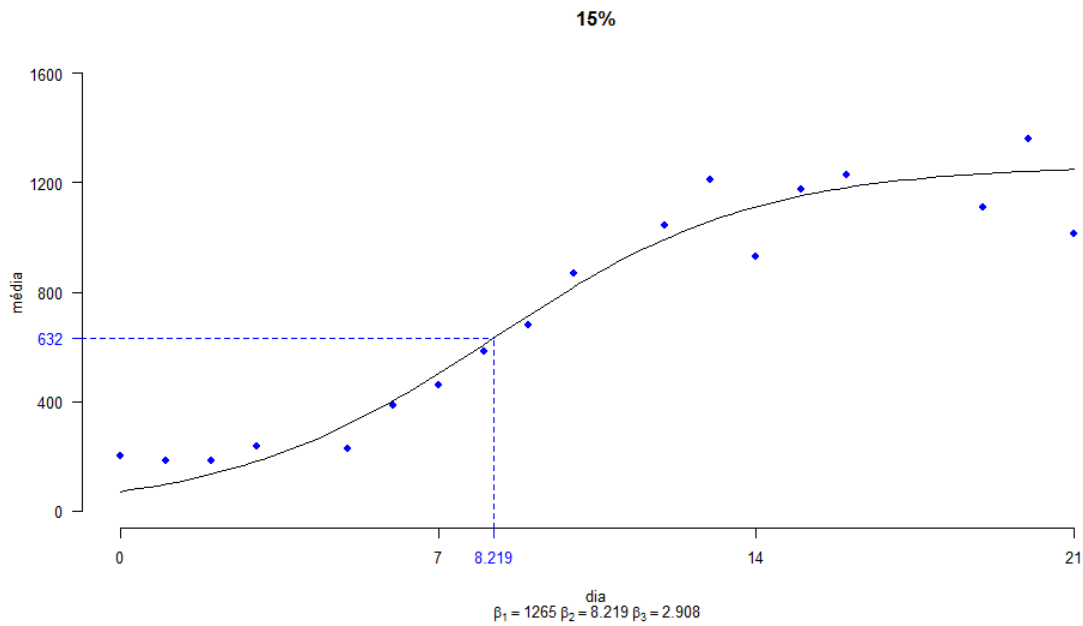
FIGURA 24 – CURVA DE AJUSTE LOGÍSTICO PARA OS DADOS DE CRESCIMENTO CELULAR DO CULTIVO COM 15% DE ESGOTO EM ESCALA LABORATORIAL
