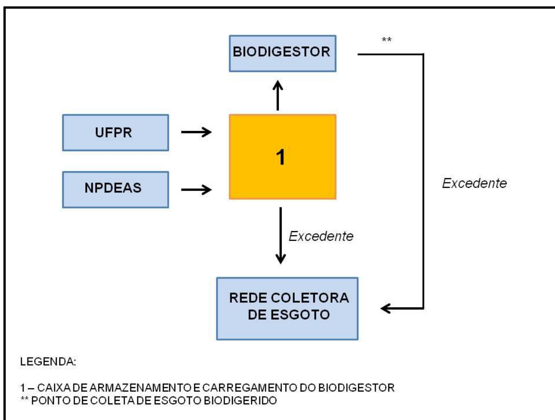
FIGURA 10 – FLUXOGRAMA COLETA E BIODIGESTÃO DO ESGOTO SANITÁRIO DA UFPR E DO NPDEAS
