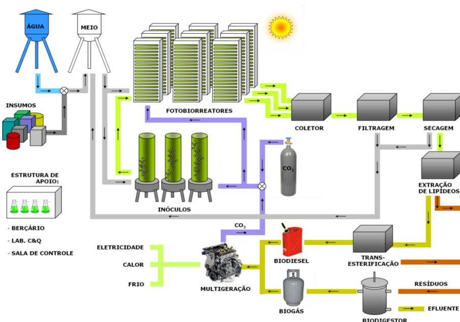
FIGURA 05 – FLUOXOGRAMA DAS ATIVIDADES REALIZADAS NO NPDEAS
