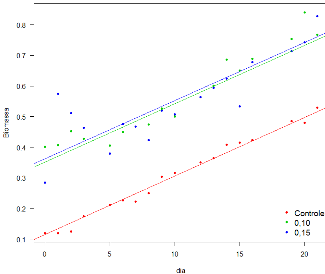
FIGURA 26 – AJUSTE LOGÍSTICO DE REGRESSÃO LINEAR PARA VARIÁVEL BIOMASSA EM ESCALA LABORATORIAL
