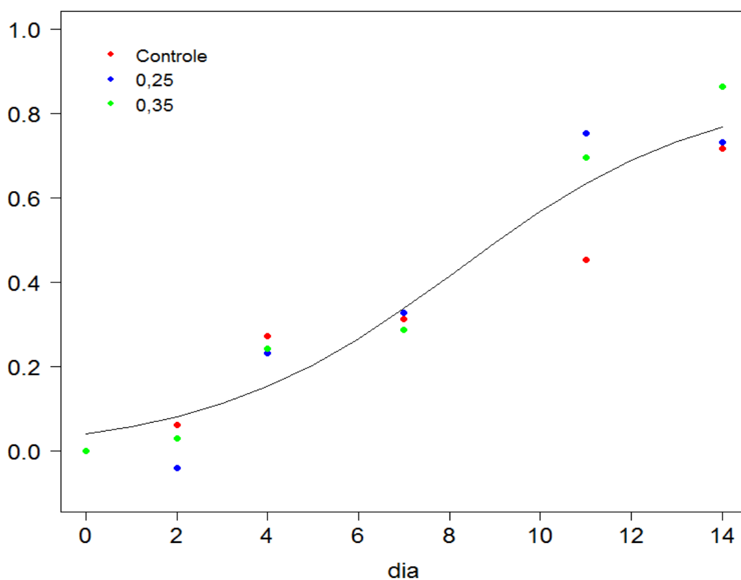
FIGURA 35 – CURVA DE AJUSTE LOGÍSTICO EXPLICANDO COMPORTAMENTO DA VARIÁVEL BIOMASSA SECA EM REATOR AIRLIFT
