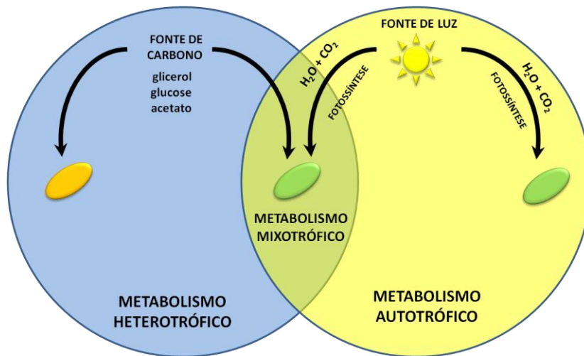
FIGURA 02 – ESQUEMA METABOLISMOS MICROALGAS.
