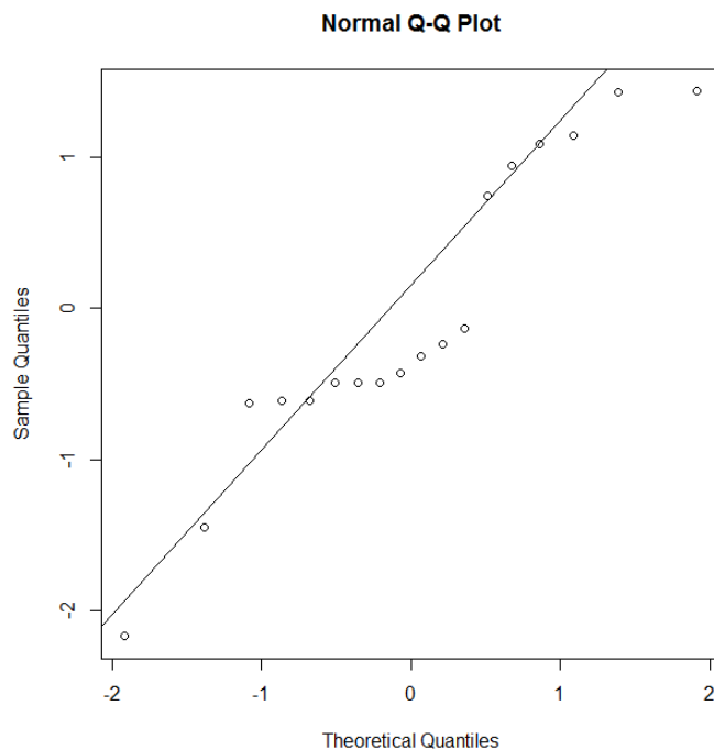
FIGURA 36 – GRÁFICO QUANTIL-QUANTIL PARA VARIÁVEL BIOMASSA EM REATOR AIRLIFT
