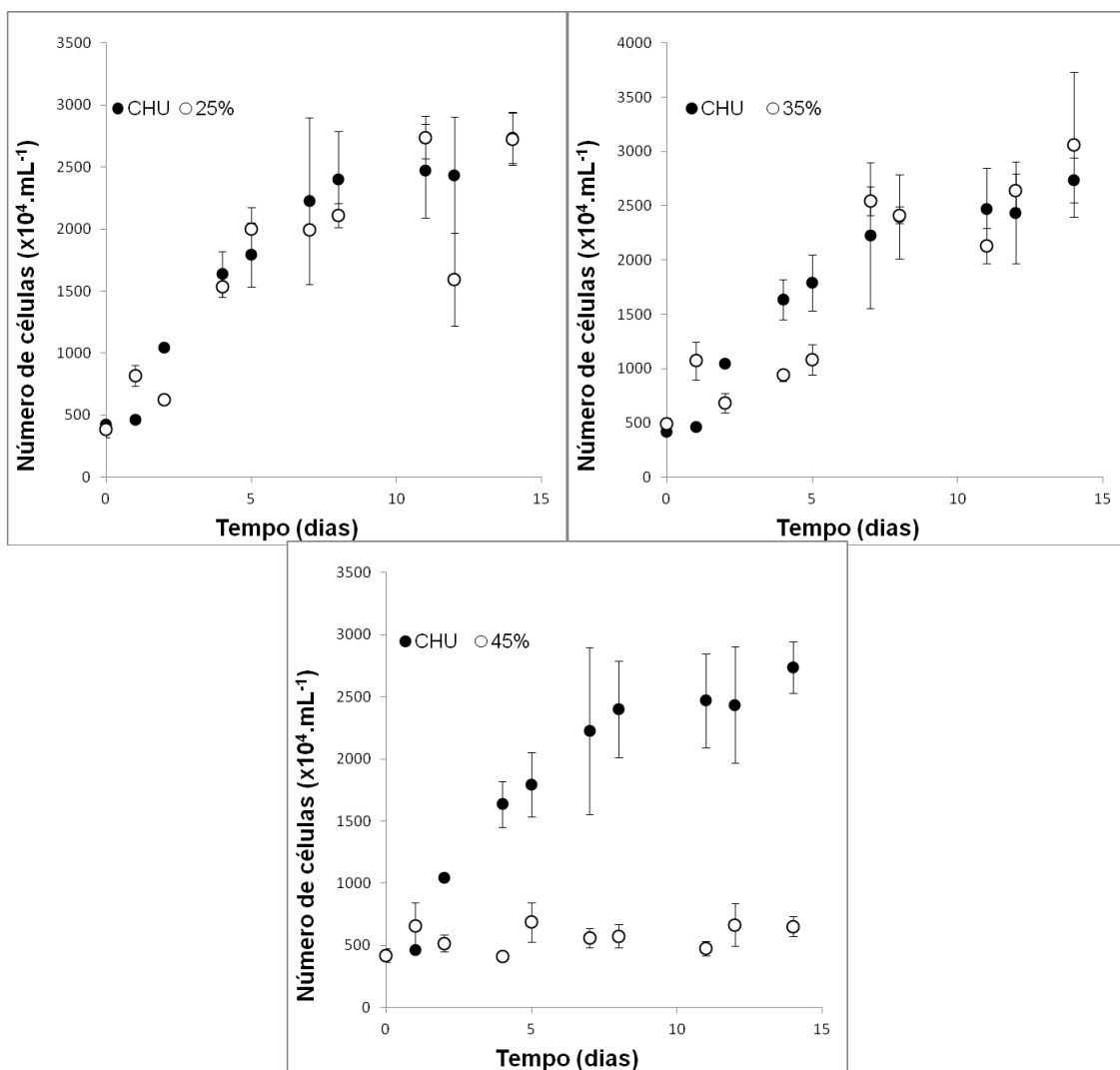
FIGURA 29 – NÚMERO DE CÉLULAS DOS TRATAMENTOS EM REATORES AIRLIFT COMPARADOS COM O CONTROLE (CHU)
