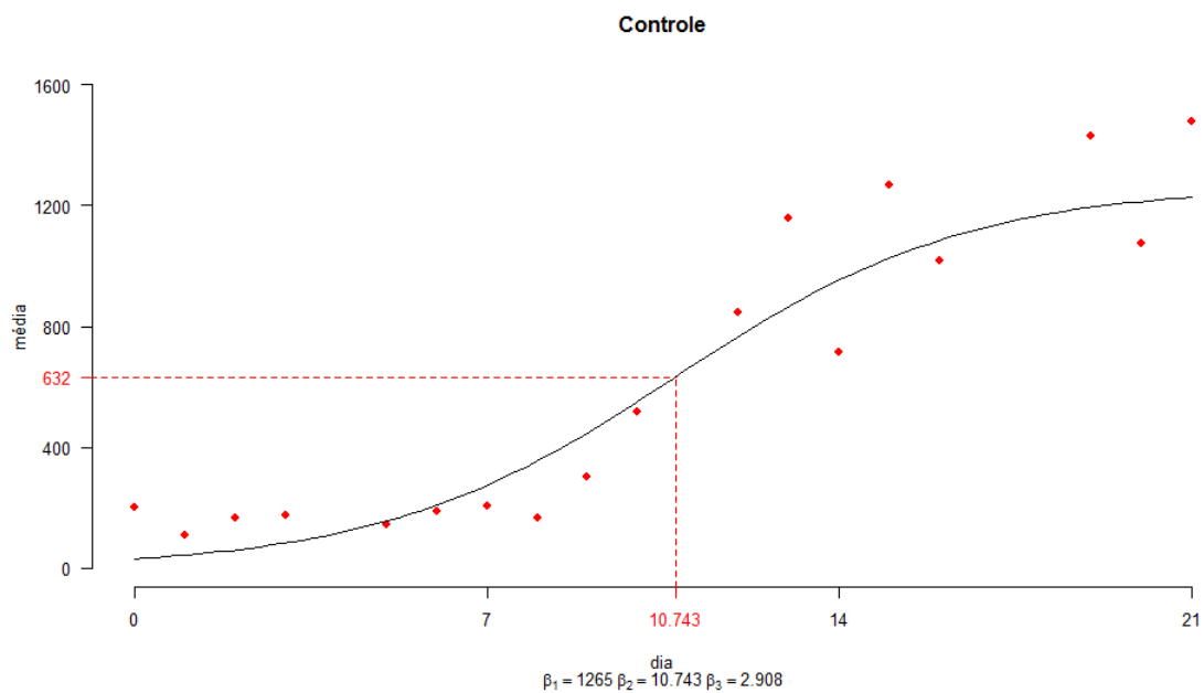
FIGURA 22 – CURVA DE AJUSTE LOGÍSTICO PARA OS DADOS DE CRESCIMENTO CELULAR DO CONTROLE (CHU) EM ESCALA LABORATORIAL
