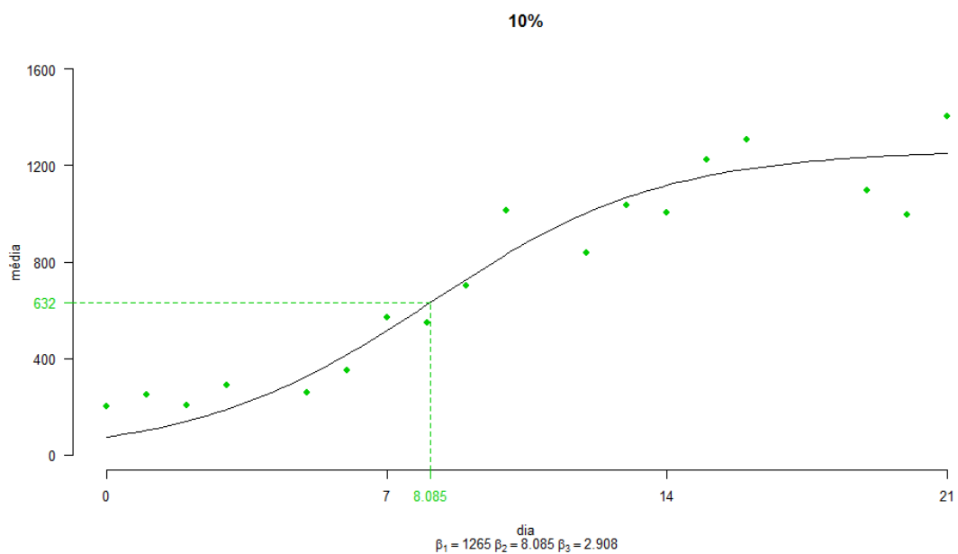
FIGURA 23 – CURVA DE AJUSTE LOGÍSTICO PARA OS DADOS DE CRESCIMENTO CELULAR DO CULTIVO COM 10% DE ESGOTO EM ESCALA LABORATORIAL
