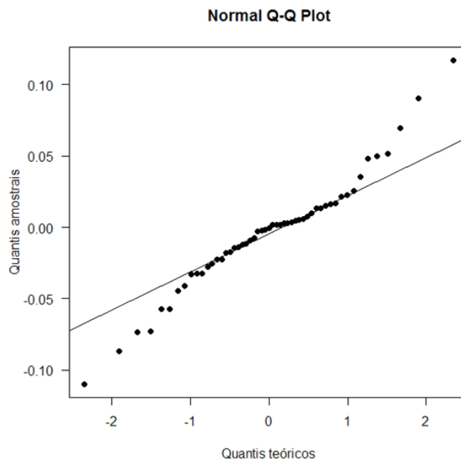
FIGURA 27 – GRÁFICO QUANTIL-QUANTIL PARA VARIÁVEL BIOMASSA EM ESCALA LABORATORIAL
