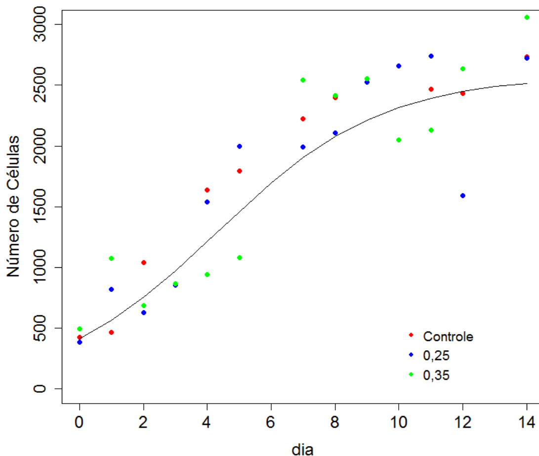
FIGURA 33 – CURVA DE AJUSTE LOGÍSTICO EXPLICANDO COMPORTAMENTO DA VARIÁVEL NÚMERO DE CÉLULAS EM REATOR AIRLIFT
