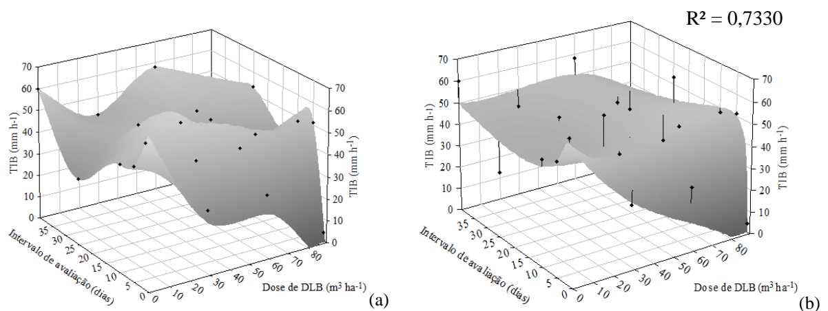
FIGURA 3. Superfície de resposta dos dados médios de Taxa de Infiltração Básica ( \text{mm h}^{-1} ): dados sem ajuste (a) e ajustados pela regressão do tipo z(x, y) (b).
