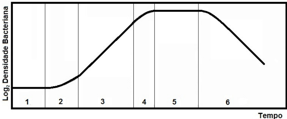
Figura 2. Fases do crescimento bacteriano, limitadas pelas retas verticais e identificadas pelo número das fases acima explicadas. O eixo y está em escala logarítmica e mostra a densidade bacteriana em cada fase. Fonte: adaptado de Monod (1949).
