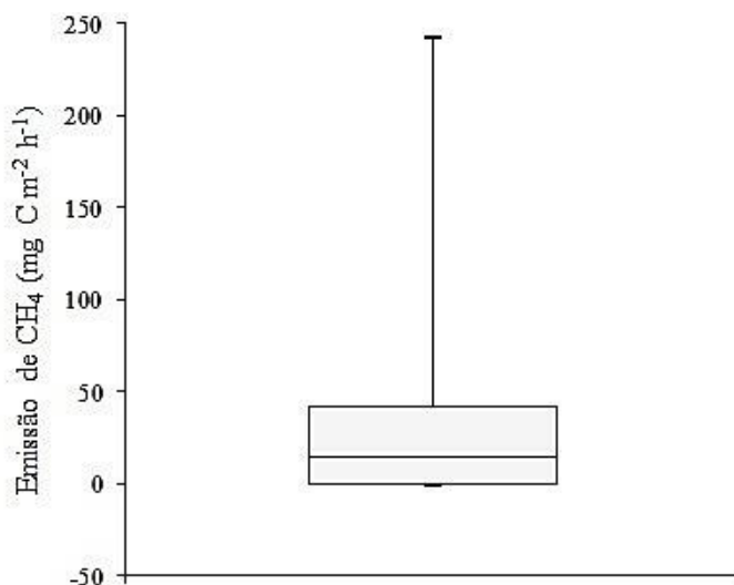
Figura 10. Box-plot dos dados de emissões de CH 4 ao longo de todo experimento.
