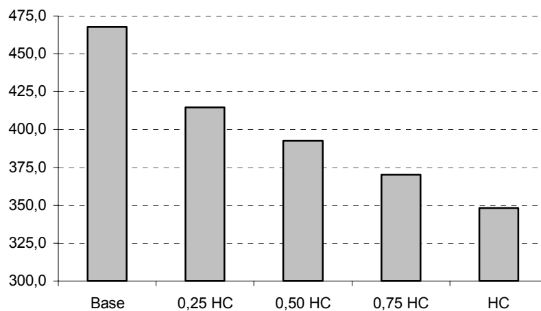
FIGURA 24 – TENDÊNCIA DE VARIAÇÃO DA MASSA ESPECÍFICA BÁSICA NAS POSIÇÕES RELATIVAS AO LONGO DO FUSTE PARA TODAS AS ÁRVORES AMOSTRADAS.
