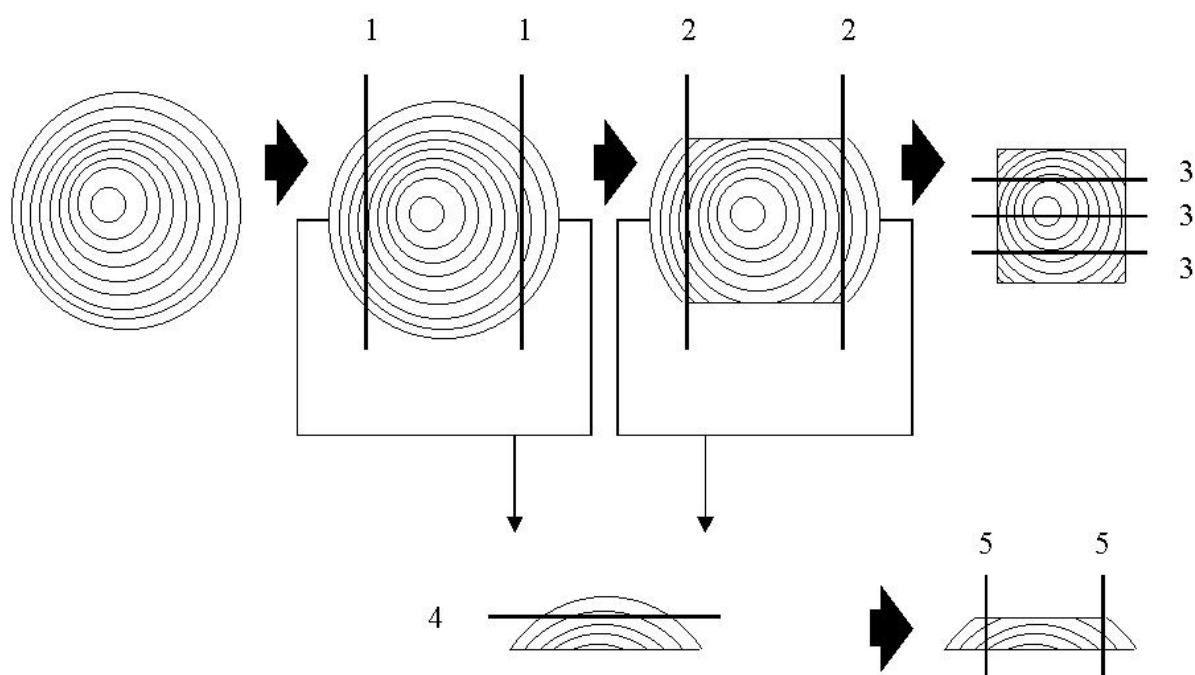
FIGURA 18 –SISTEMA DE DESDOBRÓ UTILIZADO.
