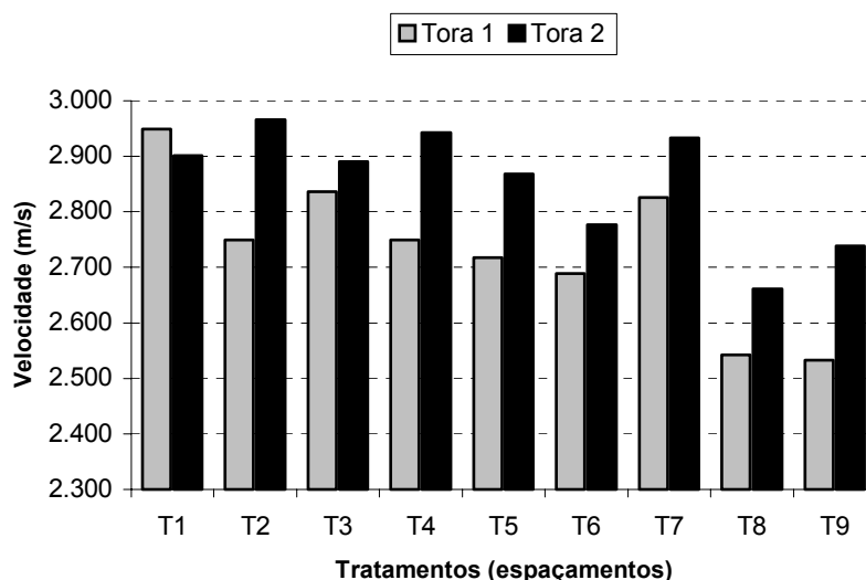
FIGURA 42 – TENDÊNCIA DE VARIAÇÃO DA VELOCIDADE DE PROPAGAÇÃO DAS ONDAS DE TENSÃO ENTRE AS POSIÇÕES DAS TORAS
