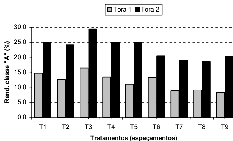
FIGURA 37 – VARIAÇÃO DOS RENDIMENTOS OBTIDOS NA CLASSE DE QUALIDADE “A” PARA DIFERENTES POSIÇÕES DAS TORAS ENTRE OS ESPAÇAMENTOS.
