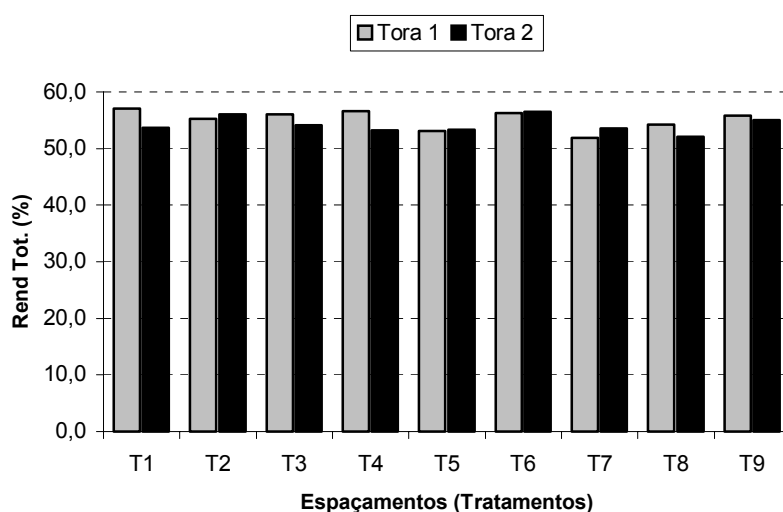
FIGURA 35 – RENDIMENTO TOTAL DETERMINADO PARA OS ESPAÇAMENTOS E POSIÇÕES DAS TORAS.
