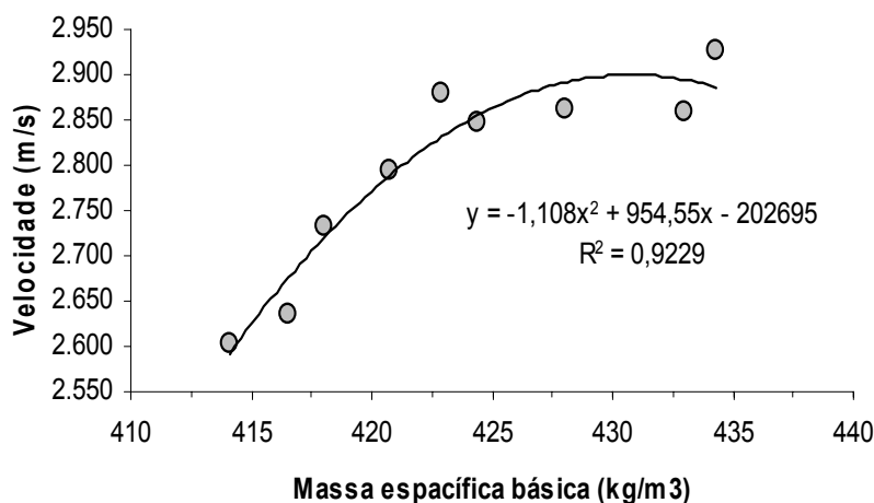
FIGURA 44 – TENDÊNCIA DE VARIAÇÃO DA VELOCIDADE MÉDIA DE PROPAGAÇÃO DAS ONDAS DE TENSÃO EM RELAÇÃO A MASSA ESPECÍFICA BÁSICA.
