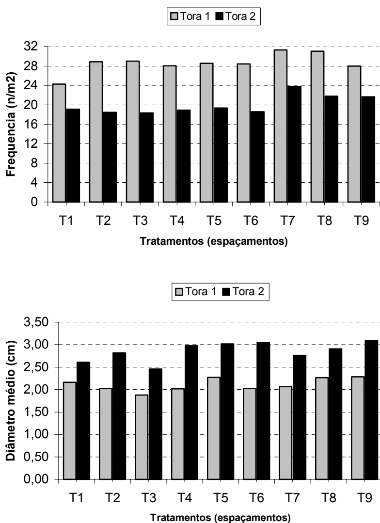
FIGURA 33 –VARIAÇÃO DA FREQUÊNCIA E DO DIÂMETRO DOS NÓS PARA DIFERENTES POSIÇÕES DAS TORAS ENTRE OS DIFERENTES ESPAÇAMENTOS.
