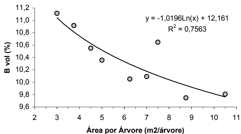
FIGURA 27 – TENDÊNCIA DE VARIAÇÃO DA PROPRIEDADE DE CONTRAÇÃO MÁXIMA TANGENCIAL DAS AMOSTRAS AVALIADAS PARA OS ESPAÇAMENTOS ESTUDADOS.
