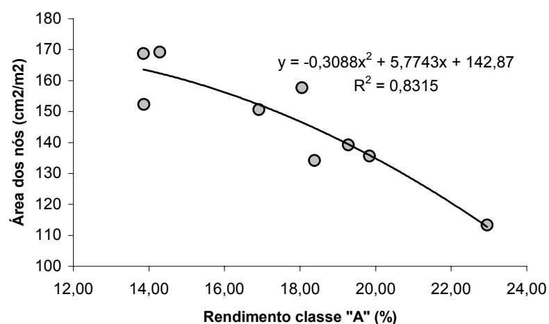
FIGURA 39 – TENDÊNCIA DE VARIAÇÃO DOS RENDIMENTOS OBTIDOS NA CLASSE DE QUALIDADE “A” EM FUNÇÃO DA ÁREA DOS NÓS.
