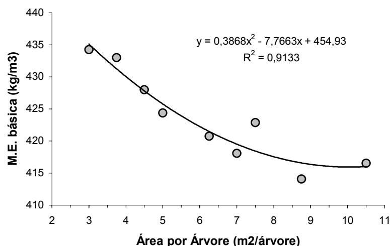
FIGURA 23 – TENDÊNCIA DE VARIAÇÃO DA MASSA ESPECÍFICA BÁSICA PONDERADA DAS ÁRVORES AMOSTRADAS NOS ESPAÇAMENTOS ESTUDADOS.
