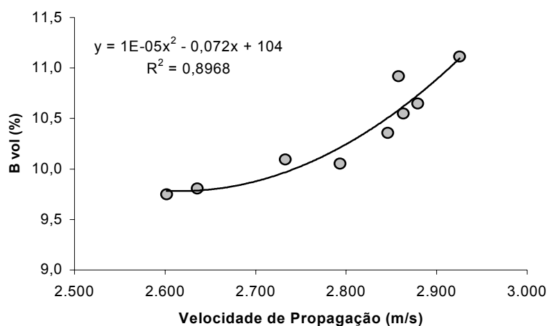
FIGURA 45 – TENDÊNCIA DE VARIAÇÃO DA VELOCIDADE MÉDIA DE PROPAGAÇÃO DAS ONDAS DE TENSÃO EM RELAÇÃO AS CONTRAÇÕES MÁXIMAS VOLUMÉTRICA E LINEARES DA MADEIRA.
