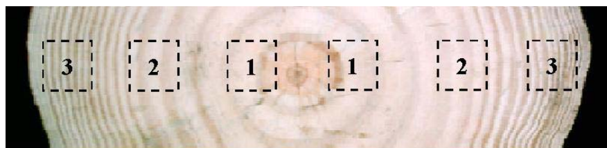
FIGURA 12 – POSIÇÃO DA RETIRADA DOS CORPOS DE PROVA NA SEÇÃO TRANSVERSAL DA TORA.
