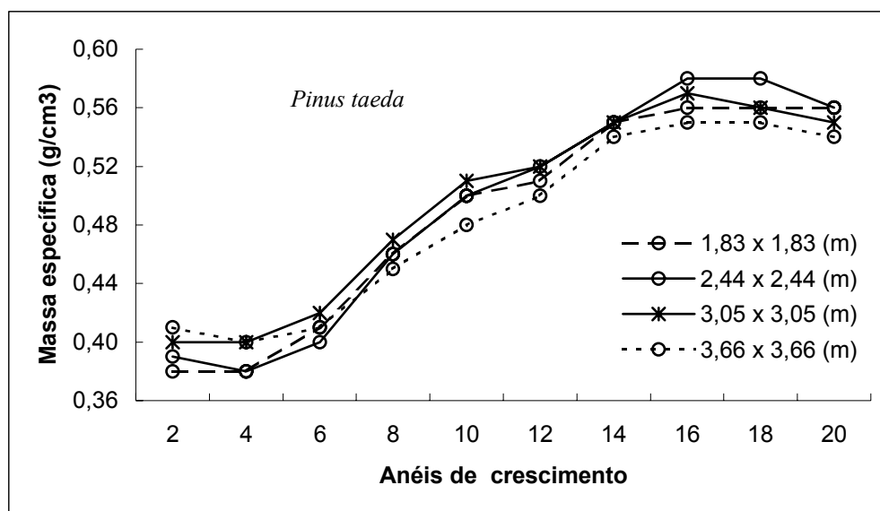
FIGURA 03 – COMPORTAMENTO DA MASSA ESPECÍFICA COM O AUMENTO DA IDADE NOS DIFERENTES ESPAÇAMENTOS PARA PINUS TAEDA .
