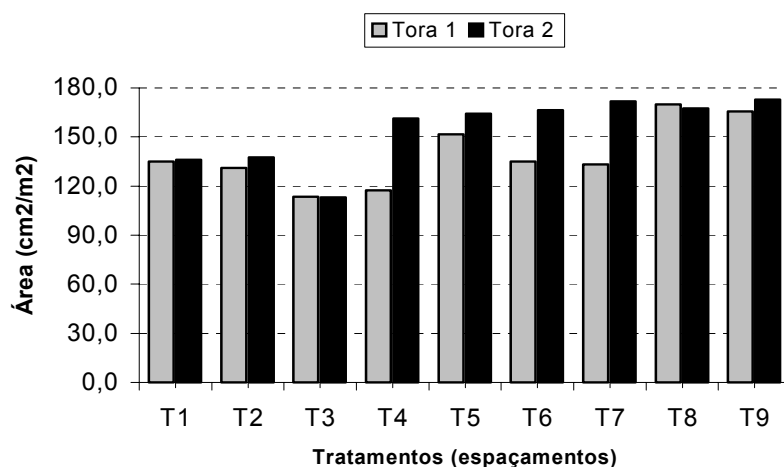
FIGURA 34 –VARIAÇÃO DA ÁREA DOS NÓS PARA DIFERENTES POSIÇÕES DAS TORAS ENTRE OS DIFERENTES ESPAÇAMENTOS.
