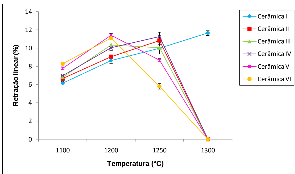
Figura 17 – Variação da retração linear (RL) em função das temperaturas de queima para as cerâmicas investigadas.
