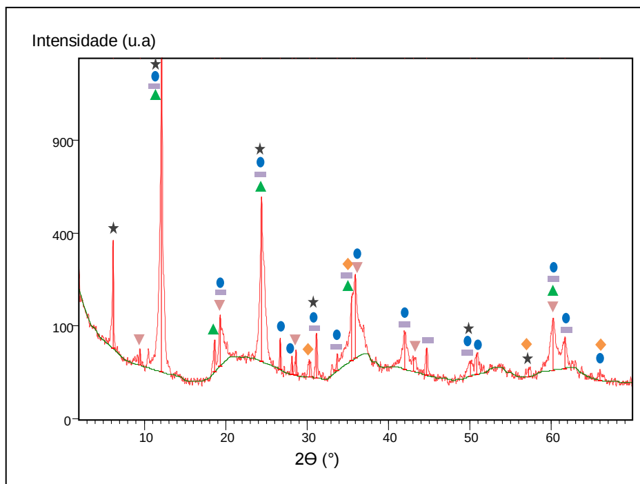
Figura 5 – Difratoograma do resíduo da mineração de serpentinito.
