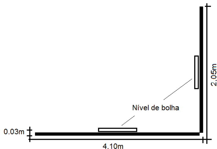
Figura 3.5: Calibrador bidimensional.
