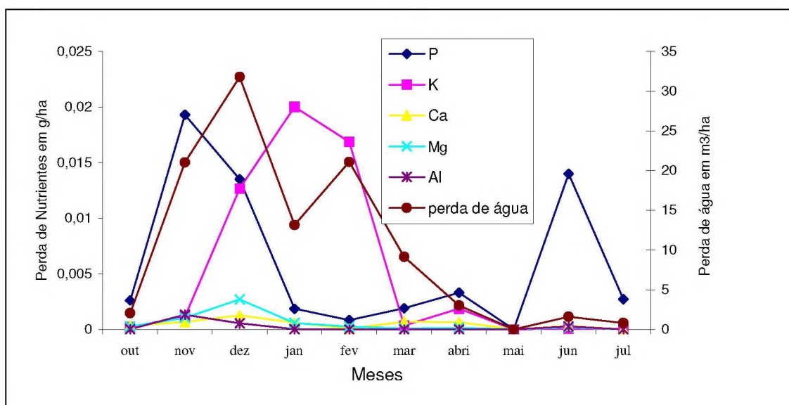
GRÁFICO 6 - PERDAS DE NUTRIENTES EM g/ha E ÁGUA EM m 3 /ha POR EROSÃO EM SOLUÇÃO NO TRATAMENTO 3 , NO PERÍODO 2002-2003
