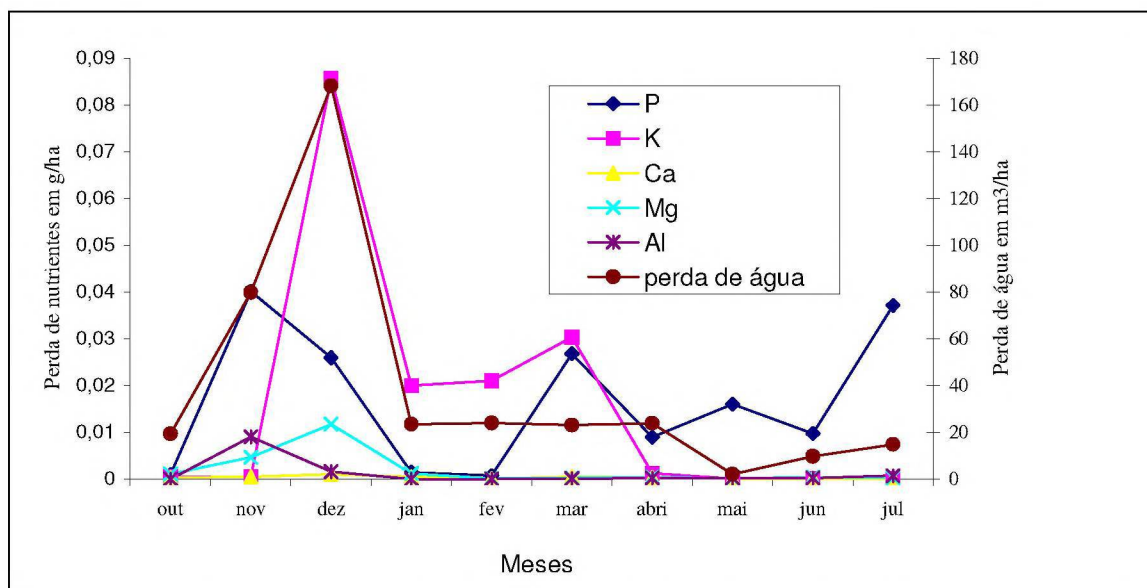
GRÁFICO 7 - PERDAS DE NUTRIENTES g/ha E ÁGUA m 3 /ha POR EROSIÃO EM SOLUÇÃO NO TRATAMENTO 4, NO PERÍODO 2002-2003
