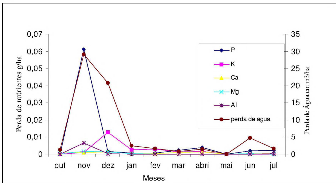
GRÁFICO 5 - PERDAS DE NUTRIENTES EM g/ha E ÁGUA EM m 3 /ha POR EROSÃO EM SOLUÇÃO NO TRATAMENTO 1 , NO PERÍODO 2002-2003
