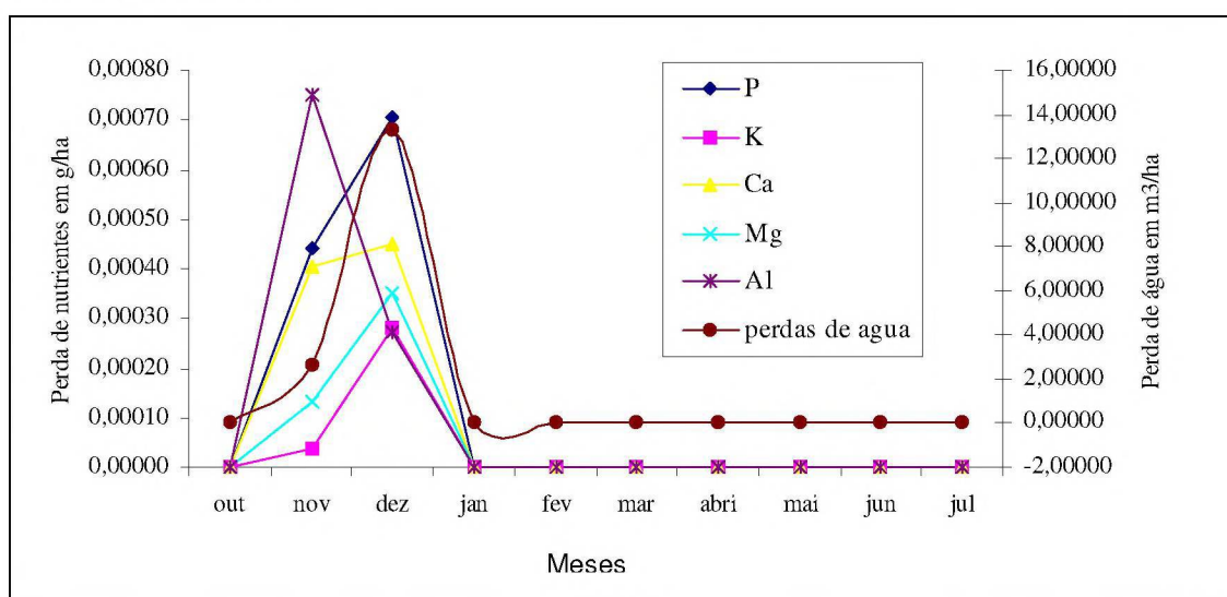
GRÁFICO 8 - PERDAS DE NUTRIENTES EM g/ha E ÁGUA EM m³/ha POR EROSIÃO EM SOLUÇÃO NO TRATAMENTO 2, NO PERÍODO 2002-2003
