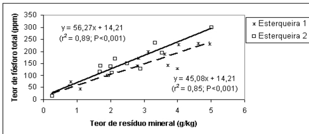
FIGURA 2 - PREDIÇÃO DO TEOR DE FÓSFORO A PARTIR DO TEOR DE RESÍDUO MINERAL EM AMOSTRAS DE EFLUENTES, DADOS COM BASE NA MATÉRIA SECA
