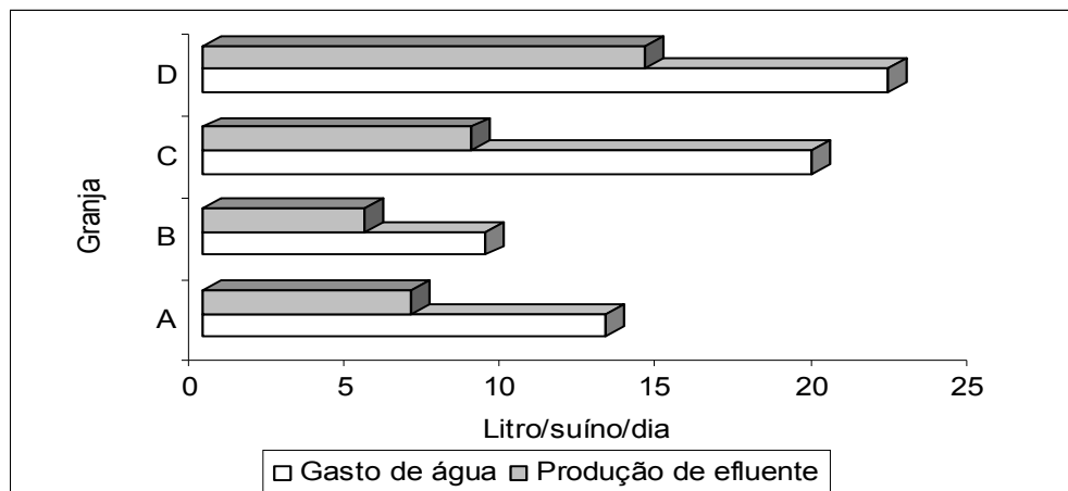
FIGURA 3 - GASTO DE ÁGUA E VOLUME DE EFLUENTE (L/SUÍNO/DIA)
