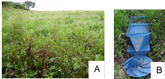
FOTO 2: A - USO E COBERTURA DO SOLO NA ENCOSTA SOB SISTEMA CONVENCIONAL, B - ASPECTO DA RODA DE COSCHOCTON EM 07 DE DEZ DE 2007.
