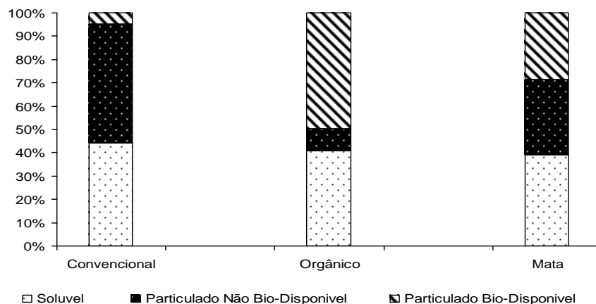
FIGURA 2.1 – PERCENTUAL DE PERDA ANUAL DE FÓSFORO EM SUAS DIFERENTES FORMAS NA ÁGUA DO ESCOAMENTO SUPERFICIAL NOS DIFERENTES SISTEMAS
