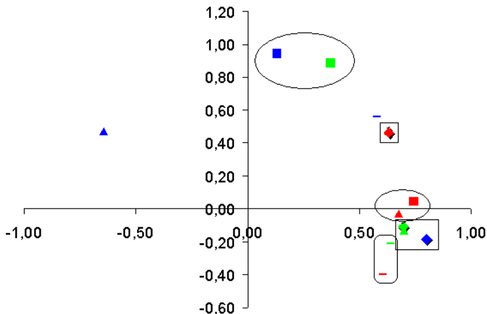
FIGURA 1.2 - ANÁLISE DE COMPONENTES PRINCIPAIS DOS ATRIBUTOS FÍSICOS DO SOLO NOS DIFERENTES SISTEMAS DE CULTIVO E NAS TRÊS PROFUNDIDADES DE ACORDO COM A LEGENDA APRESENTADA ACIMA, NA BACIA HIDROGRÁFICA DO RIO CAMPESTRE, COLOMBO, PR
