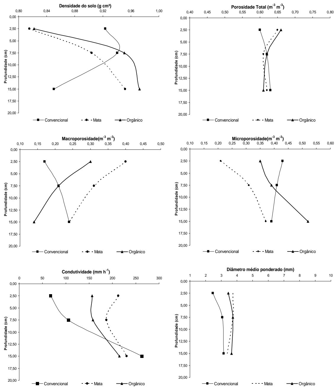
FIGURA 1.1 – ATRIBUTOS FÍSICOS DO SOLO NA PROFUNDIDADE DE 0-20 cm DAS ENCOSTAS SOB DIFERENTES SISTEMAS, NA BACIA HIDROGRÁFICA DO RIO CAMPESTRE, COLOMBO, PR
