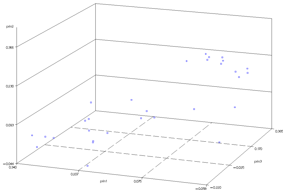
FIGURA 2.3 – GRÁFICO GERADO APARTIR DO PROGRAMA ESTATÍSTICO: SAS VERSÃO 8.2. ANÁLISE DE COMPONENTES PRINCIPAIS DAS CONCENTRAÇÕES DE NUTRIENTES NOS DIFERENTES SISTEMAS ESTUDADOS
