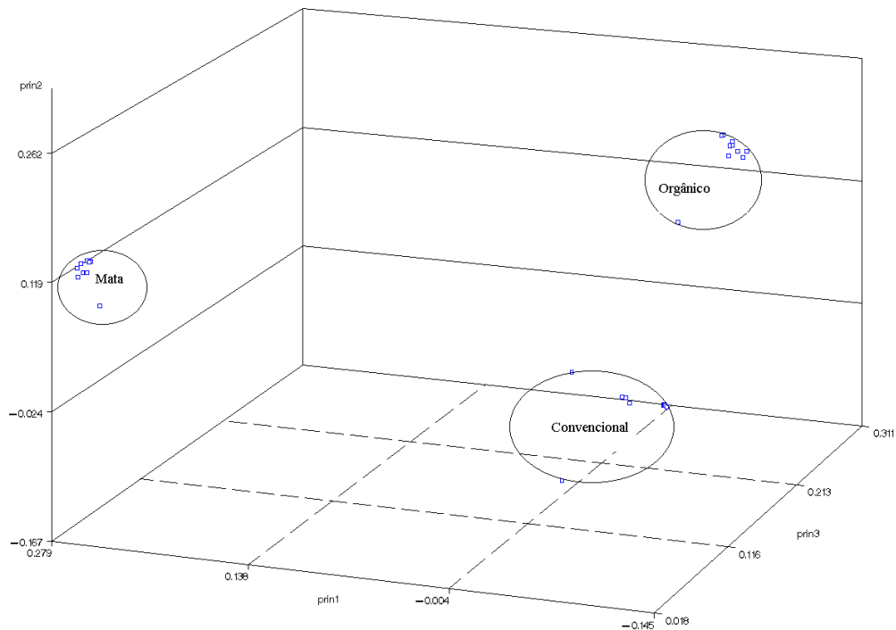
FIGURA 2.4 – GRÁFICO GERADO APARTIR DO PROGRAMA ESTATÍSTICO: SAS VERSÃO 8.2. ANÁLISE DE COMPONENTES PRINCIPAIS DAS PERDAS DE NUTRIENTES NOS DIFERENTES SISTEMAS ESTUDADOS
