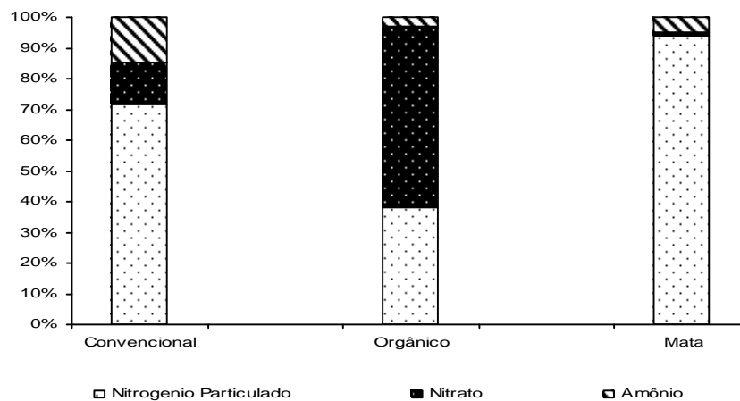
FIGURA 2.2 – PERCENTUAL DE PERDA ANUAL DE NITROGÊNIO POR ENCOSTA, NAS SUAS DIFERENTES FORMAS NA ÁGUA DO ESCOAMENTO SUPERFICIAL NOS DIFERENTES SISTEMAS
