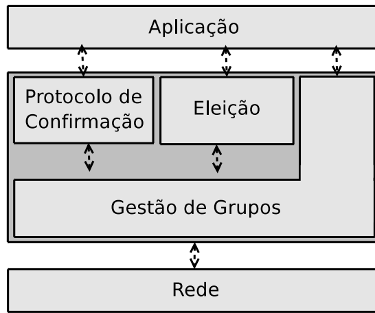
Figura 4.1: Estrutura em módulos da ferramenta.
