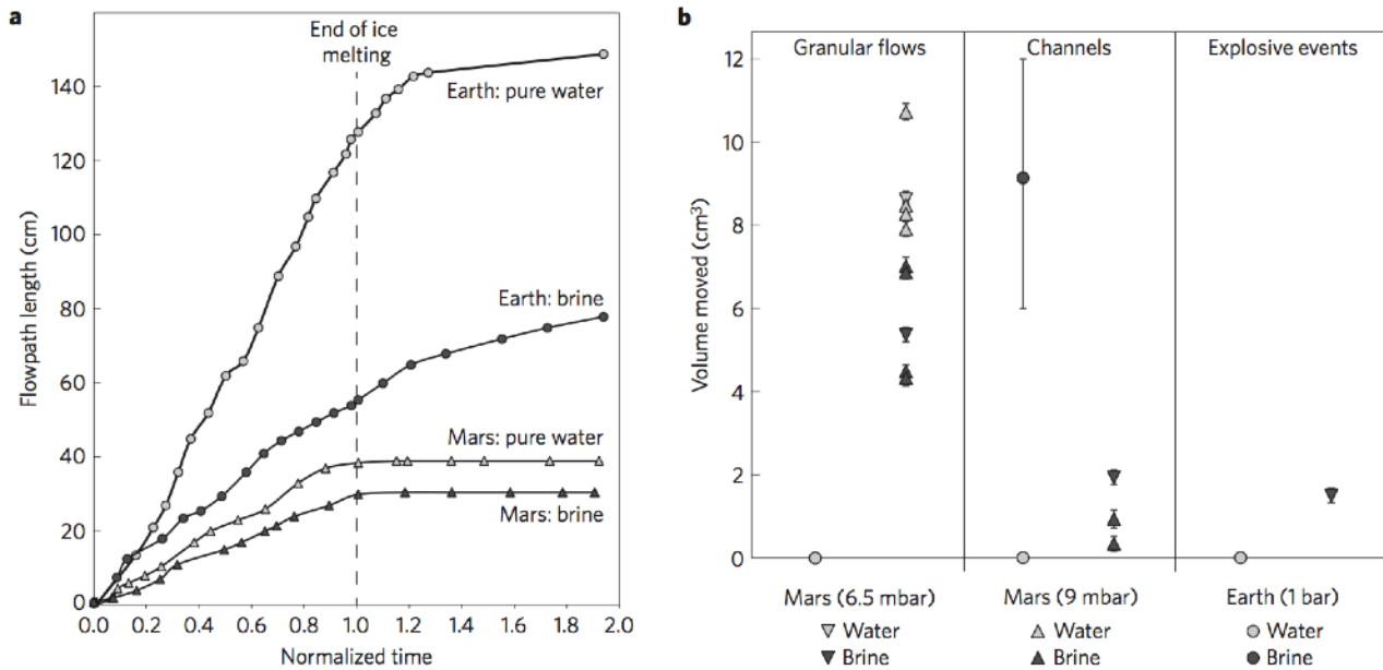
Figura 27 - a) Evolução das dimensões das feições geradas pelo fluxo com o tempo para os experimentos retratados na Fig. 26 (tempo normalizado pela duração total do derretimento do gelo). b) Volume de sedimentos movidos pelos experimentos, para diferentes condições ambientais. Fonte: Massé et al. (2016).
