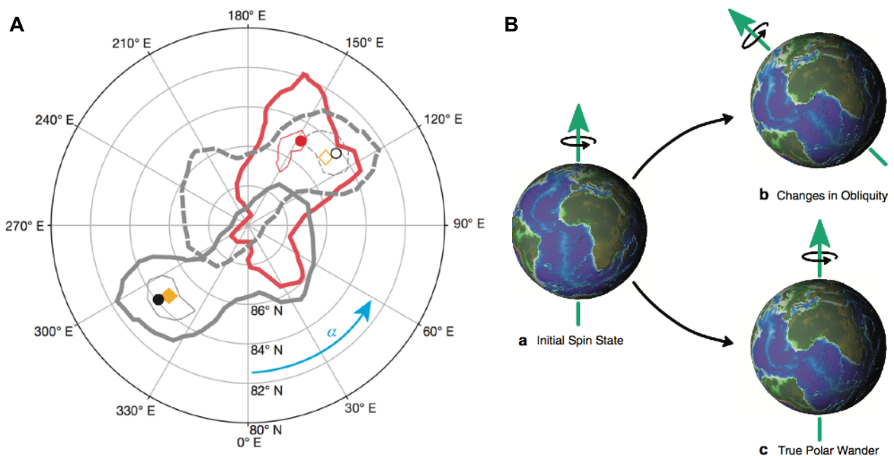
Figura 16 - A) Contornos de concentração de hidrogênio para 75ppm (linhas finas) e 100ppm (linhas grossas) nos pólos norte (em vermelho) e sul (em cinza). Os círculos vermelho e preto mostram os máximos da concentração de hidrogênio nos pólos norte e sul respectivamente. O diamante laranja mostra o local de impacto da LCROSS. As formas sem preenchimento são projeções no pólo norte. B) Ilustração de dois modos de reorientação planetária: mudança na obliquidade (b) e TPW (c).
