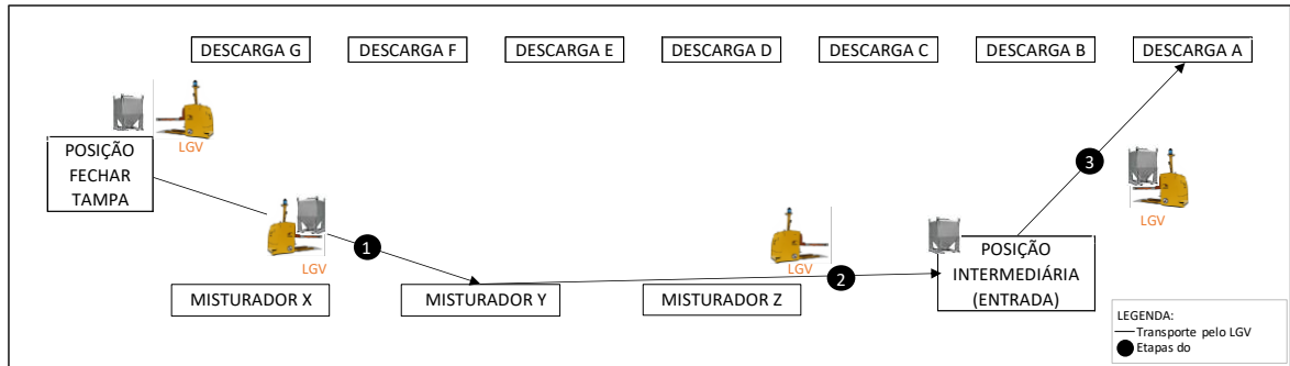
FIGURA 22 - FLUXO DO PROCESSO COM AÇÃO RETARDATÁRIA
