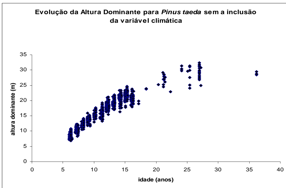
FIGURA 12 – EVOLUÇÃO DA ALTURA DOMINANTE SEM A INCLUSÃO DA VARIÁVEL CLIMÁTICA
