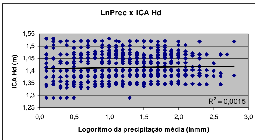
FIGURA 8 - RELAÇÃO ENTRE O LOGARITMO NATURAL DA PRECIPITAÇÃO MÉDIA E O INCREMENTO CORRENTE ANUAL EM ALTURA DOMINANTE
