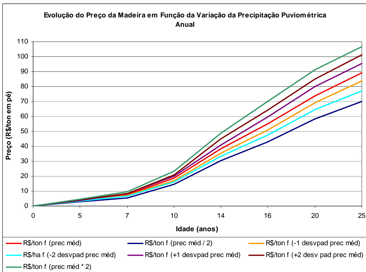
FIGURA 18 – EVOLUÇÃO DO RECEITA POTENCIAL DA MADEIRA EM PÉ EM REAIS POR TONELADA EM FUNÇÃO DA VARIAÇÃO DA PRECIPITAÇÃO PLUVIOMÉTRICA ANUAL
