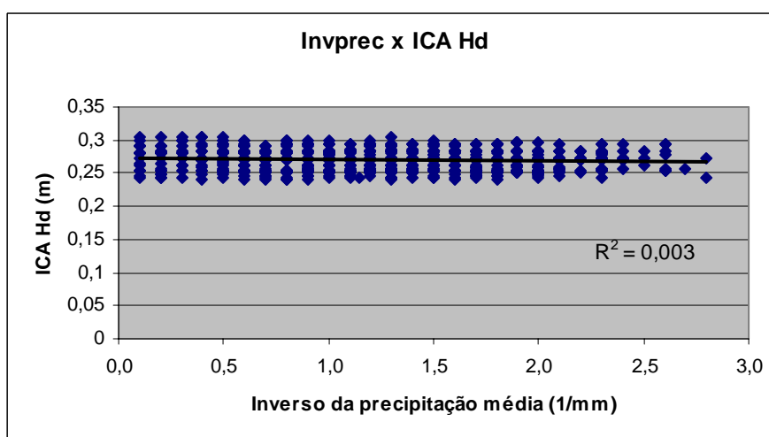
FIGURA 9 - RELAÇÃO ENTRE O INVERSO DA PRECIPITAÇÃO MÉDIA E O INCREMENTO CORRENTE ANUAL EM ALTURA DOMINANTE
