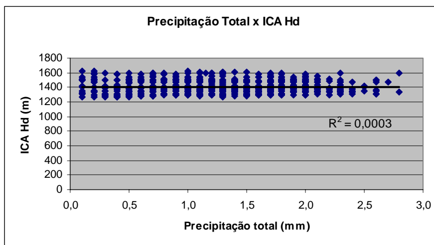
FIGURA 7 - RELAÇÃO ENTRE A PRECIPITAÇÃO TOTAL E O INCREMENTO CORRENTE ANUAL EM ALTURA DOMINANTE
