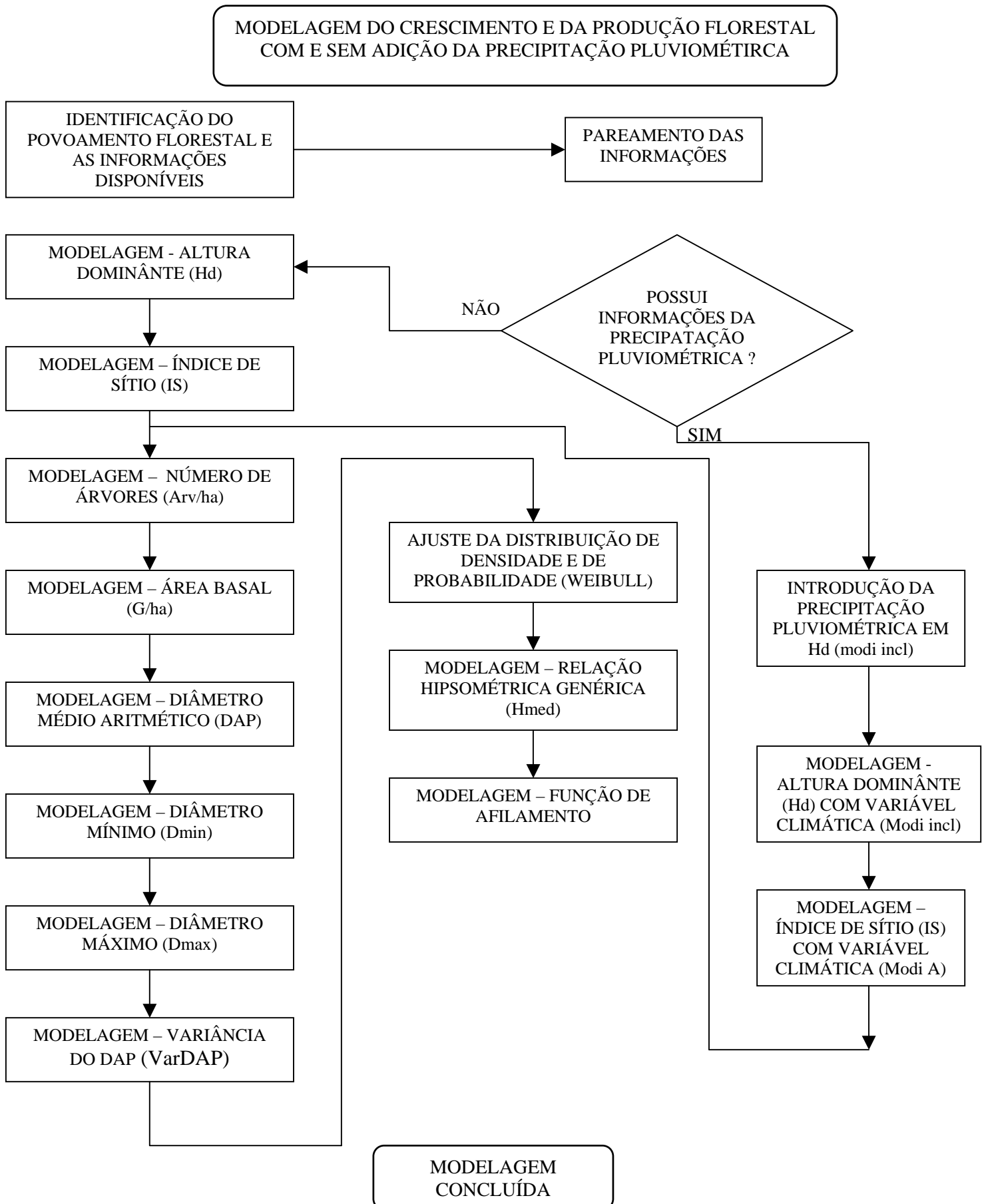
FIGURA 15 – FLUXOGRAMA DA MODELAGEM DO CRESCIMENTO E DA PRODUÇÃO FLORESTAL COM E SEM A ADIÇÃO DA PRECIPITAÇÃO PLUVIOMÉTRICA
