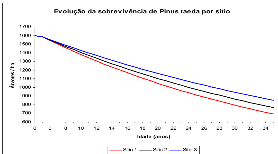
FIGURA 14 - EVOLUÇÃO DA SOBREVIVÊNCIA DE PINUS TAEDA POR SÍTIO
