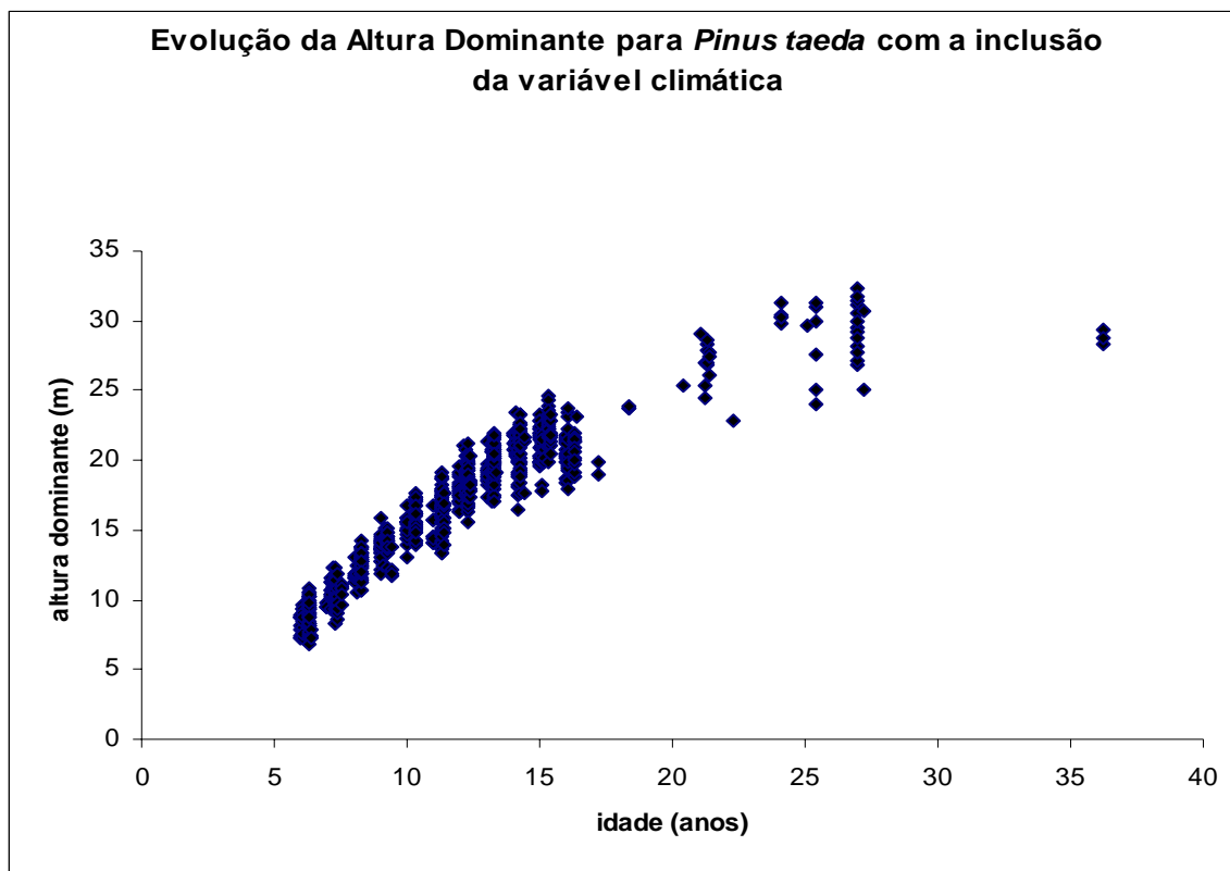
FIGURA 13 – EVOLUÇÃO DA ALTURA DOMINANTE COM A INCLUSÃO DA VARIÁVEL CLIMÁTICA
