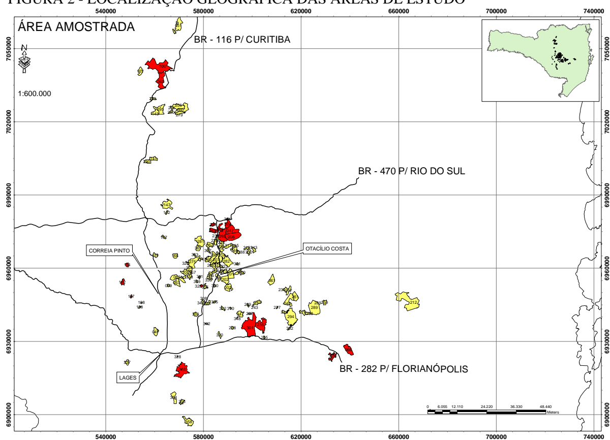
FIGURA 2 - LOCALIZAÇÃO GEOGRÁFICA DAS ÁREAS DE ESTUDO
