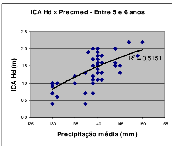
FIGURA 11 - RELAÇÃO ENTRE A PRECIPITAÇÃO MÉDIA E O INCREMENTO CORRENTE ANUAL EM ALTURA DOMINANTE EM DIFERENTES IDADES
