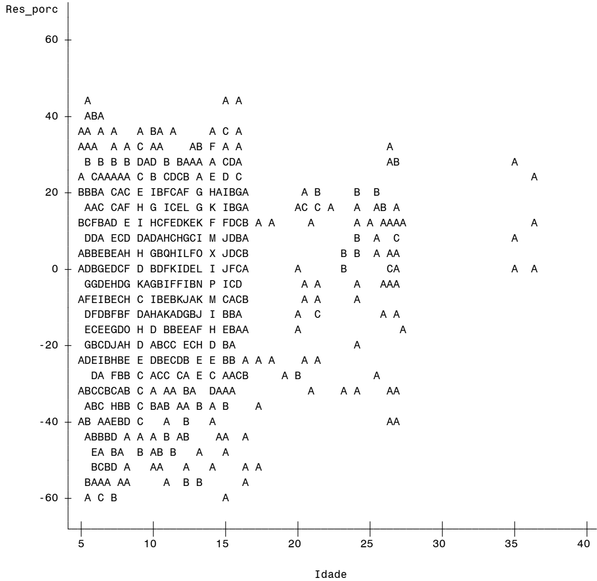
Plot of Res_porc*Idade. Legend: A = 1 obs, B = 2 obs, etc.
