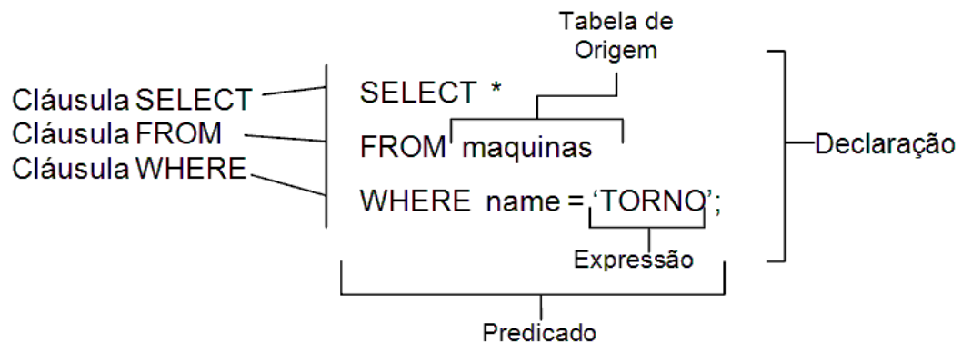
ILUSTRAÇÃO 2 - Exemplo da sentença "SELECT" da linguagem SQL
