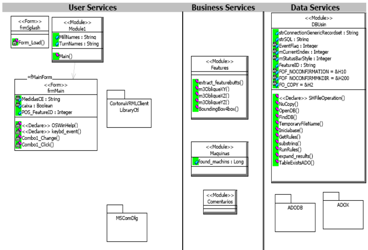
ILUSTRAÇÃO 30 - Diagrama de Classes do UML2, "logical view"
