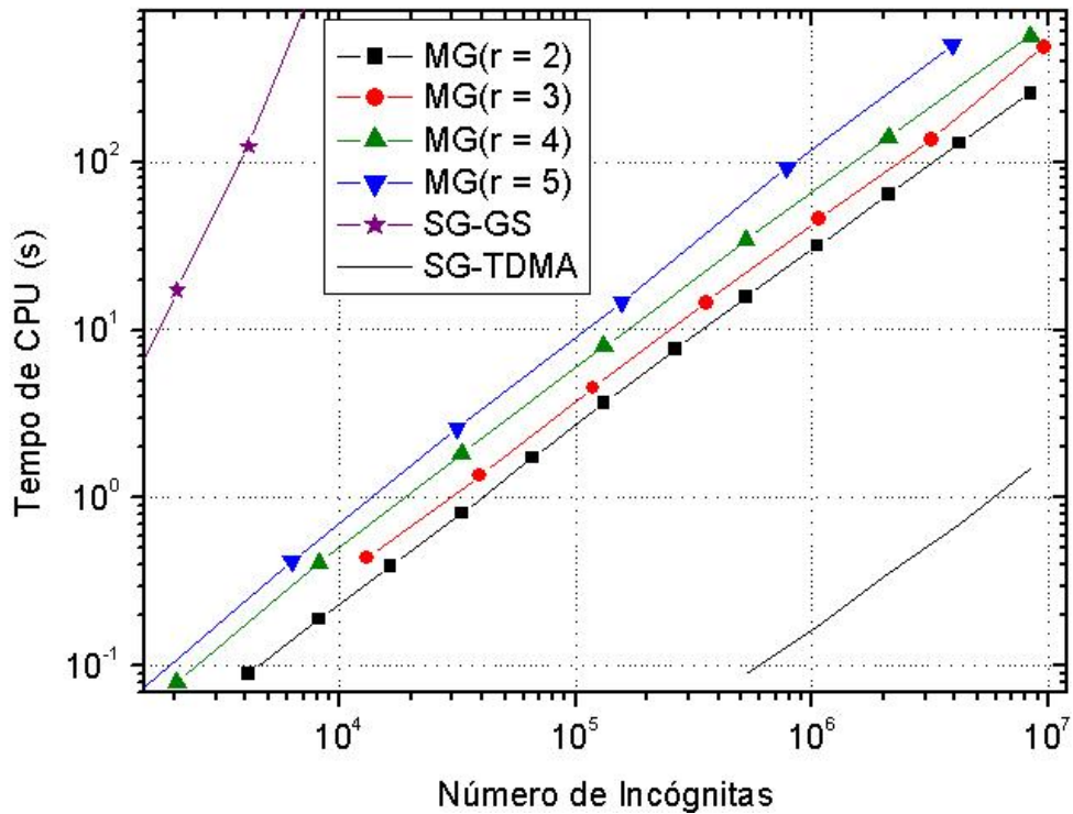
Figura 4.7: Tempo de CPU versus N para a equação de advecção-difusão com o esquema CS, diversos r , com o esquema numérico UDS/CDS e diversos métodos
