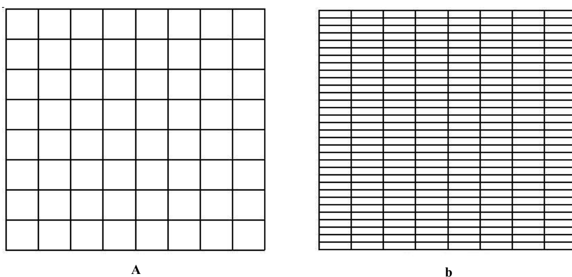
Figura 7.1: Exemplos de malhas: a) isotrópica e b) anisotrópica com RA = 4
