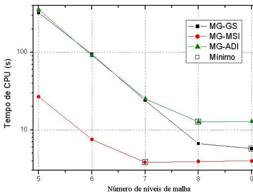
Figura 6.8: Tempo de CPU versus L para a equação de Laplace com o esquema FAS, r = 2 , com o esquema numérico CDS/CDS e diversos solvers
