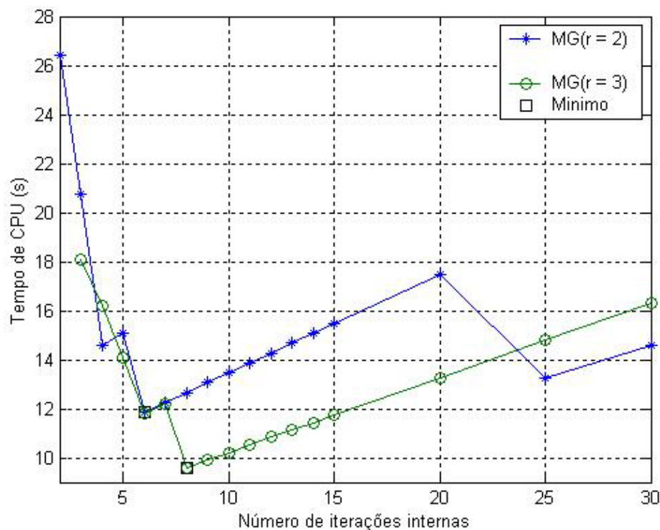
Figura 5.7: Tempo de CPU versus ITI para a equação de Burgers com o esquema FAS, diversos r e com o esquema numérico CDS_CA/CDS
