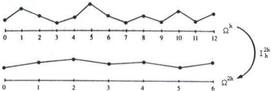
Figura 3.3: Operador de restrição (ponderação completa) da malha fina para a malha grossa (BRIGGS et al., 2000)
