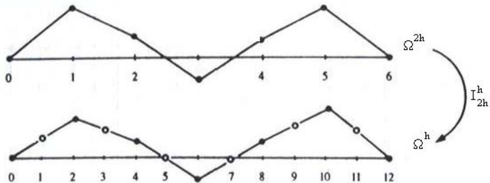
Figura 3.4: Operador de prolongação (interpolação linear) da malha grossa para a malha fina (BRIGGS et al., 2000)
