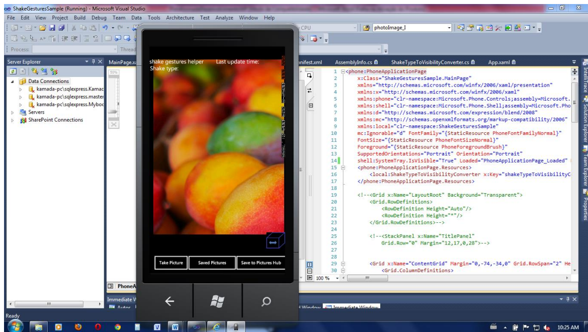
Figura 2. Ferramenta de Desenvolvimento para Mobile - Visual Studio (Kamada, 2012). Catura da imagem Visual Studio 2010 com emulador em modo debugging (Processo de encontrar e reduzir defeitos) e visualização do design e marcação XAML. O Visual Studio, utilizando o IDE, com resposta de edição simultanea com Blend 4
