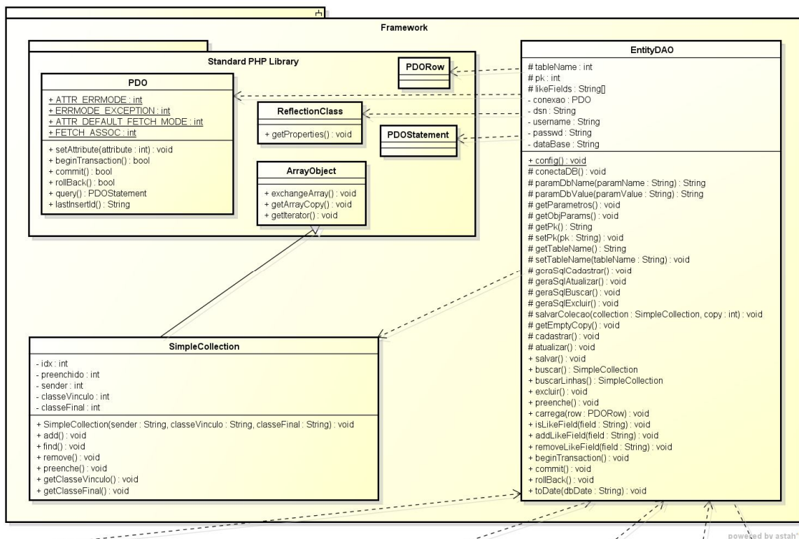
Figura 15 – Diagrama de Classes – Parte 1
