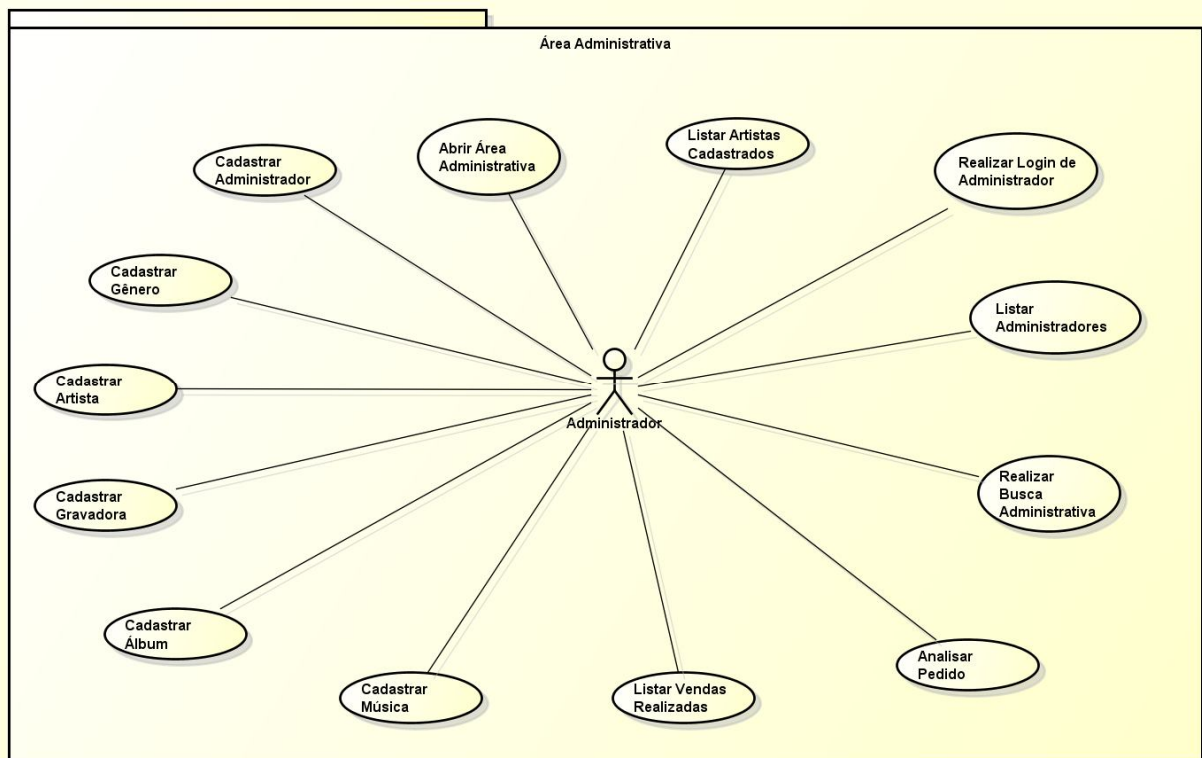
Figura 5 – Diagrama de Casos de Uso - Site
