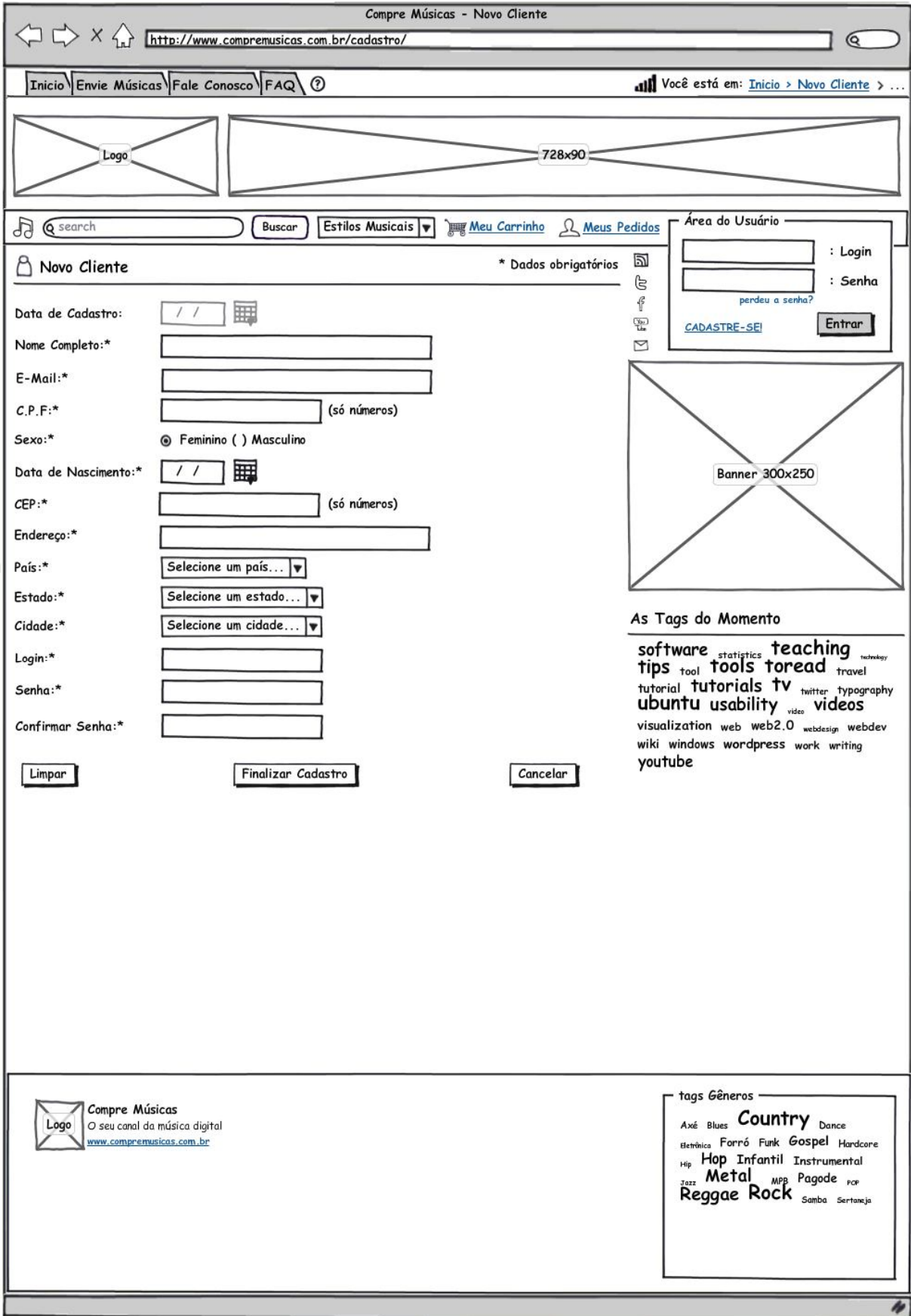
Figura 10 – Projeto Ergonômico - Protótipo – Cadastro de Novo Cliente
