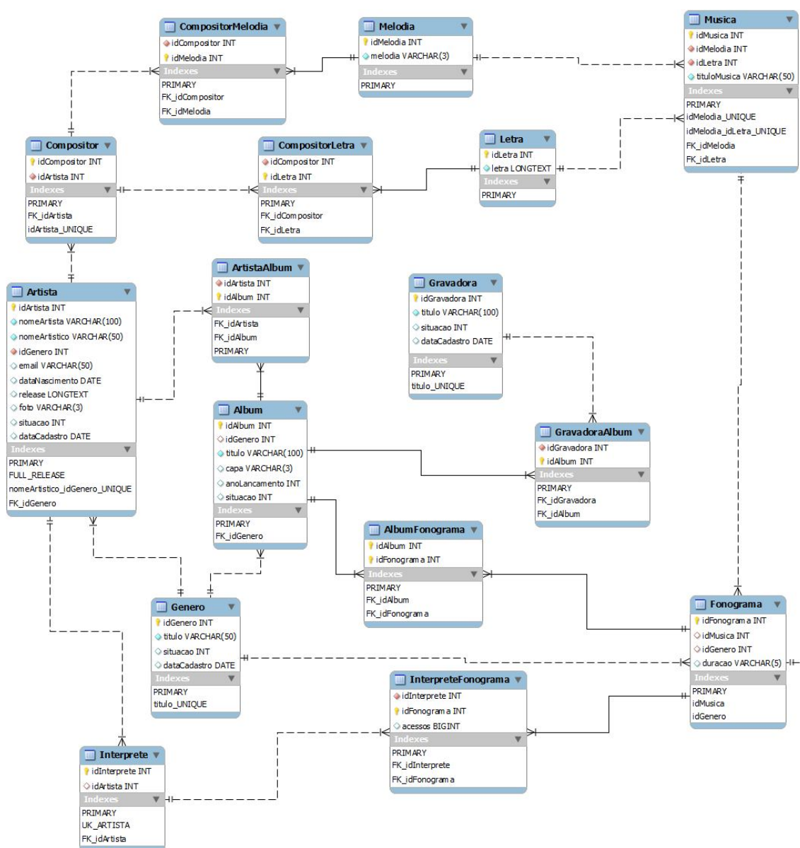
Figura 13 – Projeto do Banco de Dados – Parte 1
