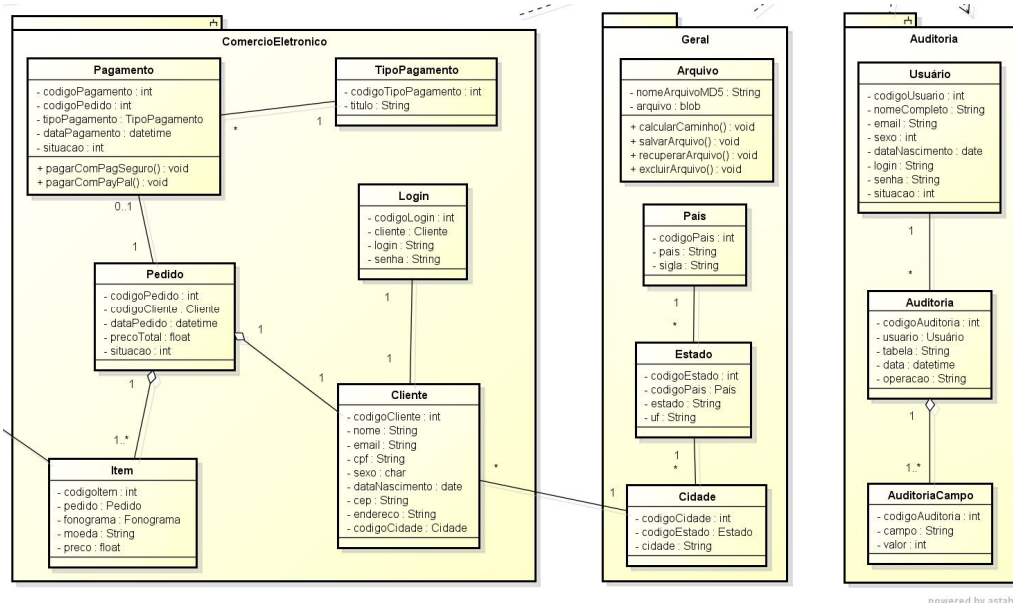
Figura 16 – Diagrama de Classes – Parte 2
