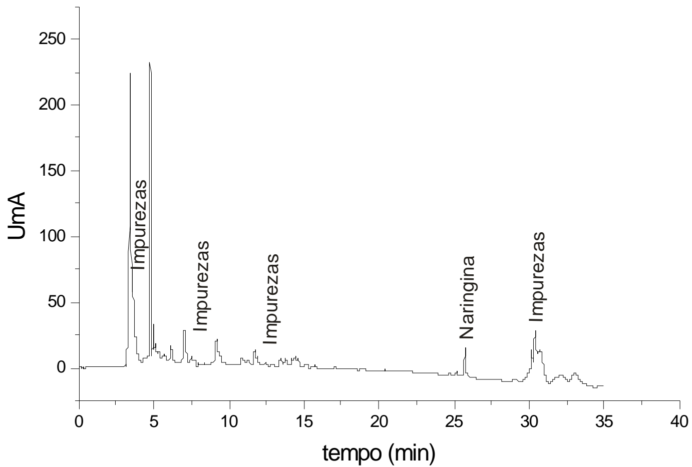
FIGURA 02 - Análise pelo HPLC do extrato aquoso dos frutos da Schinus terebenthifolius Raddi.
