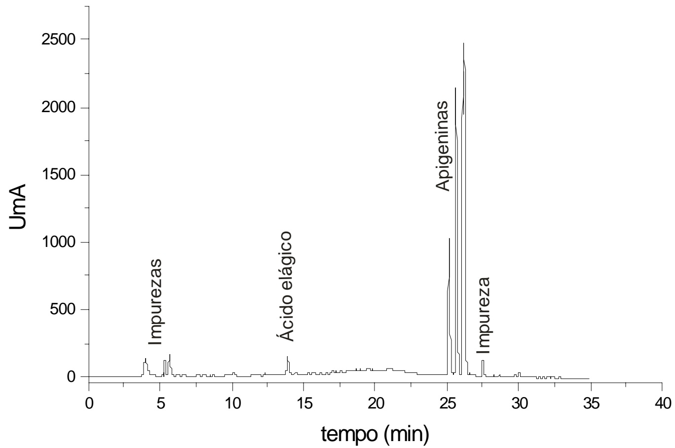
FIGURA 01 - Análise pelo HPLC do extrato alcoólico dos frutos da Schinus terebenthifolius Raddi.
